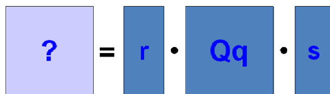
Figura 03: Variante do Método Bi-proporcional Fonte: UFBA, 2008
