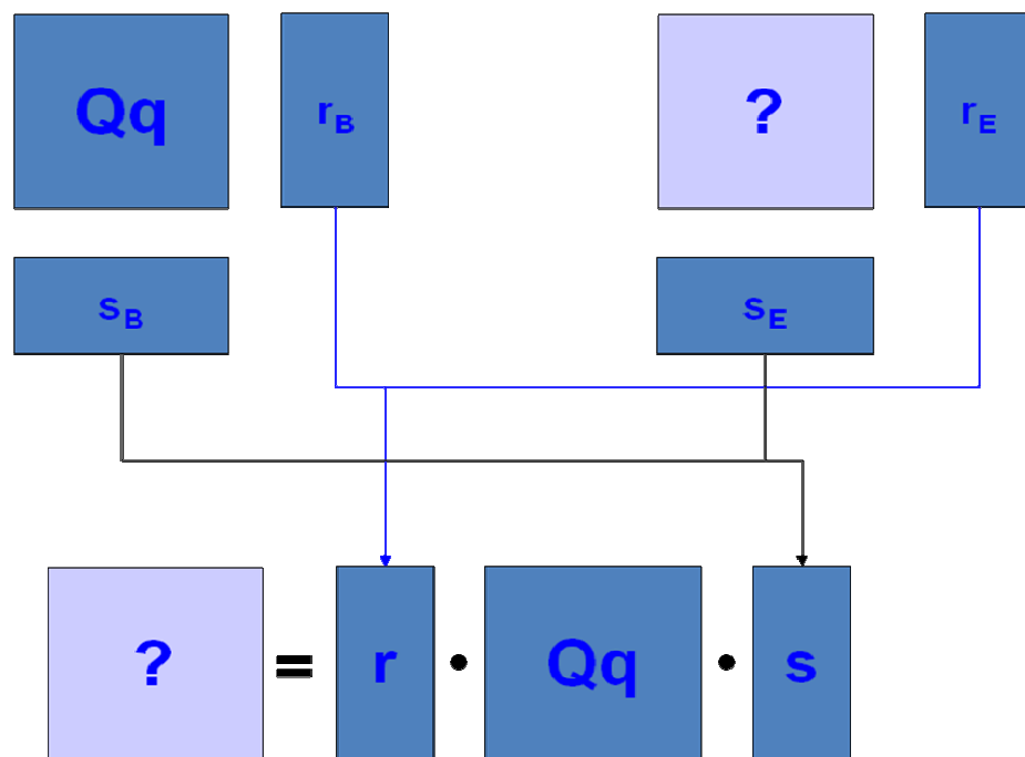
Figura 04: Variante do Método Bi-proporcional Expandido Fonte: UFBA, 2008
