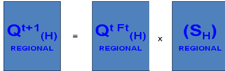
Figura 10: Segundo Passo do Processo de Iteração Fonte: LEITE, 2009
