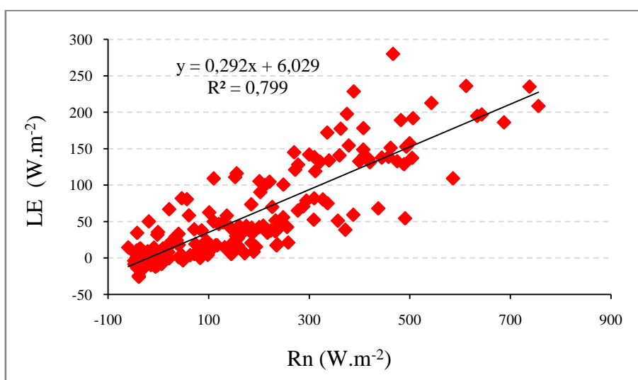
Figura 4.33- Dispersão entre o saldo de radiação e o fluxo de calor latente em área de pastagem.
