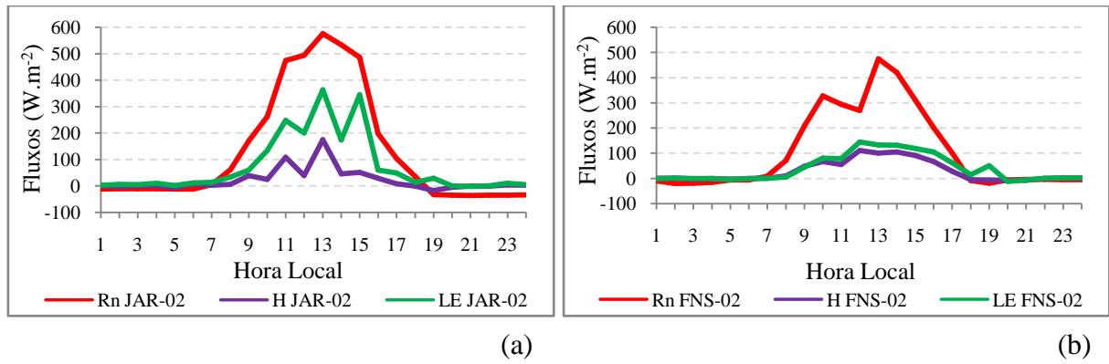
Figura A.10- Dia Juliano 81 (22/mar) em área de Floresta (a) e Pastagem (b).
