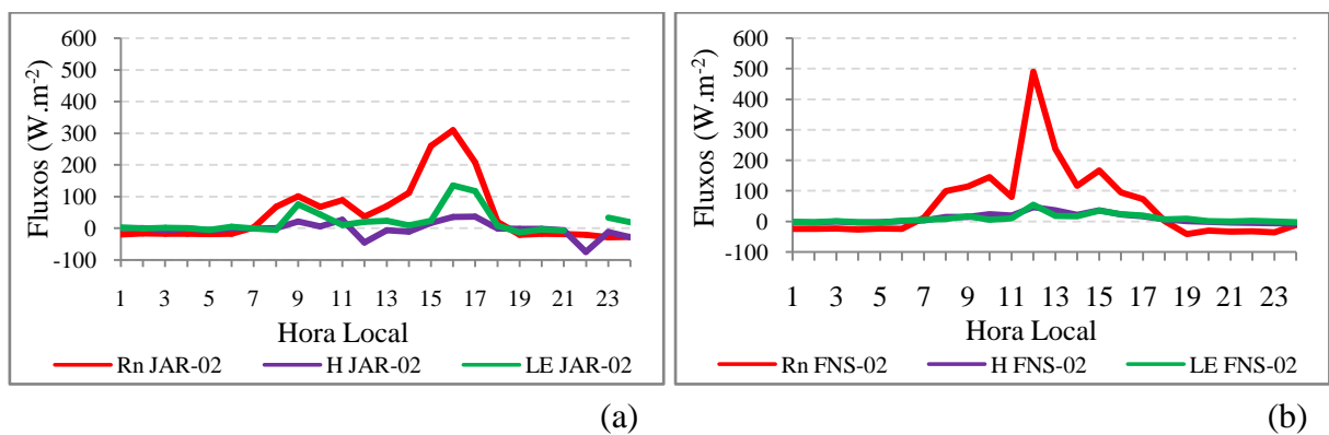
Figura A.11- Dia Juliano 83 (24/mar) em área de Floresta (a) e Pastagem (b).
