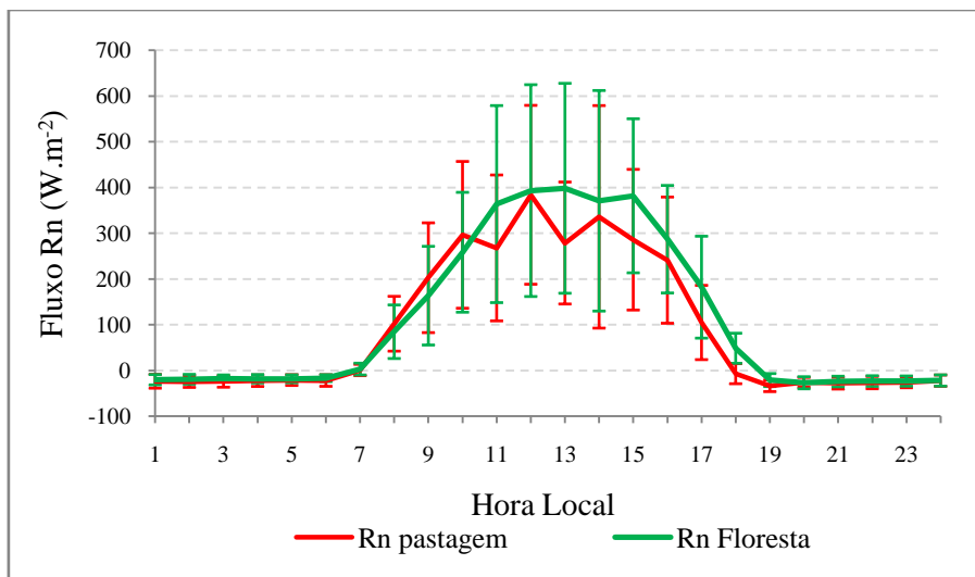
Figura 4.12- Ciclo médio diário do saldo de radiação na floresta (verde) e na pastagem (vermelho). As linhas verticais representam o desvio médio.
