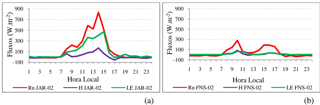
Figura A.12- Dia Juliano 85 (26/mar) em área de Floresta (a) e Pastagem (b).
