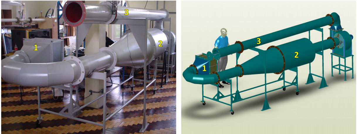
Figura 5.10 — Bancada de ensaios de elementos filtrantes para material particulado (1 primeiro filtro, 2 segundo filtro, 3 pontos de aquisição)
