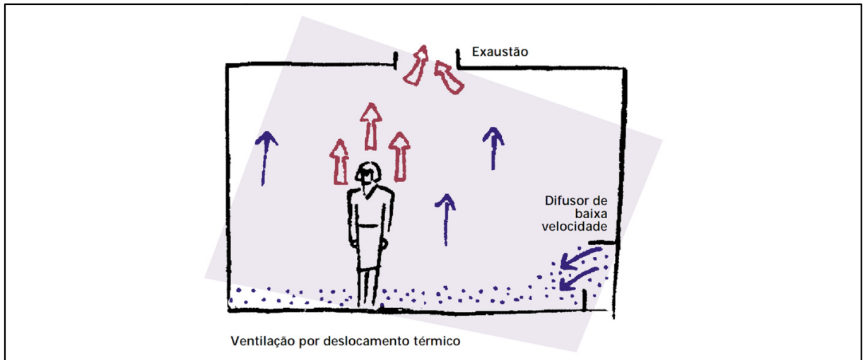
Figura 4.4 — Ventilação por deslocamento térmico [Souza Cruz, 1996b]
