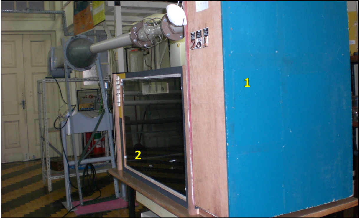
Figura 4.8 — Modelo, vista do plenum (1 plenum, 2 modelo)
