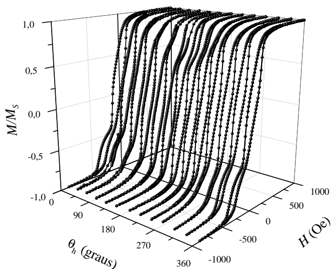
Figura 4.5: Variação angular da amostra \text{Co}_3/\text{IrMn}/\text{Co}_7 .
