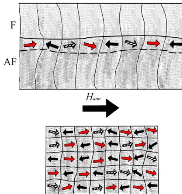
Figura 1.8: Representação esquemática da estrutura de uma bicamada AF/FM policristalina. Acima: corte transversal; abaixo: vista superior. As flechas hachuradas representam os clusters não-compensados.
