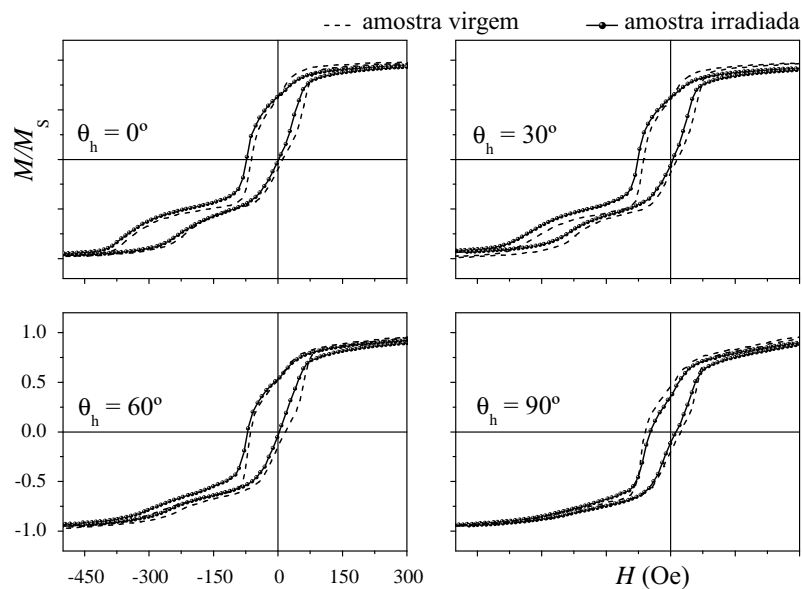
Figura 4.25: Curvas de magnetização da amostra de Co_3/IrMn/Cu_{0.5}/Co_7 virgem (linha tracejada) e irradiada (linha e círculos cheios) com \theta_{irr} = 100^\circ para \theta_h = 0, 30, 60 e 90^\circ .
