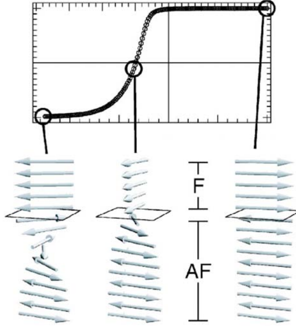
Figura 1.10: Esquema representativo de formação de paredes de domínio no antiferromagneto durante um ciclo de histerese [48] . Note que os autores deste artigo consideram que as camadas AF e FM se acoplam antiferromagneticamente.
