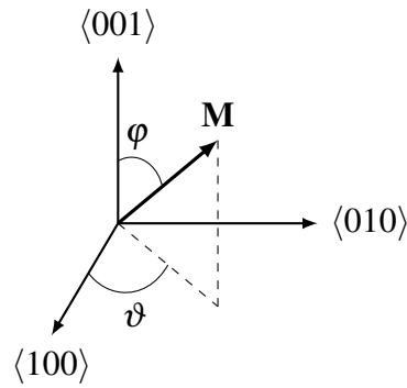
Figura 1.4: Representação da magnetização em relação aos eixos cristalinos de um sistema cúbico.
