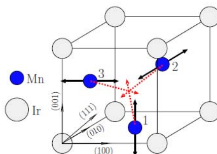
Figura 1.9: Estrutura triangular magneticamente frustrada dos spins dos átomos de Mn. As esferas escuras representam os átomos de Mn enquanto as claras representam os de Ir. As linhas pretas indicam os eixos fáceis locais e as linhas tracejadas em vermelho a direção do spin total no estado fundamental. Figura retirada da referência 37.
