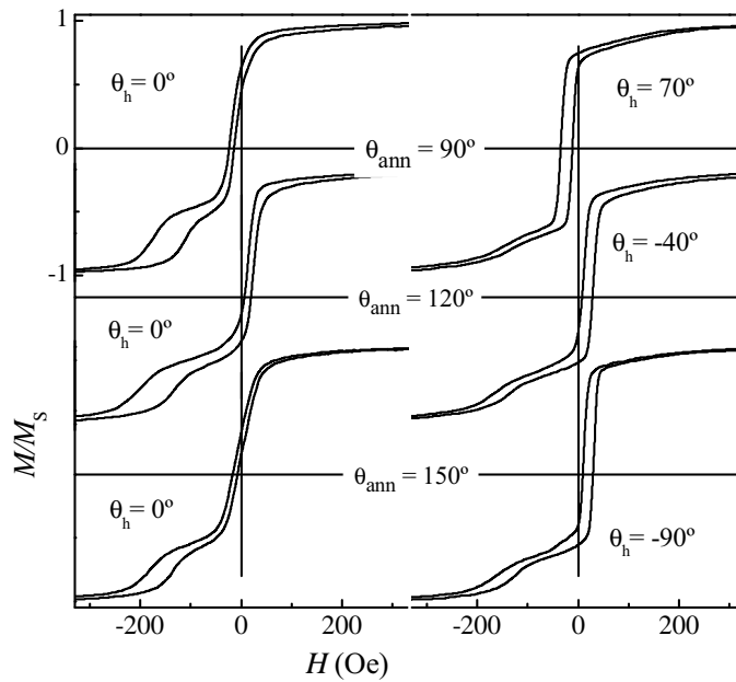
Figura 4.2: Variação do deslocamento da fase bottom-pinned FM em função da direção de H_{\text{ann}} para a amostra de \text{Co}_3/\text{IrMn}/\text{Cu}_{0.75}/\text{Co}_7 tratada termicamente com H_{\text{ann}} = 20 Oe. Esquerda: curvas de histerese medidas com o campo no sentido do EB da configuração FM/AF; direita: o mesmo para o campo de medição no sentido do EB da camada bottom-pinned FM.
