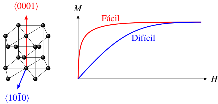
Figura 1.3: Diagrama representando os eixos de fácil (vermelho) e difícil (azul) magnetização para o cobalto h.c.p..
