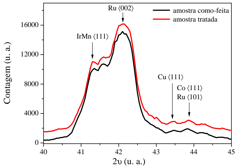
Figura 3.4: Difração de raios-X para a amostra \text{Co}_3/\text{IrMn}/\text{Cu}_{0.75}/\text{Co}_7 . Em preto está representada a amostra no estado como-feita e em vermelho a amostra tratada termicamente. O padrão referente à amostra tratada termicamente foi deslocado verticalmente para melhor visualização.
