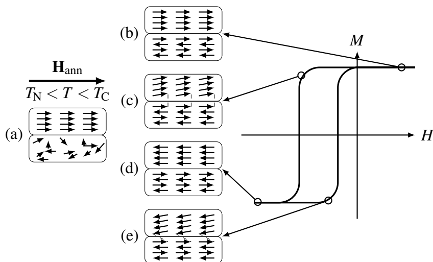
Figura 1.6: Diagrama simples das configurações de spin de uma bicamada AF/FM durante o ciclo de histerese [4] .
