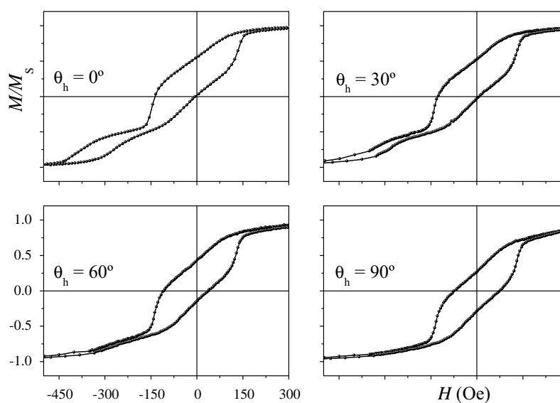
Figura 4.6: Curvas de magnetização da amostra de \text{Co}_3/\text{IrMn}/\text{Co}_7 como-feita para \theta_h = 0, 30, 60 e 90^\circ .
