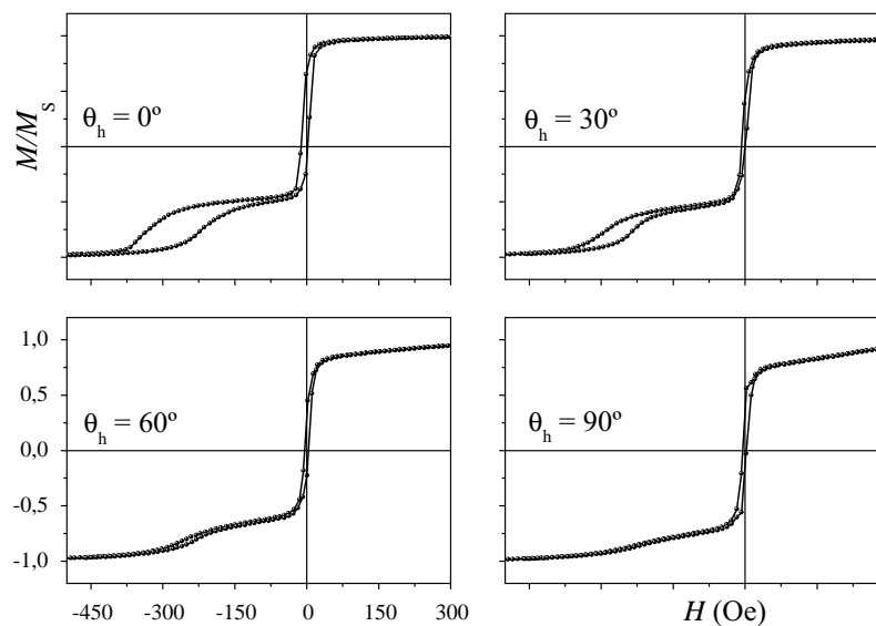
Figura 4.7: Curvas de magnetização da amostra de \text{Co}_3/\text{IrMn}/\text{Cu}_{1.5}/\text{Co}_7 como-feita para \theta_h = 0, 30, 60 e 90^\circ .
