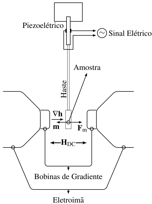
Figura 2.1: Esquema simplificado do AGFM.
