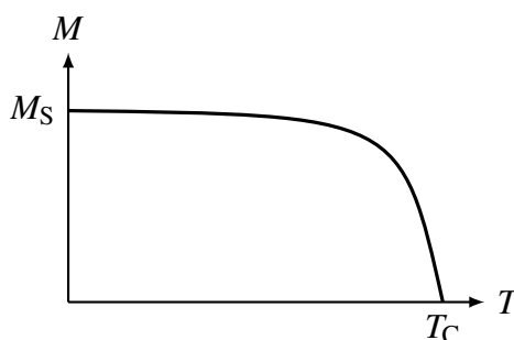
Figura 1.2: Representação ilustrativa da magnetização de um ferromagneto em função da temperatura.
