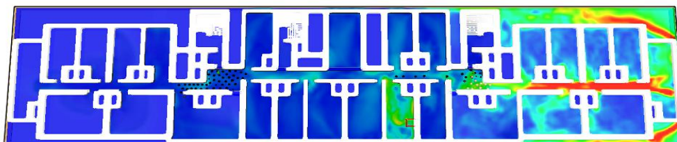
Figura 148 – Velocidade do ar no tempo de 60s (ambiente aberto)
