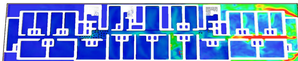
Figura 149 – Velocidade do ar no tempo de 120s (ambiente aberto)
