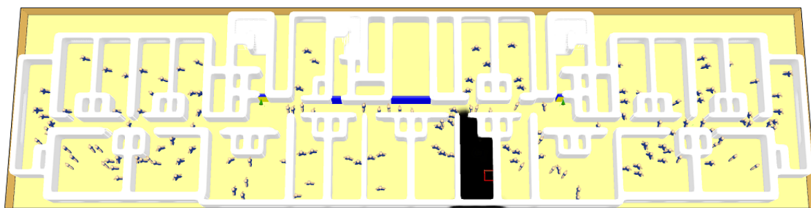
Figura 120 – Imagem da simulação de incêndio e evacuação no tempo de 5s (ambiente fechado).
