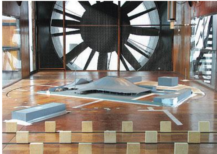
Figura 16 – Modelo reduzido de um projeto e o túnel de vento.
