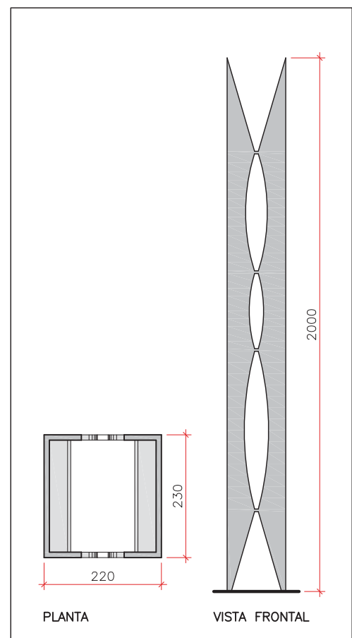
Figura 2.18 - Desenho pombal
