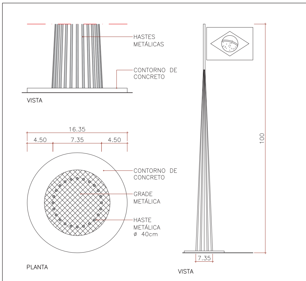
Figura 2.63 - Desenho do Mastro da Bandeira
