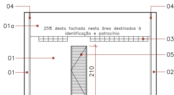
FACHADA POSTERIOR
