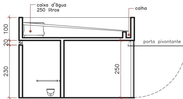
CORTE B-B
