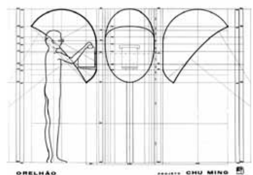
Figura 2.60 - Projeto original do orelhão
