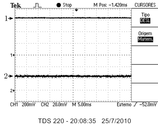
Figura 5.8: Intensidades dos feixes bombeamento e complementar com o OPO estabilizado. No Canal 1 é mostrada a intensidade do feixe bombeamento transmitido pela cavidade, no Canal 2 é mostrada a intensidade do feixe complementar (com \lambda=1064\text{nm} ) separado do bombeio por meio de um filtro como ilustrado na Figura 5.5.
