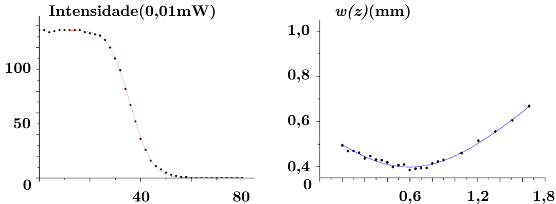
Figura 1.3: (a) Intensidade detectada versus posição da lâmina para um z fixo. (b) Gráfico que relaciona a largura experimental do feixe em função de z . O ajuste desses pontos fornece a cintura do feixe.
