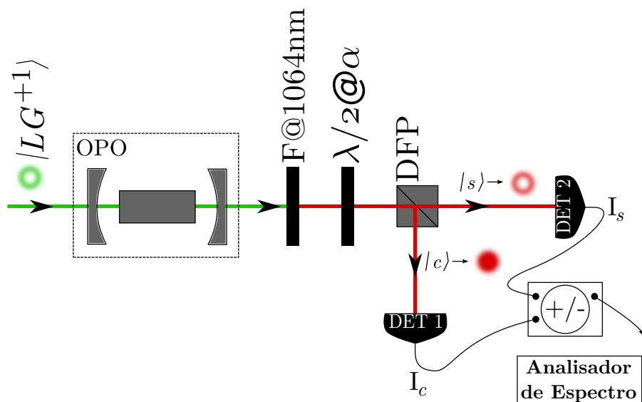
Figura 5.9: Figura Colorida na versão online - Esquema experimental de Detecção Balanceada para a medida de correlações quânticas entre os feixes gêmeos produzidos no OPO bombeado com um modo LG, portador de MAO.
