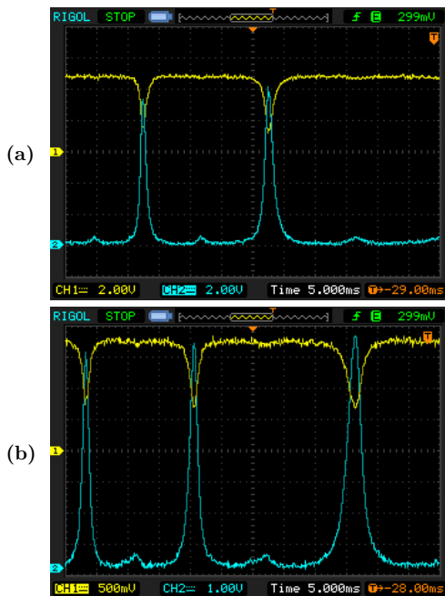
Figura 1.12: Figura Colorida na versão online - Medidas experimentais de I_{t-puro} e I_{t-conv} obtidas no osciloscópio ilustrado na Figura 1.11. (a) resultado obtido com anteparo em 1 e (b) resultado obtido com anteparo em 2.
