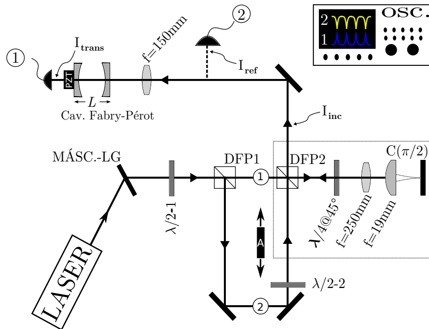
Figura 1.11: Figura Colorida na versão online - Esquema experimental de medida para obtenção da estimativa da fidelidade do conversor de lente única. No canal 2 (amarelo) é mostrada a voltagem associada ao feixe refletido pela cavidade. No canal 1 (azul), intensidade referente ao feixe transmitido.
