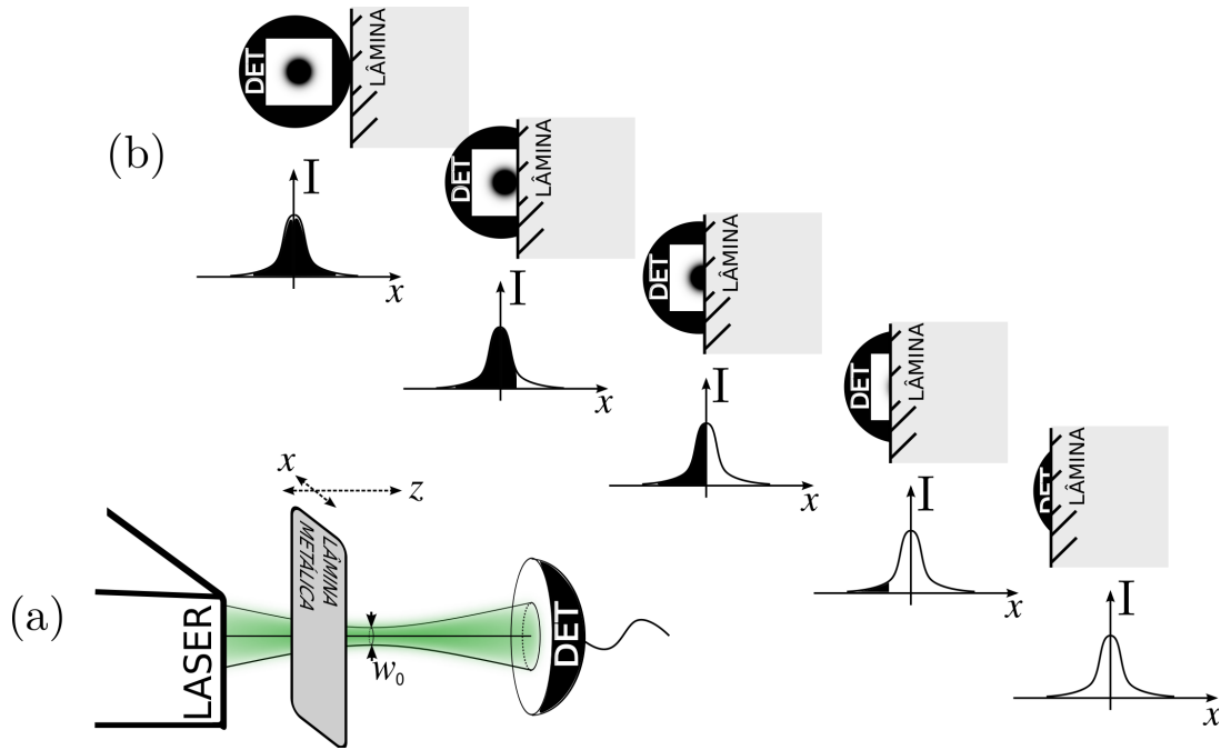
Figura 1.2: (a) Esquema experimental para determinação do parâmetro de Rayleigh. (b) Intensidades medidas no detector para diversas posições da lâmina metálica.
