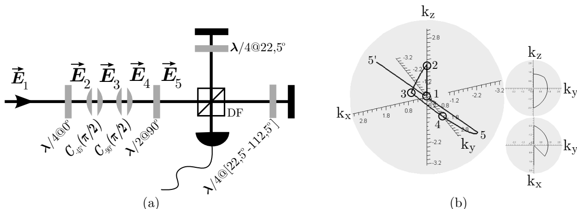
Figura 2.17: (a) Esquema experimental, (b) Gráfico referente ao cálculo analítico de toda evolução do modo maximamente não-separável no experimento ilustrado em (a).
