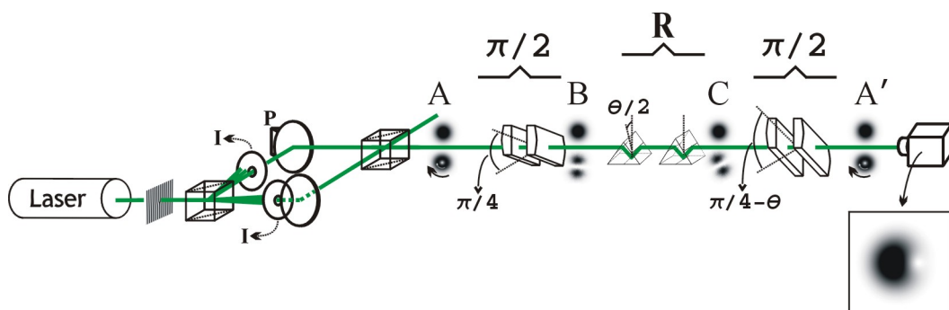
Figura 2.3: Aparato experimental para medição da fase geométrica associada às evoluções cíclicas de modos transversos. No esquema: I- íris e P- PZT.
