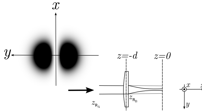
Figura 6.1: Um modo HG_{01} inicialmente isotrópico passa por uma lente cilíndrica e é focalizado em z = 0 . As trajetórias tracejadas entre a lente e o plano z = 0 representam \omega_Y(z) e as contínuas representam \omega_X(z) .
