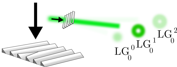
Figura 1.19: Máscara Biased. O modo fundamental de um laser é difratado produzindo um modo superior bem mais intenso que os outros feixes difratados.
