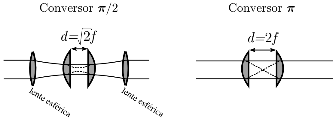
Figura 1.8: Conversores Astigmáticos. No conversor \pi/2 , um par de lentes esféricas é inserido para realizar o casamento de modos.
