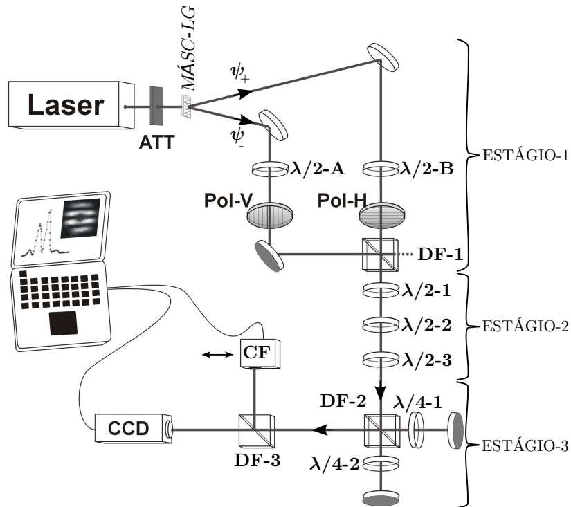
Figura 2.10: Aparato experimental para medida da fase topológica. Estágio 1: a preparação do estado maximamente emaranhado; estágio 2: realização das transformações no estado maximamente emaranhado produzindo a trajetória 1234 na esfera do SO[3] ; estágio 3: transformações 4 \rightarrow 1 e 4' \rightarrow 1 e medida da fase topológica.
