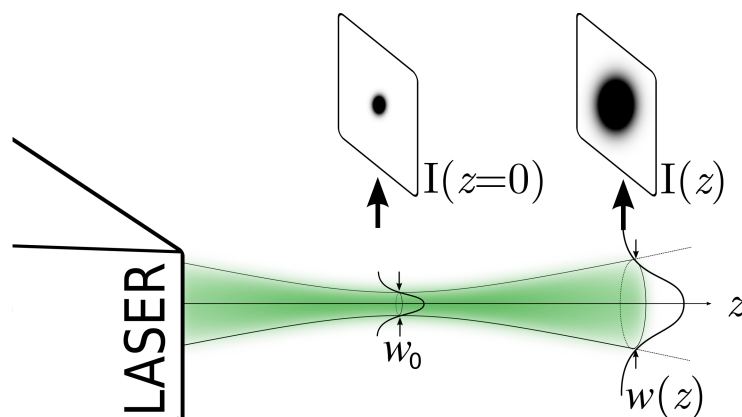
Figura 1.1: Propriedades do feixe gaussino.
