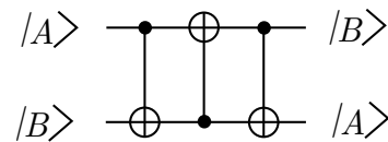
Figura 3.1: Circuito quântico que permuta os estados de dois q-bits.
