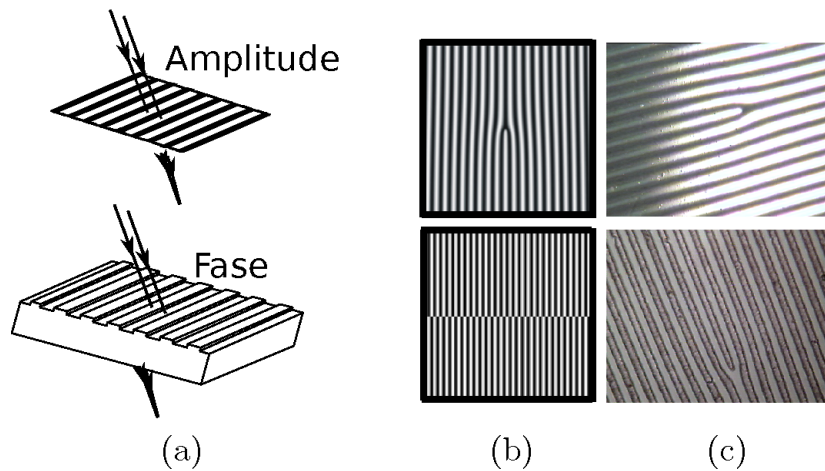
Figura 1.17: (a) Máscaras de amplitude e de fase; (b) acima: perfil de interferência calculado no MATHEMATICA ® entre os modos HG_{00} e LG_0^{+1} e abaixo: entre os modos HG_{00} e HG_{01} ; (c) acima: foto de uma máscara de amplitude e abaixo: foto de fase.
