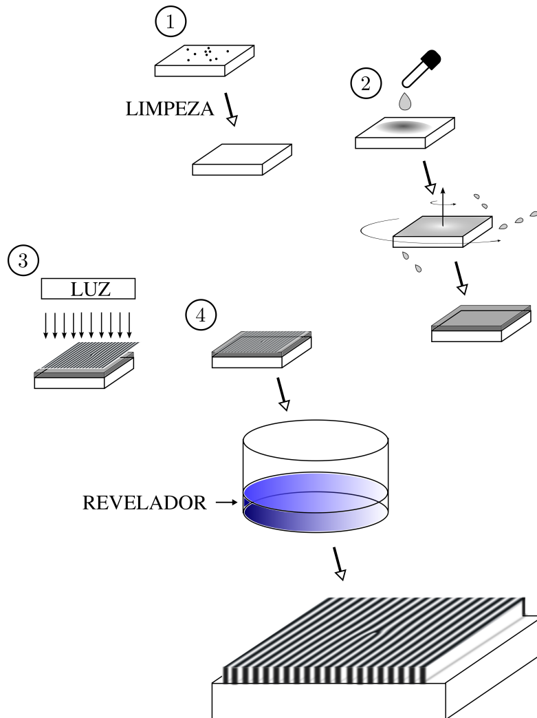
Figura 1.18: Etapas da litografia.
