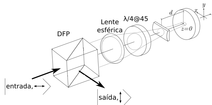
Figura 1.9: Esquema experimental do Conversor de Modos de Lente Única. A distância d determina a fase \phi do conversor.
