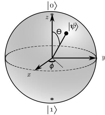
Figura 1.5: A Esfera de Bloch para a representação geométrica de 1 q-bit.
