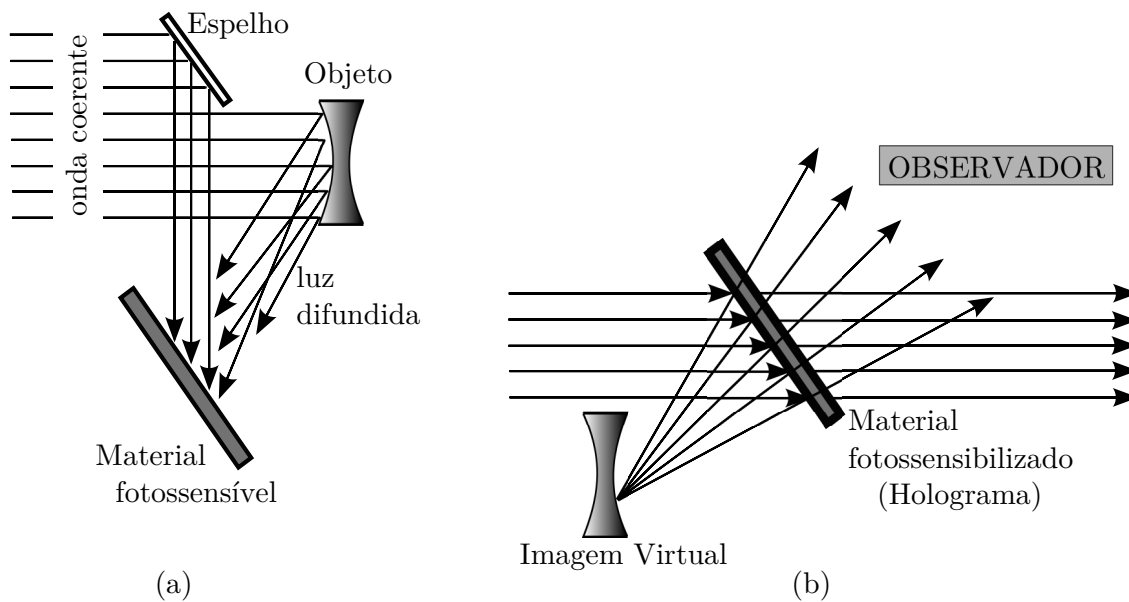
Figura 1.16: (a) A luz difundida por um objeto interfere com uma onda coerente dando origem ao holograma. (b) Um observador localizado na posição indicada vê a imagem do objeto atrás do holograma, iluminado por uma onda coerente, como se ele estivesse presente.
