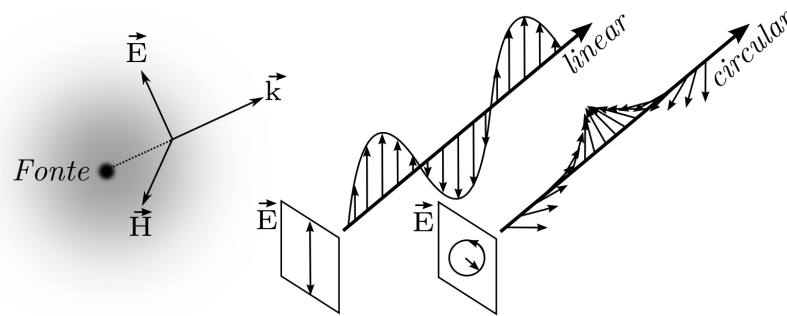
Figura 1: À esquerda, uma fonte pontual de luz e a representação dos campos elétrico e magnético num dado ponto. À direita, a representação da dinâmica dos campos elétricos para ondas linearmente e circularmente polarizadas.
