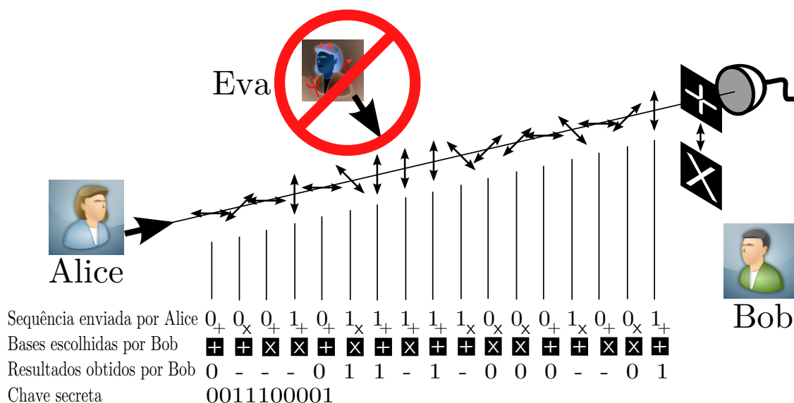
Figura 4.1: Protocolo BB84: Alice envia bits 0s e 1s para Bob codificados como estados de polarizações dos fótons. Bob possui polaróides que podem ser ajustados para medidas nas bases + ou \times . Os resultados de ambos são descartados quando a base escolhida por Bob não coincide com a base de Alice. Por fim, a sequência de bits 0011100001 é compartilhada somente por Alice e Bob e poderá ser utilizada como uma chave para criptografia. As imagens dos bonecos que representam Alice e Bob foram retiradas do programa AMSN.
