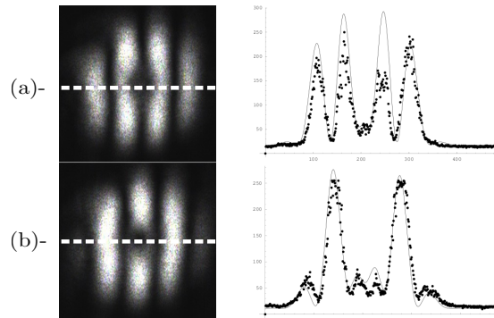
Figura 2.12: Determinação quantitativa da fase \pi . Cada gráfico é obtido a partir da intensidade da imagem ao lado e o ajuste dos pontos é feito com a mesma expressão analítica defasada de \pi .
