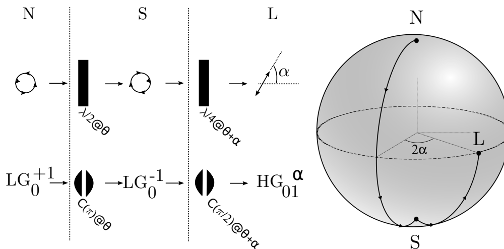
Figura 1.15: Analogia entre as lâminas de onda e os conversores astigmáticos. Acima, é representado um feixe com polarização levógira que passa por duas lâminas e tem sua polarização alterada para destrógira e linear, respectivamente. Estas transformações implementadas pelas lâminas no estado de polarização são representadas geometricamente na esfera através da trajetória que liga os pontos N \rightarrow S \rightarrow L . Abaixo, um modo LG_0^{+1} passa por dois conversores astigmáticos e sofre as transformações indicadas. Estas transformações implementadas pelos conversores também são representadas geometricamente na esfera pela mesma trajetória N \rightarrow S \rightarrow L . \alpha e \theta são ângulos que fornecem a direção de orientação das lâminas e conversores.
