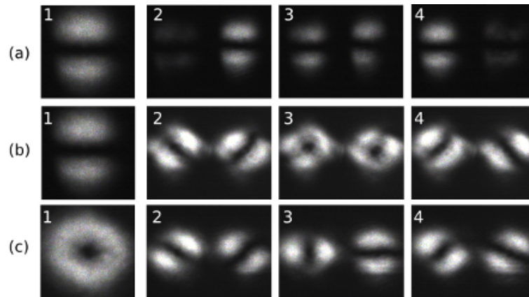
Figura 3.6: Resultados experimentais do SMT. (a) Imagem 1 - modo HG_{01} de entrada no SMT. Imagens 2-4 - modos de saída para diferentes voltagens no PZT e \theta orientado a 0^\circ ; (b) Imagem 1 - modo HG_{01} de entrada no SMT. Imagens 2-4 - modos de saída para diferentes voltagens no PZT e \theta orientado a 45^\circ e (c) Imagem 1 - modo LG de primeira ordem de entrada no SMT. Imagens 2-4 - modos de saída para diferentes voltagens no PZT e \theta orientado a 45^\circ .
