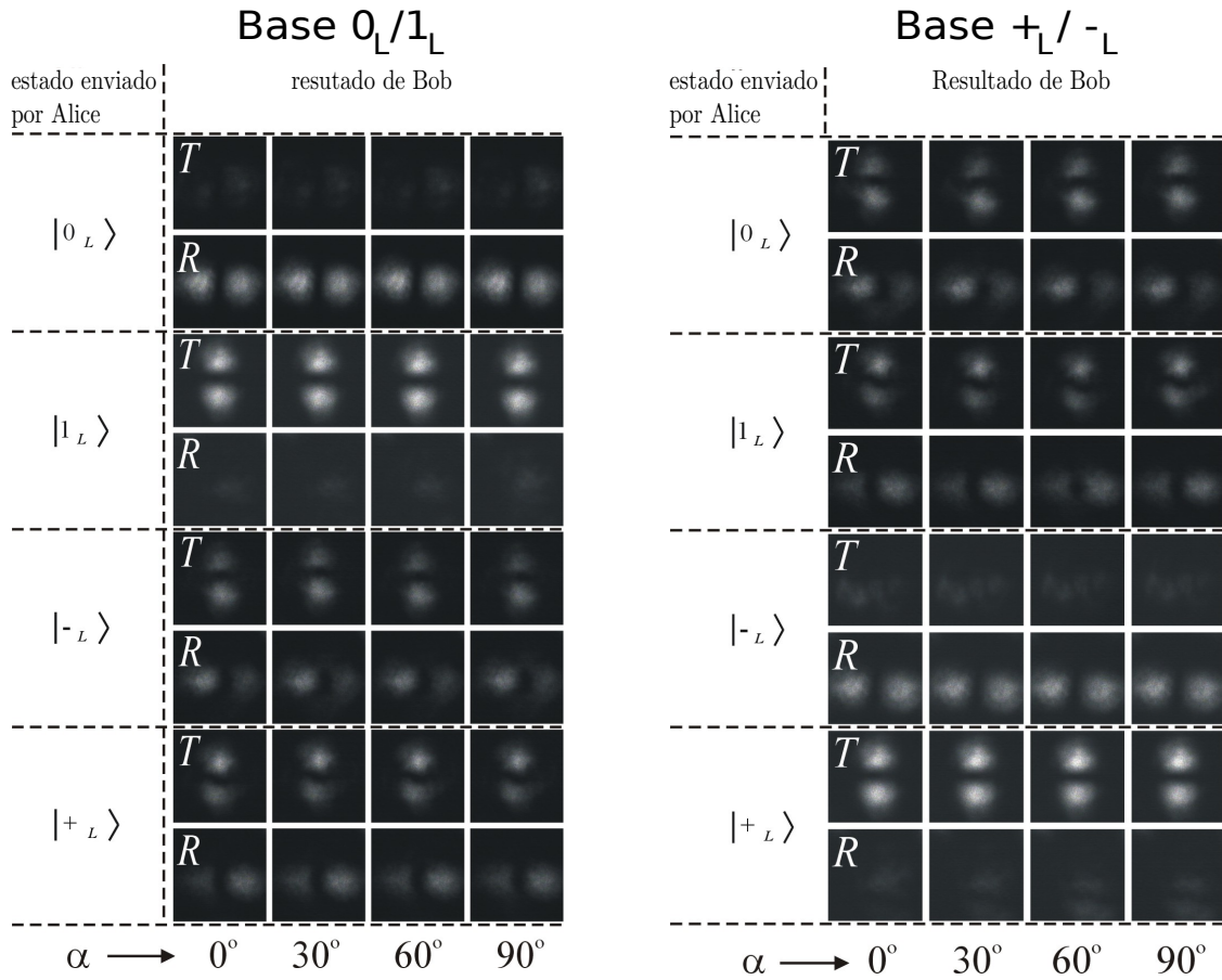
Figura 4.6: Imagens obtidas nas posições dos detectores R e T para várias rotações \alpha entre os referenciais de Alice e Bob. Na esquerda (direita) Bob escolhe a base 0_L/1_L ( +_L/-_L ).
