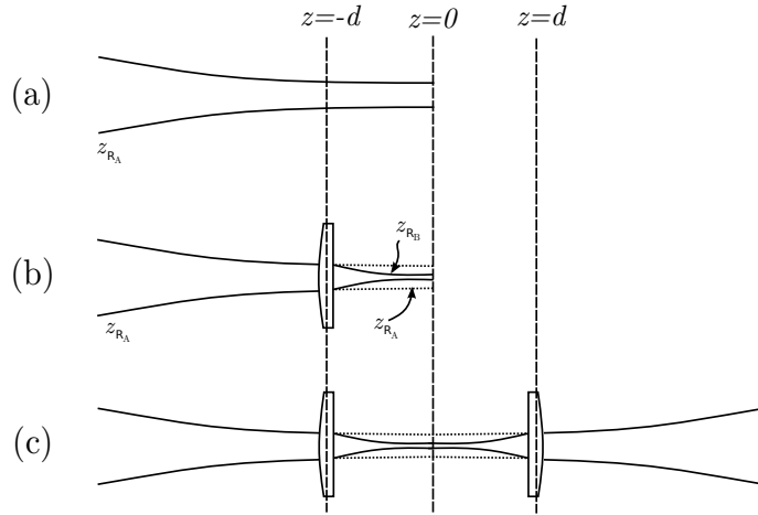
Figura 6.2: O casamento de modos. Em (a) um feixe com divergência z_{RA} tem a cintura posicionada em z = 0 ; em (b) uma lente cilíndrica torna o feixe astigmático; em (c) uma segunda lente corrige o astigmatismo.
