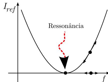
Figura 5.6: Diagrama representando a intensidade do feixe refletido pela cavidade próxima à ressonância em função da frequência. Pode-se determinar se a cavidade está acima ou abaixo da ressonância variando a frequência do laser.
