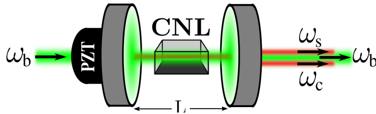
Figura 5.3: Oscilador Paramétrico Ótico.
