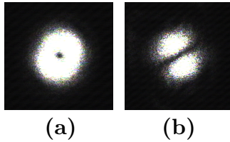
Figura 1.13: Imagem do feixe transmitido pela cavidade Fabry-Pérot em ressonância. Na imagem (a), o anteparo estava posicionado em 1. Na imagem (b), o anteparo estava posicionado em 2
