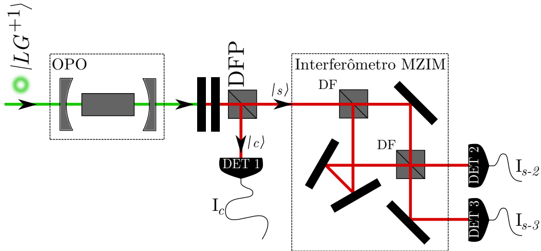
Figura 5.10: Figura Colorida na versão online - Esquema experimental para a medida de correlações quânticas entre as componentes do feixe sinal.
