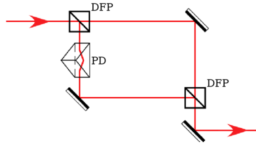
Figura 3.2: Porta CNOT que utiliza a polarização como q-bit de controle e o modo transverso como alvo. Figura retirada da referência original [76].
