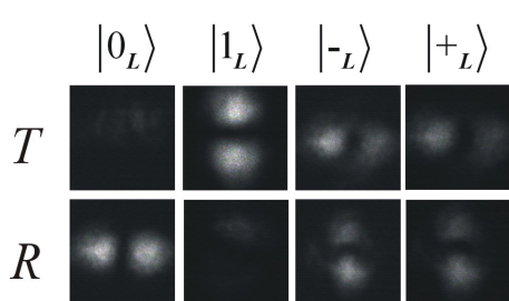
Figura 4.5: Imagens obtidas por uma câmera CCD nas posições dos detectores R e T quando Bob escolheu medir na base 0_L/1_L . Nas duas primeiras colunas, as bases de Alice e Bob coincidem e Bob obtém o bit enviado (somente um detector “acende”). Nas duas últimas colunas, as bases não coincidem e Bob não pode determinar o bit enviado (os dois detectores “acendem”).
