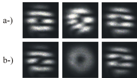
Figura 2.11: Padrões de interferência para (a-) um feixe maximamente não-separável (estado maximamente emaranhado) e (b-) para um feixe separável. Da esquerda para direita as imagens foram obtidas com \lambda/4 -2 orientada a -45^\circ , 0^\circ e 45^\circ , respectivamente.
