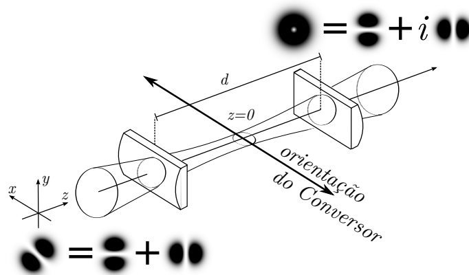
Figura 1.7: O conversor de modos funciona defasando as componentes HG do modo incidente. No exemplo ilustrado, o modo HG_{10}^{+45^\circ} é convertido no modo LG_0^{-1} ao ter suas componentes HG_{10} e HG_{01} defasadas de \pi/2 .
