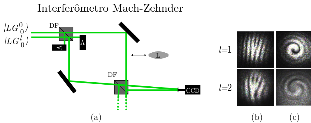
Figura 1.22: (a) Interferômetro de Mach-Zehnder; (b) Padrão de interferência entre os modos fundamental e LG_0^l produzidos por uma máscara LG. (c) Padrão de interferência entre uma onda divergente (produzida com a inserção de uma lente esférica L) com os modos LG_0^l produzidos por uma máscara LG.
