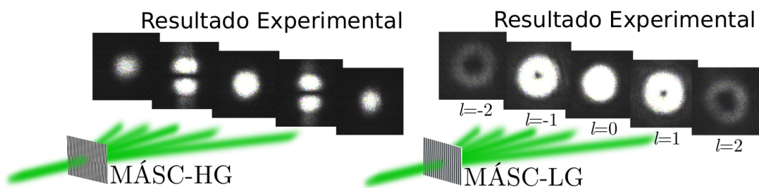
Figura 1.20: Funcionamento das máscaras. A máscara HG produz o modo HG_{01} ao difratar o modo fundamental proveniente de um laser. A máscara LG produz modos LG_0^l com diferentes l .
