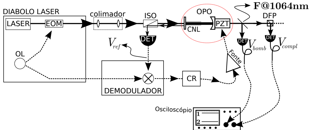
Figura 5.5: Esquema experimental de estabilização da cavidade. Nesse esquema, as linhas contínuas indicam o caminho óptico dos feixes e as linhas tracejadas indicam os cabos utilizados para transmissão das tensões elétricas.
