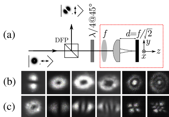
Figura 1.10: (a) O Conversor \pi/2 de lente única. A conversão do modo LG_0^{+1} no modo HG_{10}^{+45^\circ} é ilustrada neste esquema experimental. (b) Fotografia do perfil de intensidade dos modos experimentais. (c) Fotografia do perfil de intensidade dos modos experimentais convertidos no aparato.
