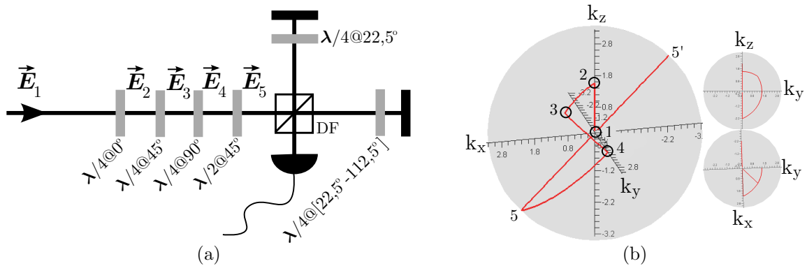
Figura 2.15: (a) Esquema experimental, (b) Gráfico referente ao cálculo analítico de toda evolução do modo maximamente não-separável no experimento ilustrado em (a).
