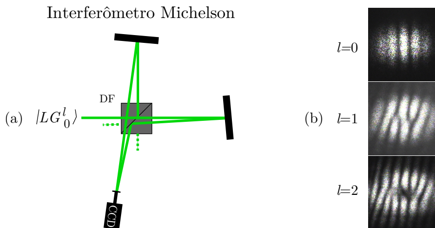
Figura 1.21: (a) Interferômetro de Michelson; (b) Padrão de interferência dos modos produzidos por uma máscara LG. O número de bifurcações em uma franja de interferência determina a carga topológica l do modo.
