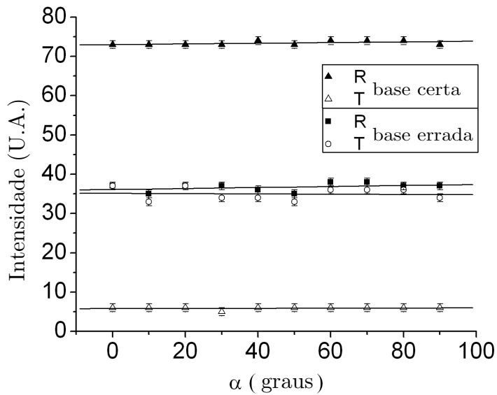
Figura 4.7: Intensidade medida com um medidor de potência como função do ângulo \alpha do laboratório de Alice. As curvas contínuas mostram os ajustes lineares dos pontos experimentais.
