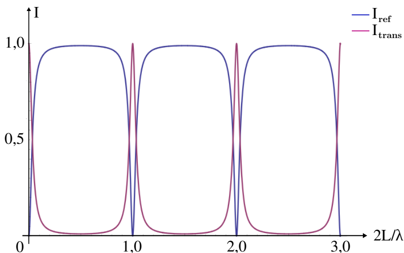
Figura 5.4: Figura Colorida na versão online - Cálculo das intensidades dos feixes transmitido e refletido por uma cavidade Fabry-Pérot.
