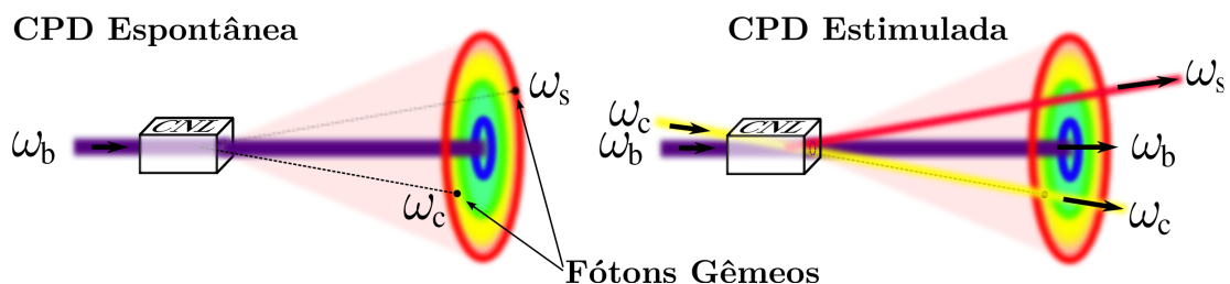
Figura 5.1: Figura colorida na versão online - Conversão Paramétrica Descendente.
