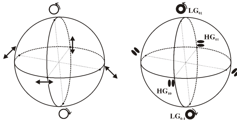
Figura 1.14: (a) Esfera de Poincaré e (b) Esfera dos modos .
