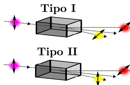
Figura 5.2: Figura colorida na versão online - Conversão paramétrica descendente. (a) no casamento de fase tipo I, um fóton do feixe de bombeamento é aniquilado para a criação de dois fótons paralelamente polarizados; (b) no casamento de fase tipo II, os dois fótons criados têm polarizações ortogonais entre si.
