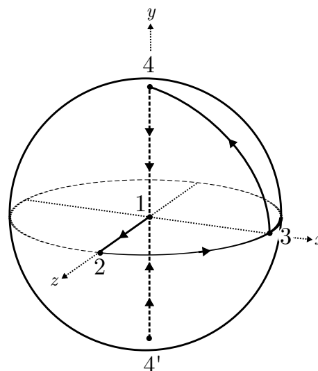
Figura 2.9: Evolução cíclica na esfera do SO[3]. Os pontos 4 e 4' são diametralmente opostos e representam o mesmo modo spin-órbita. As transformações cíclicas são representadas pelas trajetórias 1234 e 1234'.
