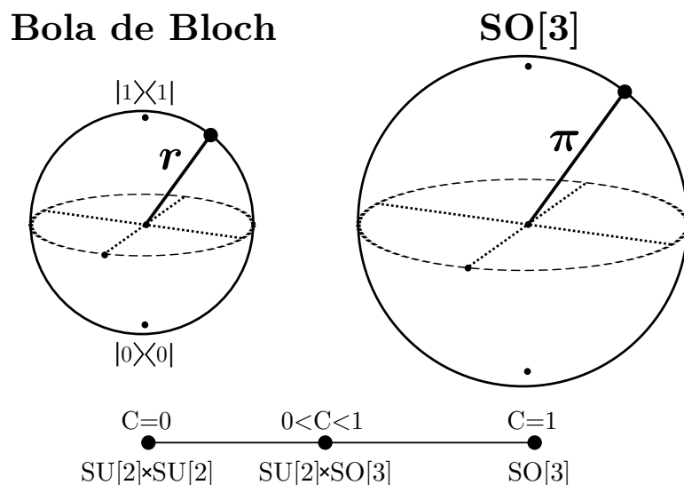
Figura 2.6: Representação geométrica de um estado de dois q -bits por meio das bolas de Bloch e do grupo SO[3] . Essa representação proposta em [64] depende do emaranhamento do sistema. Nos casos limites onde a concordância quântica vale C=0 e C=1 , as representações se reduzem a duas esferas de Bloch ( SU[2] \times SU[2] ) e uma única bola do SO[3] , respectivamente. O caso geral com 0 < C < 1 é o ilustrado na figura.
