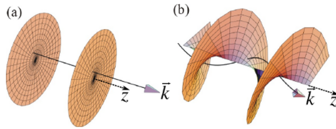
Figura 2: (a) Frente de onda plana de um feixe sem momento angular orbital se propagando ao longo da direção z com vetor de onda \vec{k} sempre paralelo à z ; (b) Frente de onda helicoidal de um feixe com momento angular orbital se propagando ao longo da direção z e com \vec{k} espiralando em torno de z .
