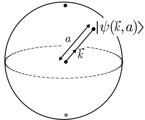
Figura 2.8: Um estado maximamente emaranhado mapeado na esfera do SO[3] em função dos parâmetros \vec{k} e a .
