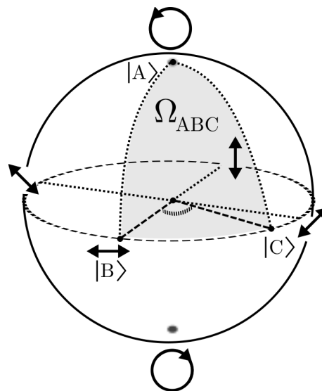
Figura 2.1: A fase de Pancharatnam na esfera de Poincaré. Um feixe que sofre uma transformação cíclica no estado de polarização adquire uma fase geométrica igual a metade do ângulo sólido determinado pela trajetória de evolução.
