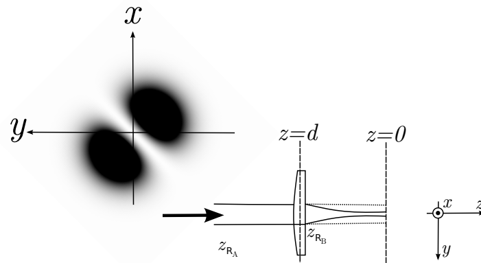
Figura 6.3: Um modo HG_{01}^{+45^\circ} inicialmente isotrópico passa por uma lente cilíndrica e é focalizado em z = 0 . As trajetórias tracejadas entre a lente e o plano z = 0 representam \omega_Y(z) e as contínuas representam \omega_X(z) .
