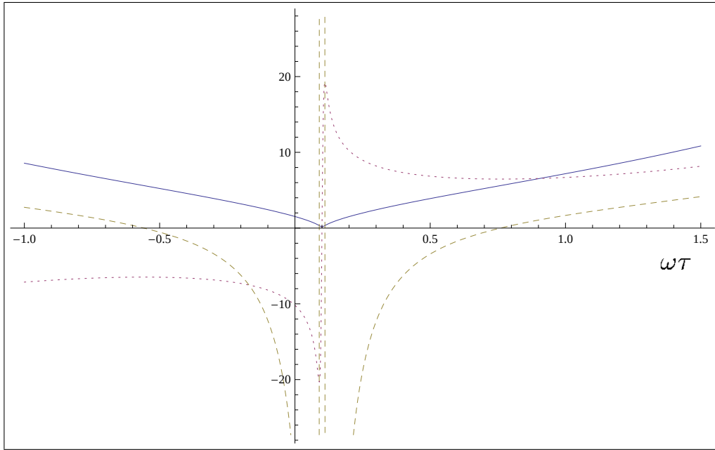
Figura 3.5: O valor esperado do fator de escala (sólido), primeira derivada (pontilhado), segunda derivada (tracejado); \sigma = 1 e \beta = 10 .
