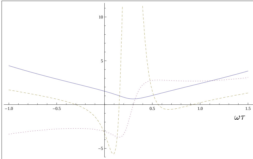
Figura 3.11: O valor esperado do fator de escala (sólido), primeira derivada (pontilhado), segunda derivada (tracejado); \sigma = 2 e \beta = 3 .
