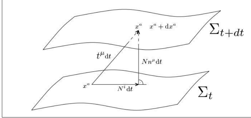
Figura 2.1: Diagrama do espaço-tempo ilustrando a decomposição 3+1 e o significado geométrico da função lapso e do vetor deslocamento.
