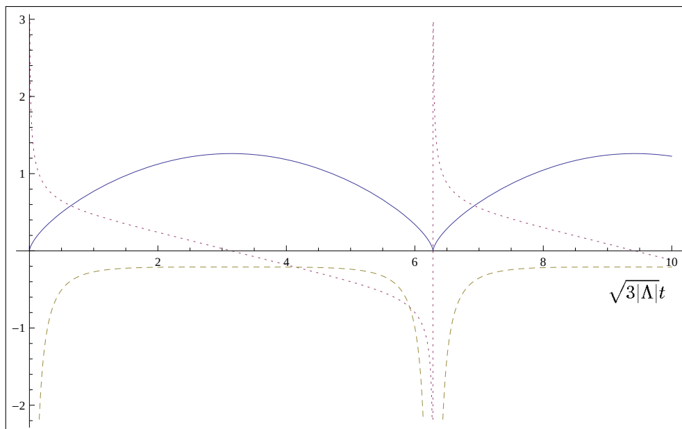
Figura 3.1: O fator de escala (sólido), primeira derivada (pontilhado), segunda derivada (tracejado); \Lambda < 0 .
