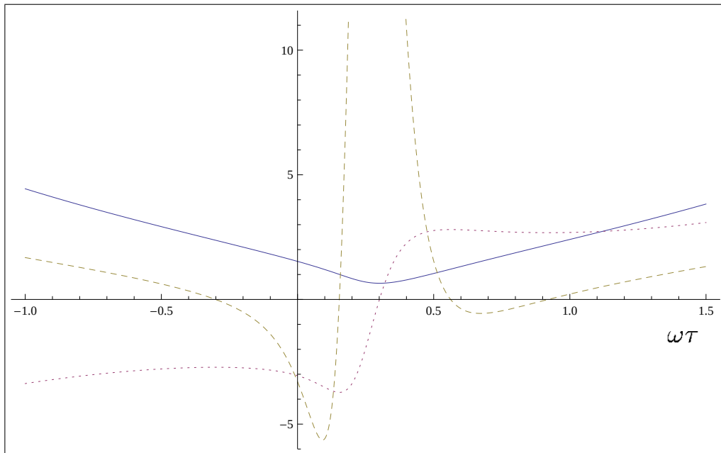
Figura 3.6: O valor esperado do fator de escala (sólido), primeira derivada (pontilhado), segunda derivada (tracejado); \sigma = 2 e \beta = 3 .
