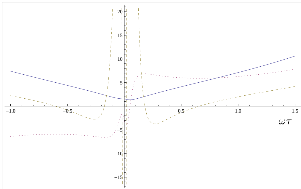
Figura 3.12: O valor esperado do fator de escala (sólido), primeira derivada (pontilhado), segunda derivada (tracejado); \sigma = 20 e \beta = 3 .
