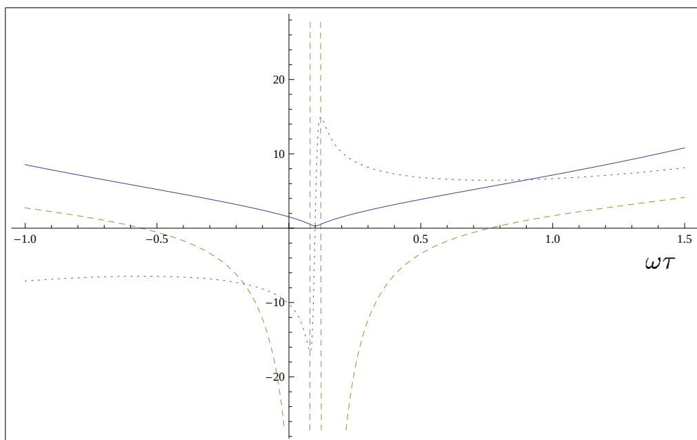
Figura 3.14: O valor esperado do fator de escala (sólido), primeira derivada (pontilhado), segunda derivada (tracejado); \sigma = 2 e \beta = 10 .
