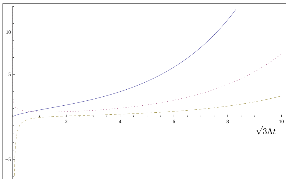
Figura 3.2: O fator de escala (sólido), primeira derivada (pontilhado), segunda derivada (tracejado); \Lambda > 0 .
