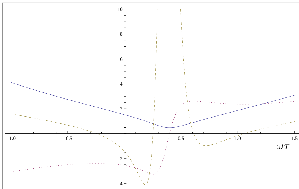
Figura 3.3: O valor esperado do fator de escala (sólido), primeira derivada (pontilhado), segunda derivada (tracejado); \sigma = 1 e \beta = 2, 5 .
