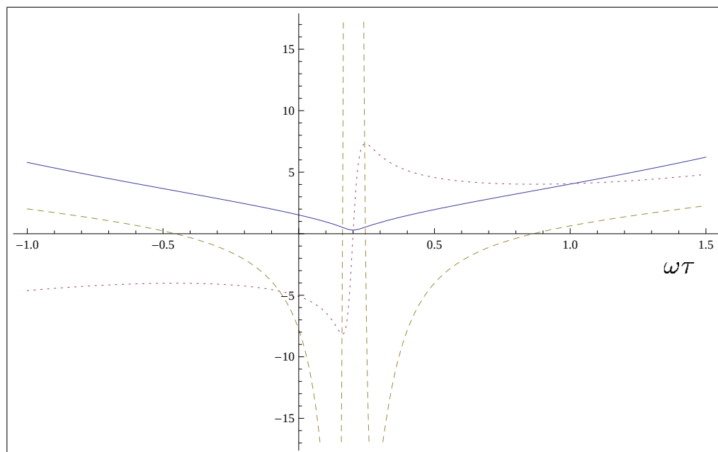
Figura 3.4: O valor esperado do fator de escala (sólido), primeira derivada (pontilhado), segunda derivada (tracejado); \sigma = 1 e \beta = 5 .
