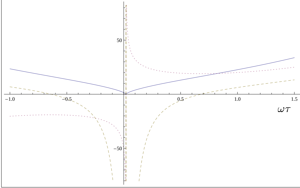
Figura 3.15: O valor esperado do fator de escala (sólido), primeira derivada (pontilhado), segunda derivada (tracejado); \sigma = 2 e \beta = 50 .
