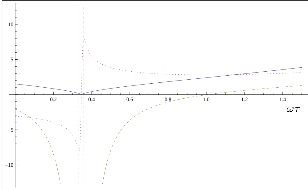
Figura 3.10: O valor esperado do fator de escala (sólido), primeira derivada (pontilhado), segunda derivada (tracejado); \sigma = 0.1 e \beta = 3 .
