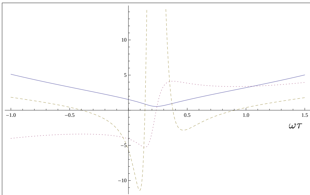
Figura 3.13: O valor esperado do fator de escala (sólido), primeira derivada (pontilhado), segunda derivada (tracejado); \sigma = 2 e \beta = 4 .
