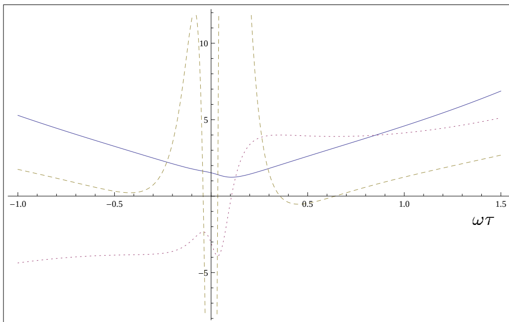
Figura 3.7: O valor esperado do fator de escala (sólido), primeira derivada (pontilhado), segunda derivada (tracejado); \sigma = 10 e \beta = 3 .
