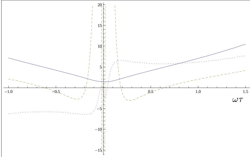
Figura 3.9: O valor esperado do fator de escala (sólido), primeira derivada (pontilhado), segunda derivada (tracejado); \sigma = 20 e \beta = 1 .
