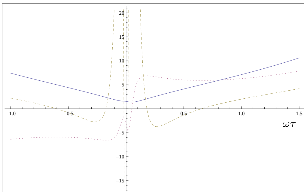
Figura 3.8: O valor esperado do fator de escala (sólido), primeira derivada (pontilhado), segunda derivada (tracejado); \sigma = 20 e \beta = 3 .
