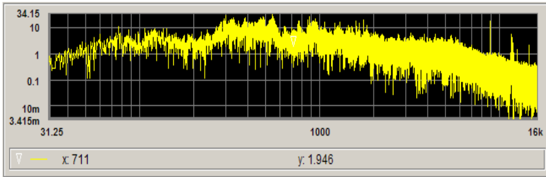
Figura A2. 10 - Transformada Rápida de Fourier (FFT) CONCEITO da Região 5 (Pressão Sonora (Pa) x Frequência (Hz)). (Fonte: Imagem obtida do programa Agilent VEE).
