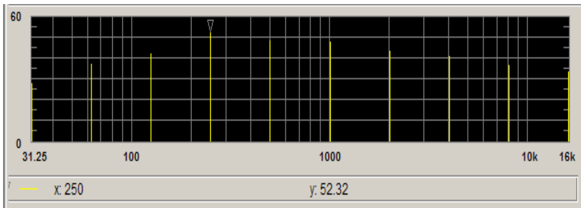
Figura A2. 17 - Transformada Rápida de Fourier (FFT) CONCEITO da Região 7 (Nível de Pressão Sonora (dB) x Freqüência (Hz)) Espectro Discreto em bandas de oitava de freqüência. (Fonte: Imagem obtida do programa Agilent VEE)
