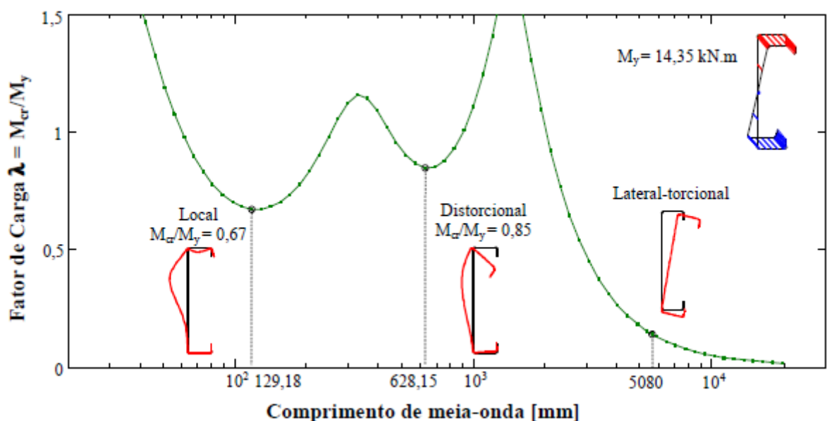
Figura 2.10: Curva de flambagem elástica obtida no CUFSM (Fonte: Grigoletti, 2008)
