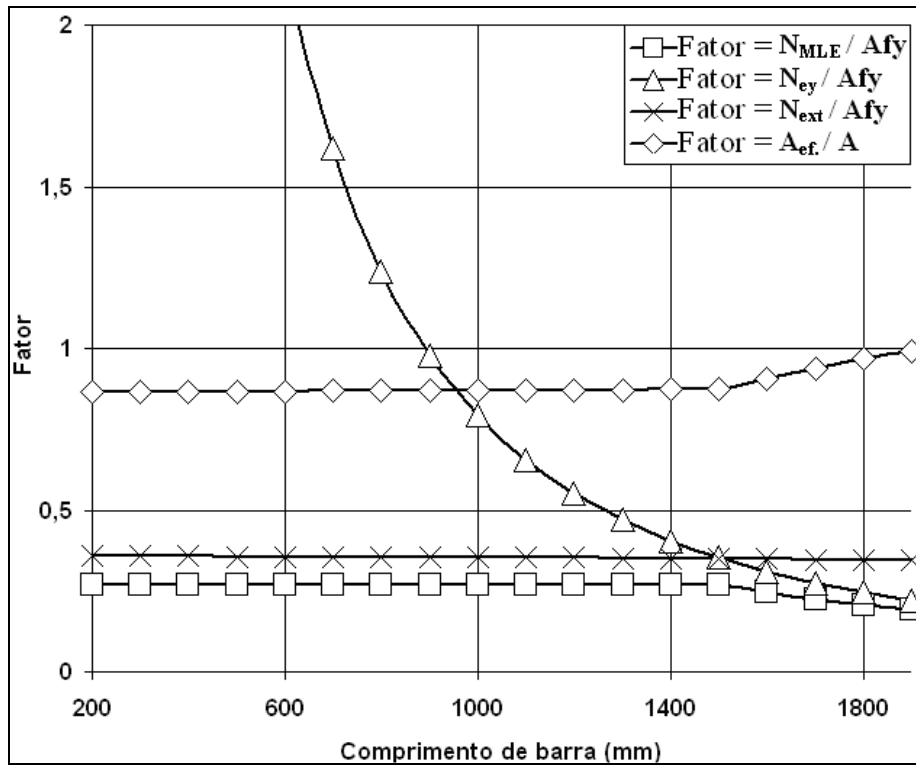
Figura 5.4: Gráfico fator x comprimento de barra correspondentes aos cálculos da cantoneira de seção 60x2,38mm via MLE
