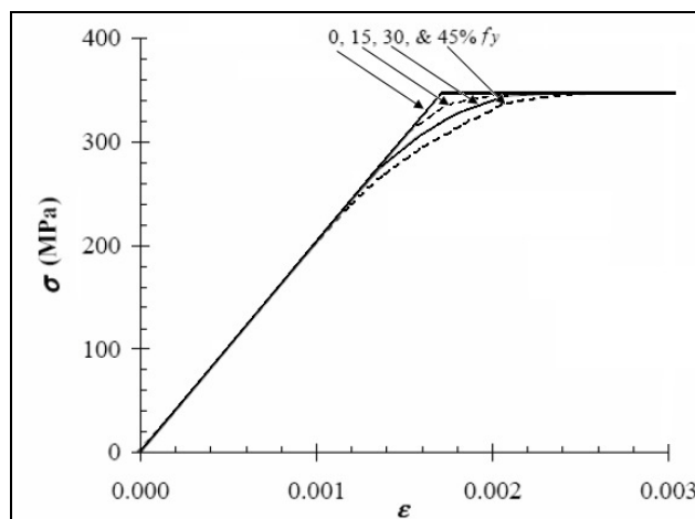
Figura 3.4: Influência da tensão residual de flexão no diagrama tensão-deformação (Fonte: modificada de Schafer, 1997)
