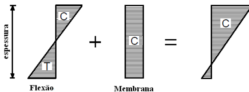
Figura 3.2: Tensões residuais em perfis de aço formados a frio: de flexão e de membrana (Fonte: adaptado de Schafer e Peköz, 1998)
