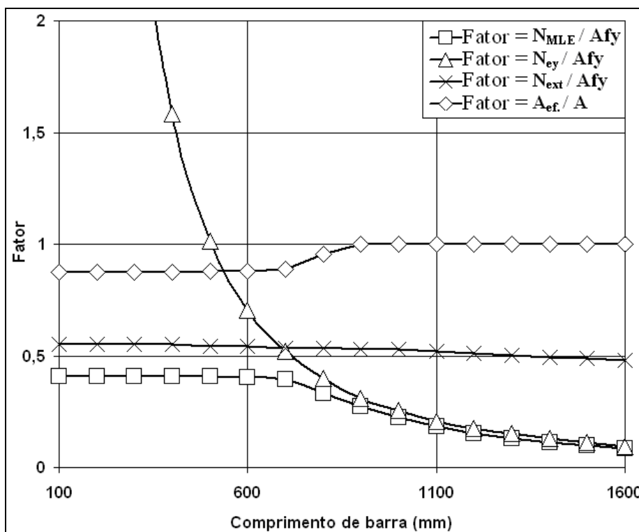
Figura 5.5: Gráfico fator x comprimento de barra correspondentes aos cálculos da cantoneira de seção 27x1,06mm via MLE
