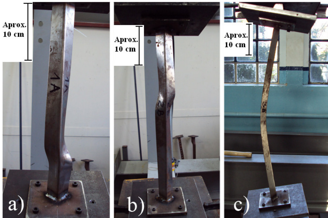
Figura 5.3: Modo de colapso para cada comprimento de barra ensaiada
