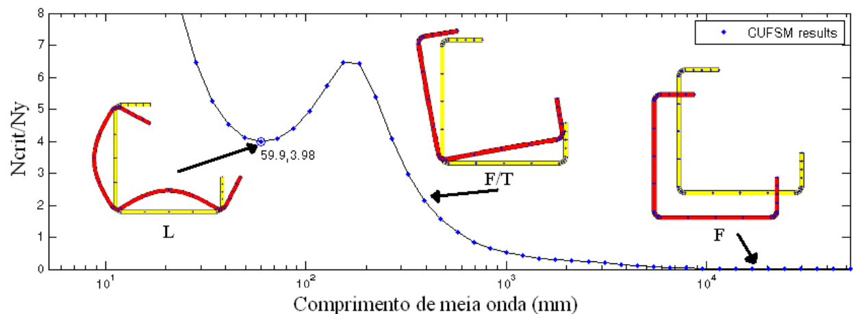
Figura 4.3: Análise de estabilidade elástica via programa CUFSM da cantoneira enrijecida (MFF convencional)
