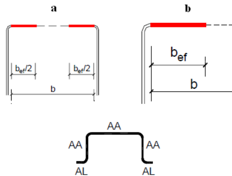
Figura 2.8: Largura efetiva juntamente com a ilustração dos tipos de elementos componentes de perfis formados a frio segundo a norma brasileira: a) Elementos AA e b) Elementos AL (Fonte: NBR 14762 revisão 6, junho 2009)
