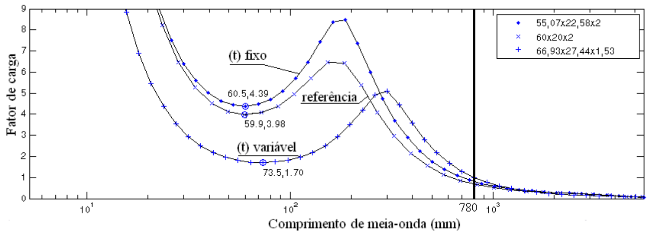
Figura 5.22: Gráfico gerado pelo programa CUFSM para o Problema A (força de colapso fixa com minimização da área da seção transversal) partindo do perfil 60x20x2mm.
