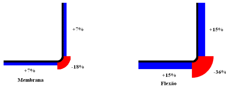
Figura 3.3: Tensões residuais médias medidas em uma cantoneira simples, porcentagem de f_y (Fonte: adaptado de Young, 2005)
