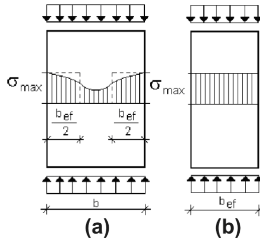
Figura 2.4: (a) Placa real sob compressão uniforme sofrendo flambagem local. A largura é b e a distribuição de tensões é não-uniforme. (b) Placa efetiva, com largura efetiva b_{ef} e distribuição de tensões uniforme
