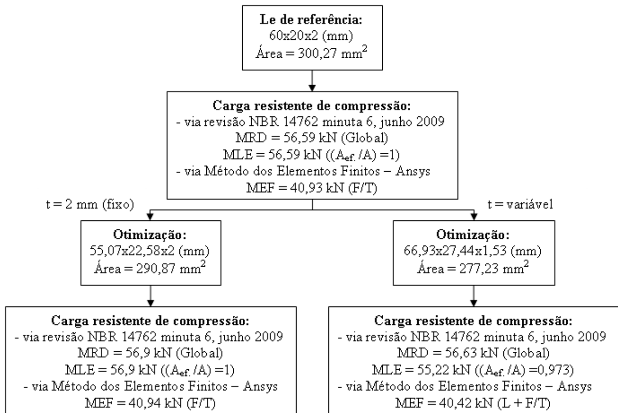
Figura 5.26: Passos da otimização e verificação da seção de referência L_e 60x20x2 mm para minimização da área da seção transversal (Problema A)
