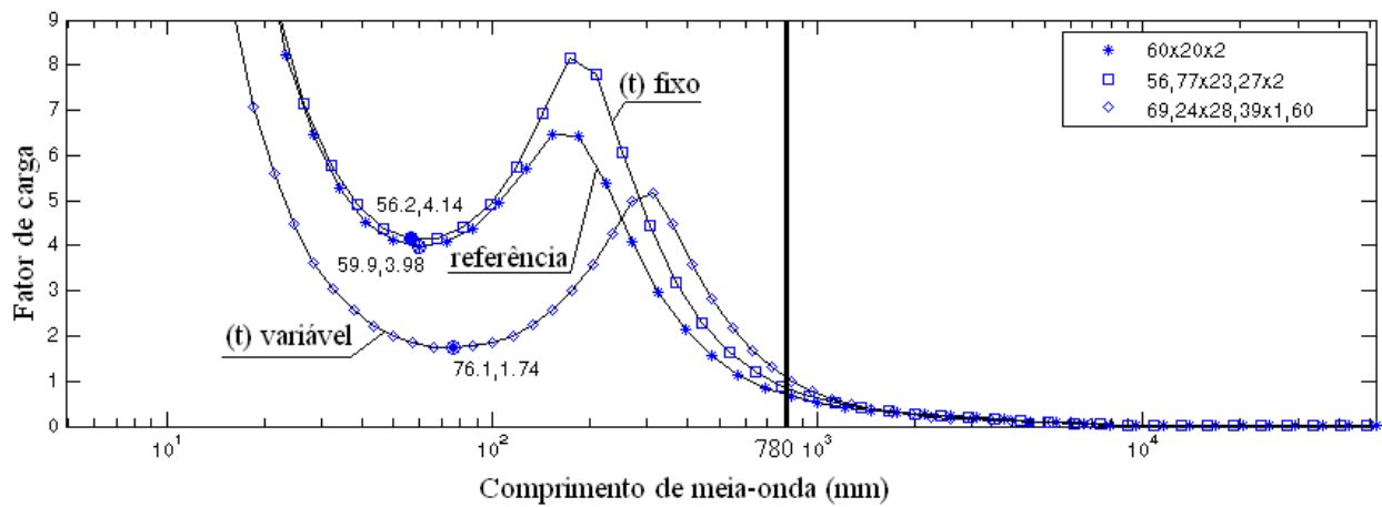
Figura 5.23: Gráfico gerado pelo programa CUFSM para o Problema B (área da seção transversal fixa com maximização da força de colapso) partindo do perfil 60x20x2mm.
