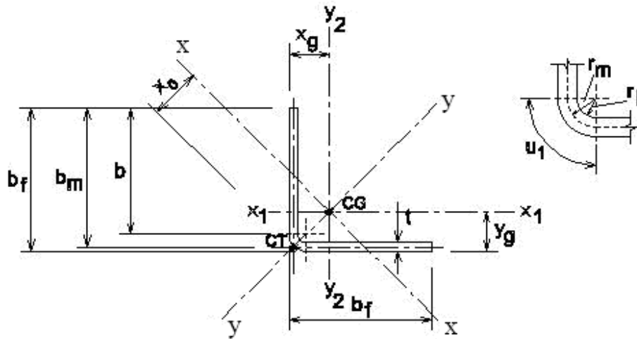
Figura 5.1: Seção transversal da cantoneira simples
