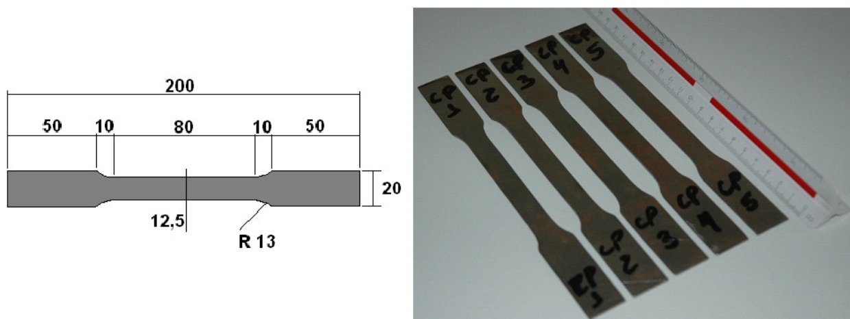
Figura 4.6: Dimensões dos corpos de prova com foto ao lado dos cinco protótipos ensaiados (dimensões em mm)
