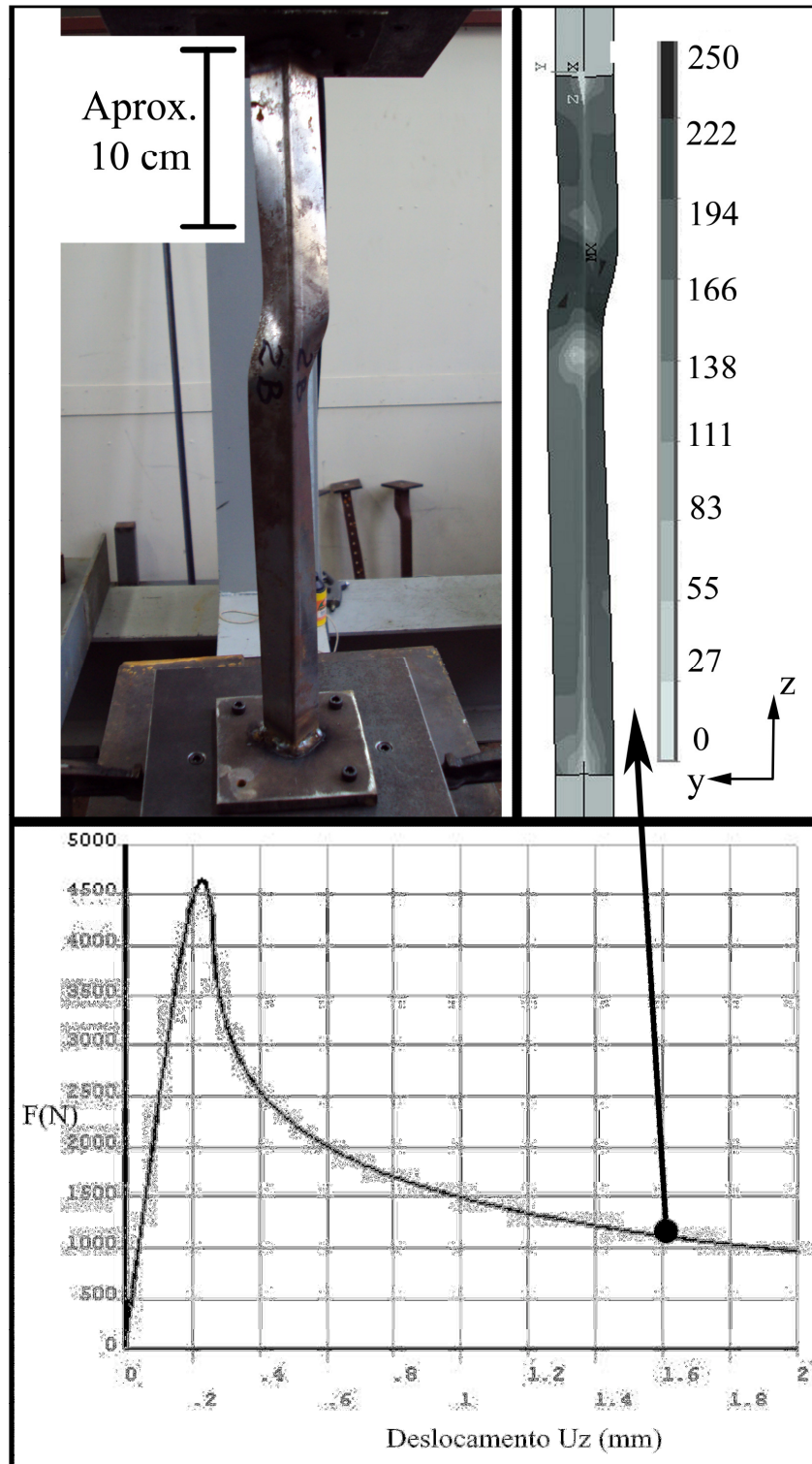
Figura 5.13: : Comparação das configurações finais obtidas experimentalmente e via MEF para a cantoneira L 27x1,06mm ( L_{teórico}=555,4 mm)
