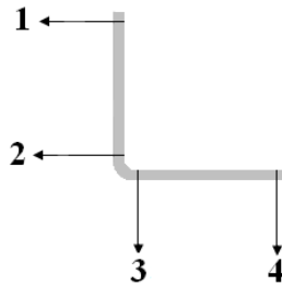
Figura 3.6: Pontos onde foram medidas as imperfeições geométricas iniciais em uma cantoneira simples (Fonte: Chodraui, 2006)
