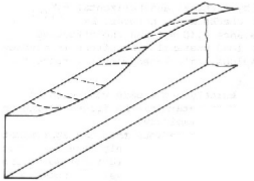
Figura 2.1: Flambagem local
