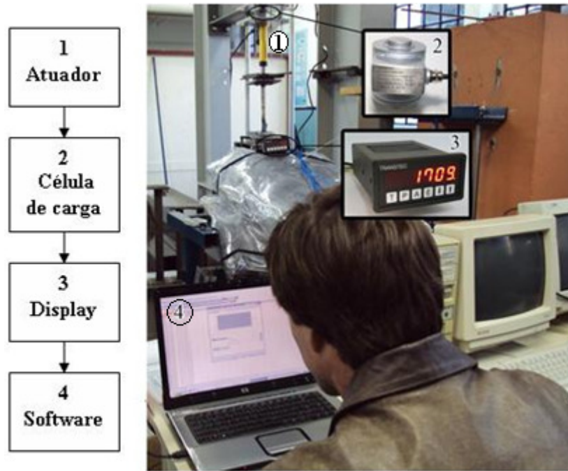
Figura 4.9: Instrumentos utilizadas nos ensaios experimentais
