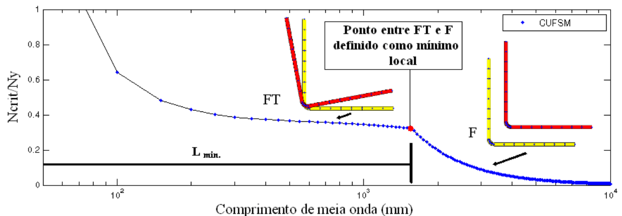
Figura 4.2: Análise de estabilidade elástica via programa CUFSM da cantoneira simples (MFF convencional)
