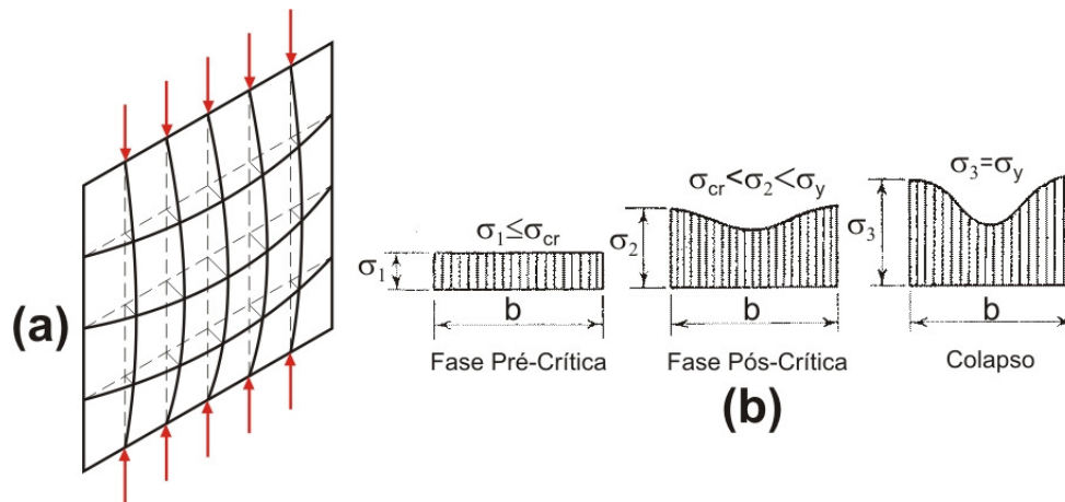
Figura 2.3: (a) Placa quadrada apoiada nos quatro lados sofrendo flambagem local. (b) Redistribuição de tensões na seção transversal da chapa
