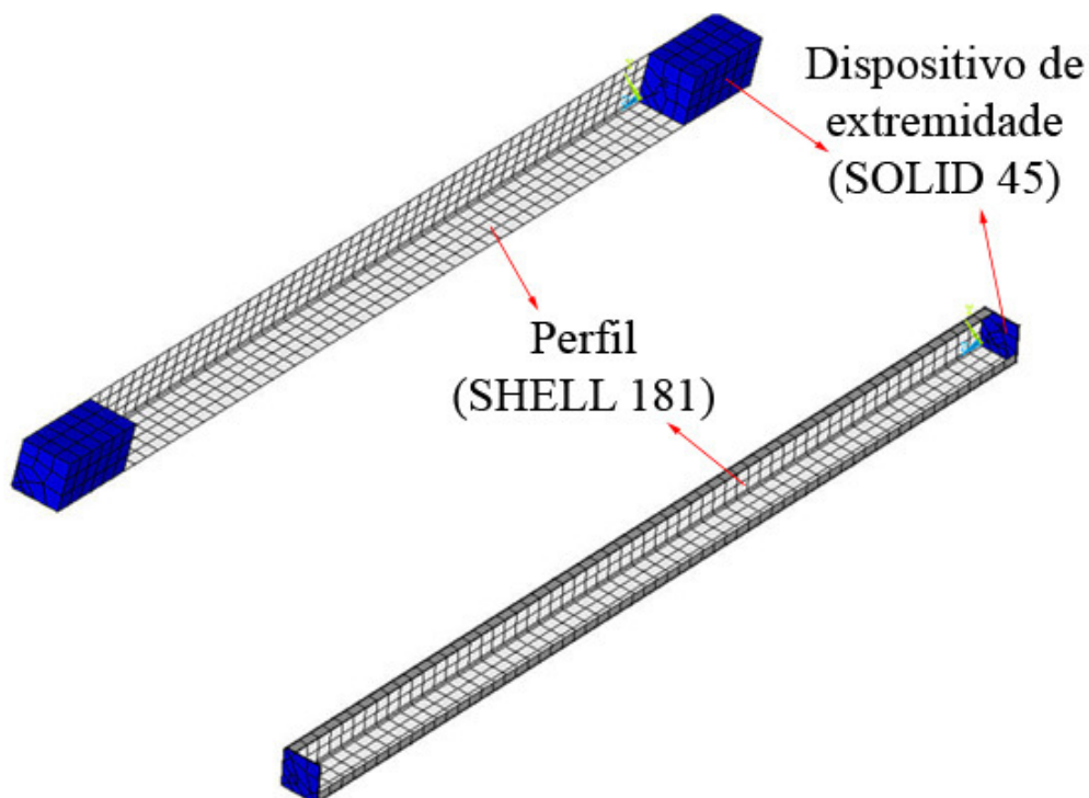
Figura 4.11: Ilustração do modelo de ambas as cantoneiras em estudo
