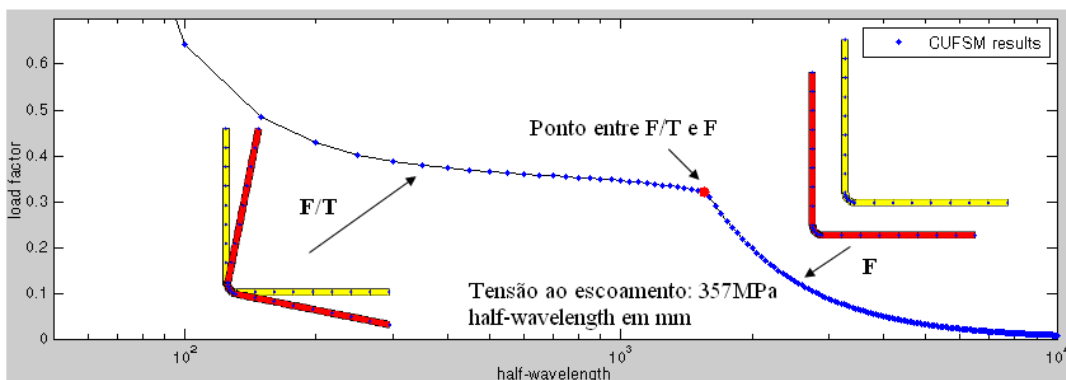
Figura 5.7: Análise de estabilidade elástica via programa CUFSM da seção L 60x2,38mm
