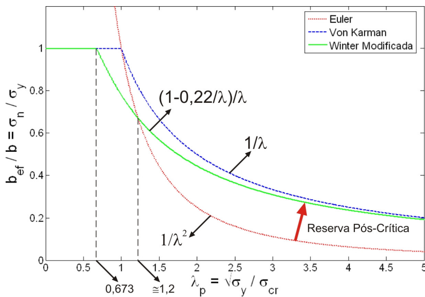
Figura 2.5: Curvas de resistência associadas à flambagem local de placas
