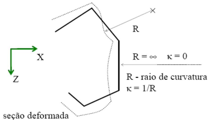
Figura 2.11: Seção transversal indeformada e deformada (Fonte: Grigoletti, 2008)
