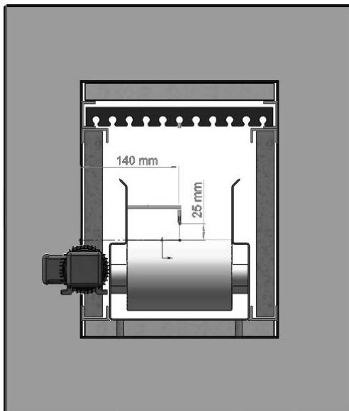
Figura 3.4 Localização dos termopares no interior do equipamento (vista lateral)
