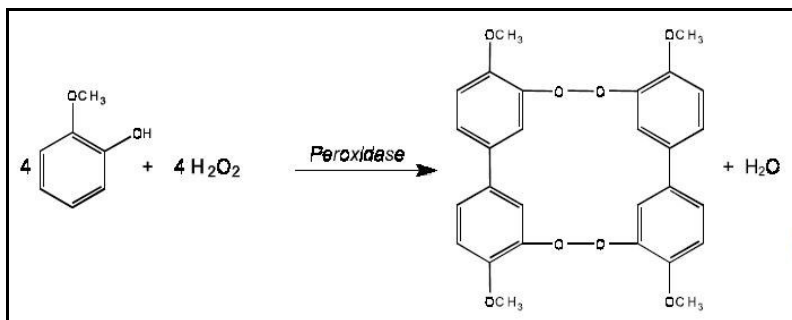
Figura 1.18 Oxidação do guaiacol à tetraguaiacol pela ação da peroxidase Fonte: Fatibello-Filho e Vieira (2002)
