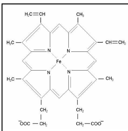
Figura 1.19 Estrutura química do grupo prostético heme ou ferro-porfirina (protoporfirina IX)
