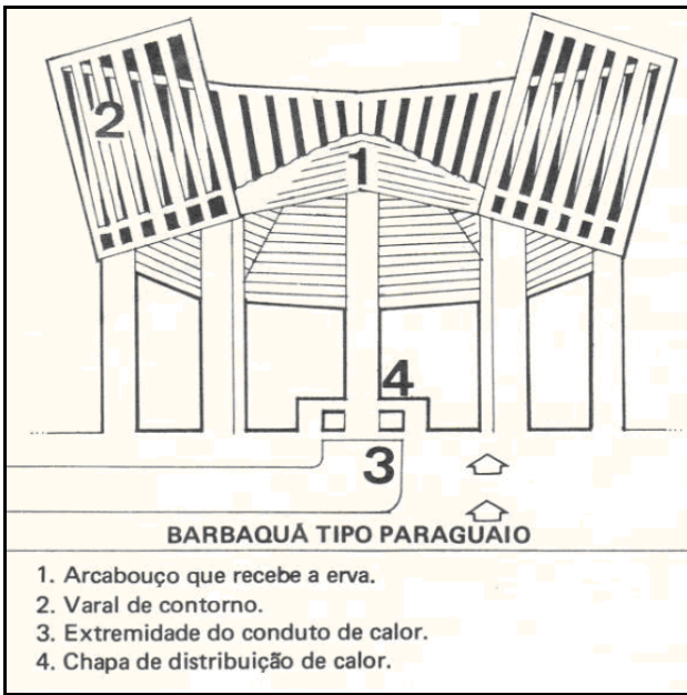
Figura 1.11 Barbaquá do tipo paraguaio Fonte: Bragagnolo (1980)
