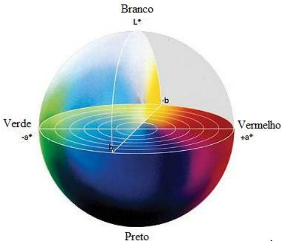
Figura 1.22 Diagrama representando o sistema de cor CIELAB Fonte: MINOLTA (2007)
