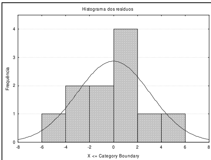
Figura 4.3 Histograma dos resíduos do modelo estatístico da atividade residual da POD em função da temperatura e do tempo de tratamento.
