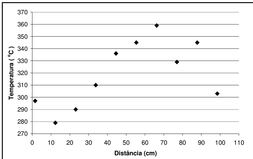
Figura 3.9 Perfil de temperatura do forno esteira no intervalo de tempo 230 a 240 min para a condição de ajuste 400 °C 40,5 Hz
