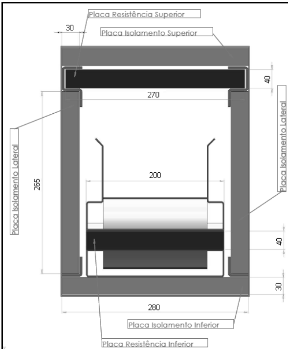
Figura 3.1 Dimensões do forno esteira estudado para o sapeco da erva-mate Fonte: LEPTEN (2007)
