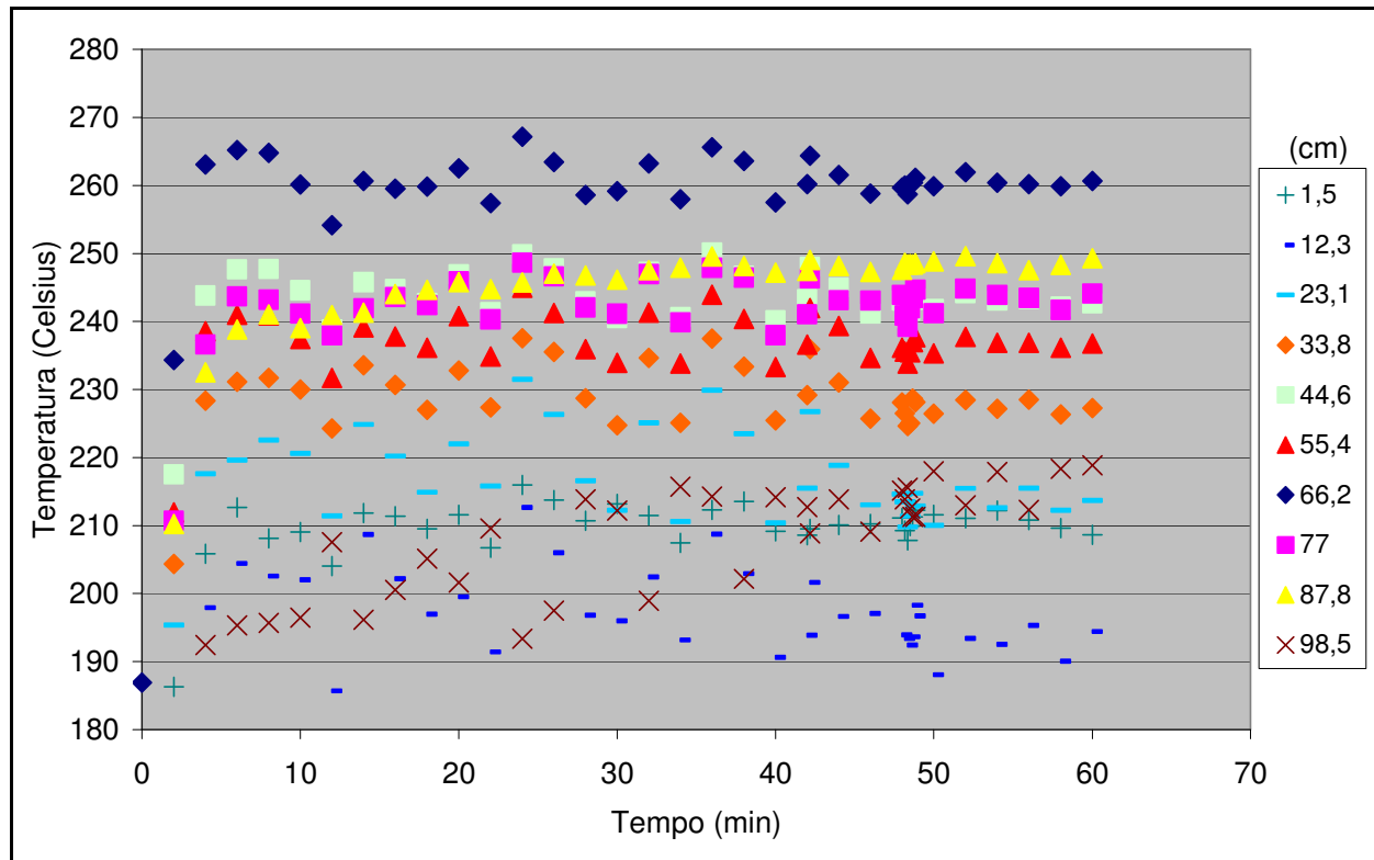
Figura 3.6 Monitoramento da temperatura do forno esteira ao longo do seu comprimento pelo período de 1 hora (300 °C 40,5 Hz)
