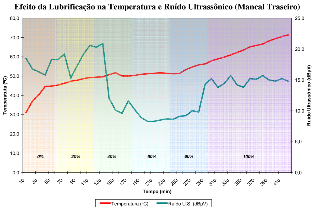
Figura 5.4 - Resultado na coleta de ruído ultrassônico e temperatura para o mancal de rolamento traseiro (Motor N°1).
