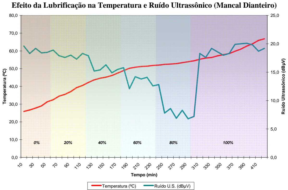
Figura 5.3 - Resultado na coleta de ruído ultrassônico e temperatura para o mancal de rolamento dianteiro (Motor N°1).
