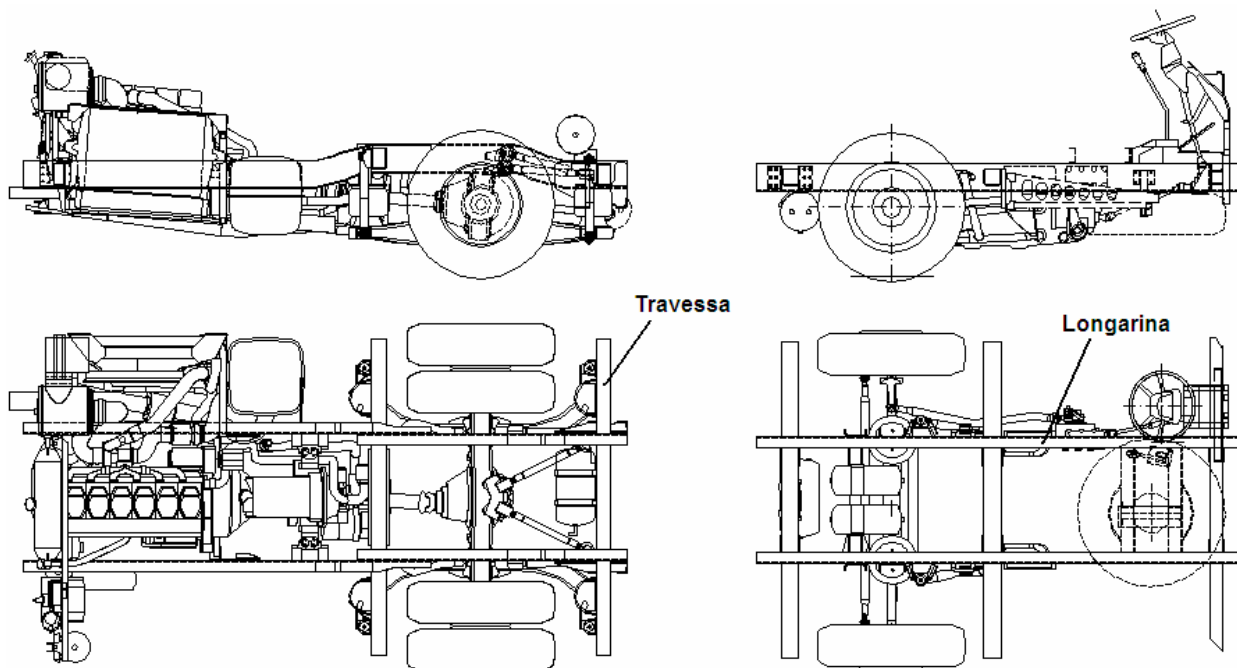
Figura 2.23: Esquema de um chassi com motor traseiro.
