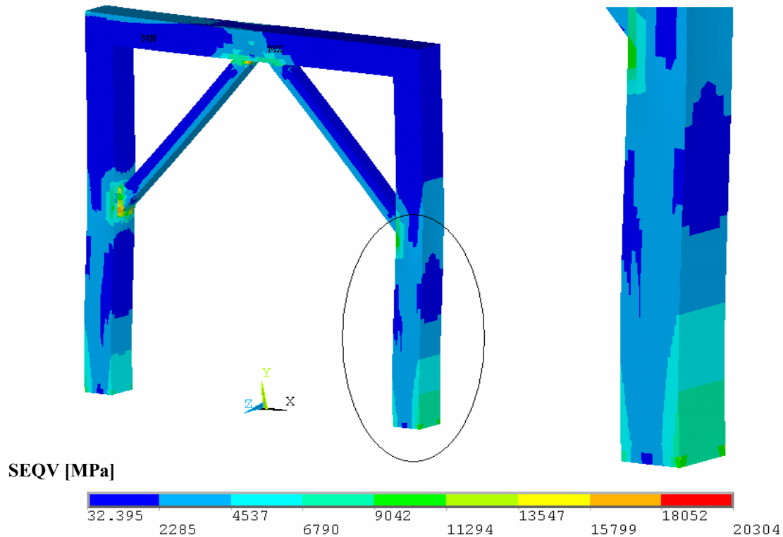
Figura 2.9: Distribuição de tensões de von Mises (em MPa) na estrutura do exemplo 1.
