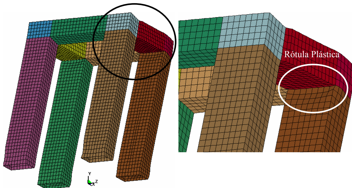
Figura 6.7: Deformação localizada na extremidade superior dos tubos verticais.
