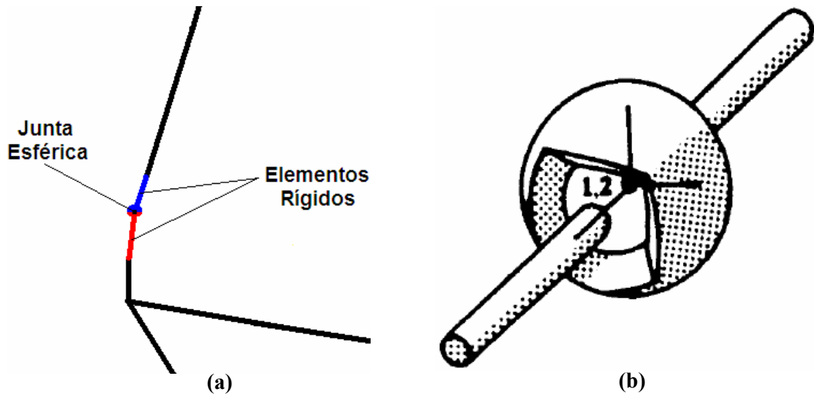
Figura 4.6: Junta esférica criada no modelo, unindo dois corpos rígidos que tem nós coincidentes em (a) e desenho esquemático da junta esférica [Ansys/Ls-Dyna, 2007] em (b).
