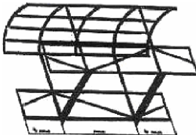
Figura 3.1: Módulo experimental correspondente ao maior passo de janelas do veículo (contém dois anéis estruturais e as uniões entre eles) [Resolução N° 811, 1996].
