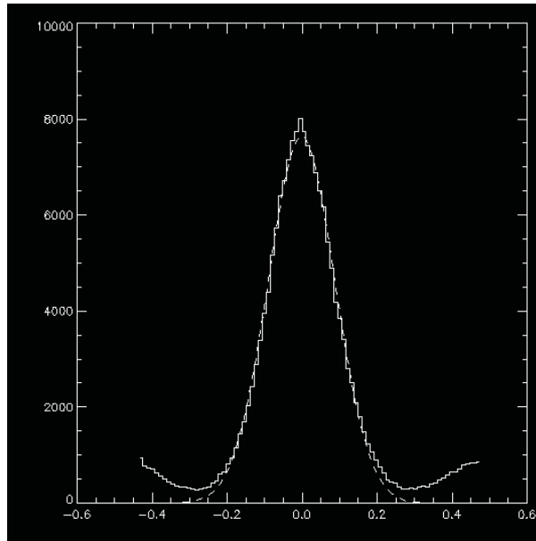
Figura 2.5: Histograma do ruído obtido para o campo do aglomerado ESO 275-01, observado em 10 de maio de 2009, com 30 segundos de exposição no filtro V.
