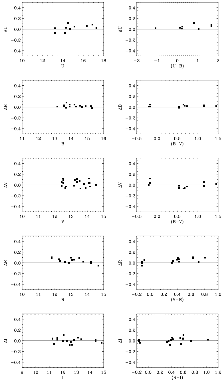
Figura 3.7: Resíduo dos ajustes para a noite de 19 de abril de 2009.
