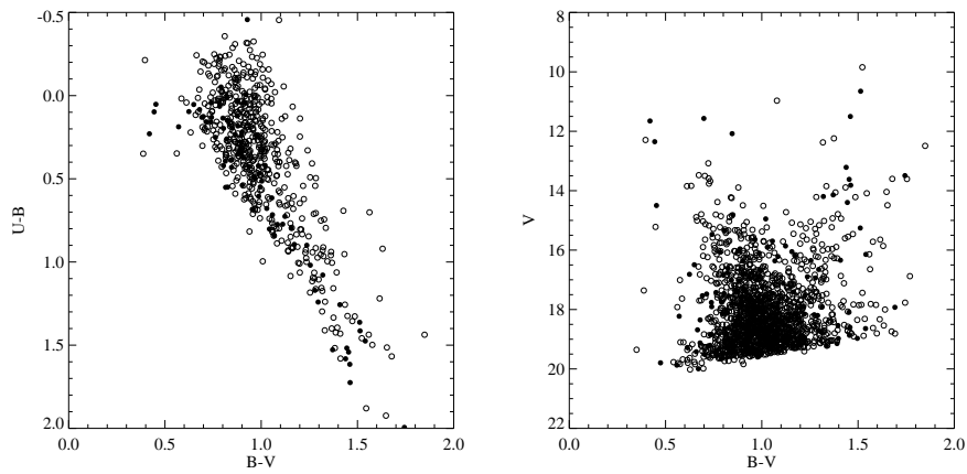
Figura 4.21: Diagramas cor-cor e cor-magnitude para as estrelas do campo do aglomerado ESO 065-07. Os círculos pretos são as estrelas que pertencem ao aglomerado, segundo critérios espaciais apenas.
