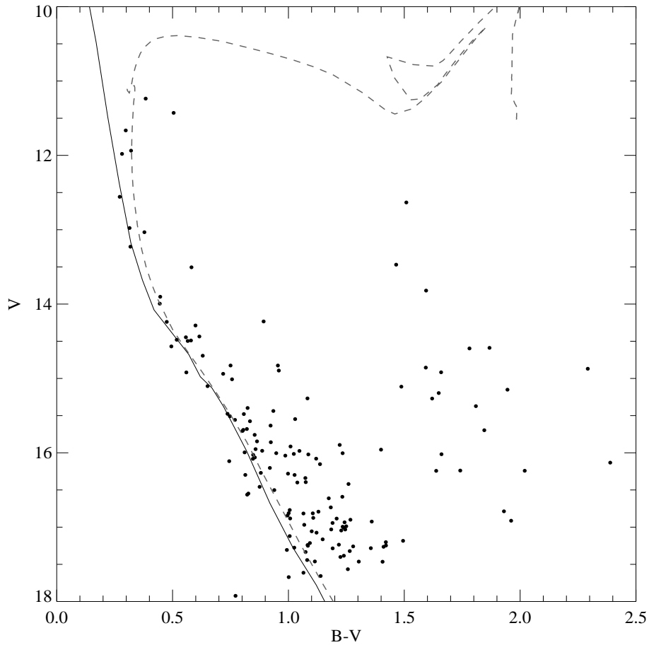
Figura 3.13: Diagrama cor-magnitude para o campo do aglomerado ESO 275-01. A linha contínua representa a ZAMS corrigida para E(B - V) igual a 0.42 magnitudes e para uma distância igual a 1670 pc. A isócrona que está representada pela linha tracejada também foi corrigida, e corresponde a uma idade de aproximadamente 178 milhões de anos.
