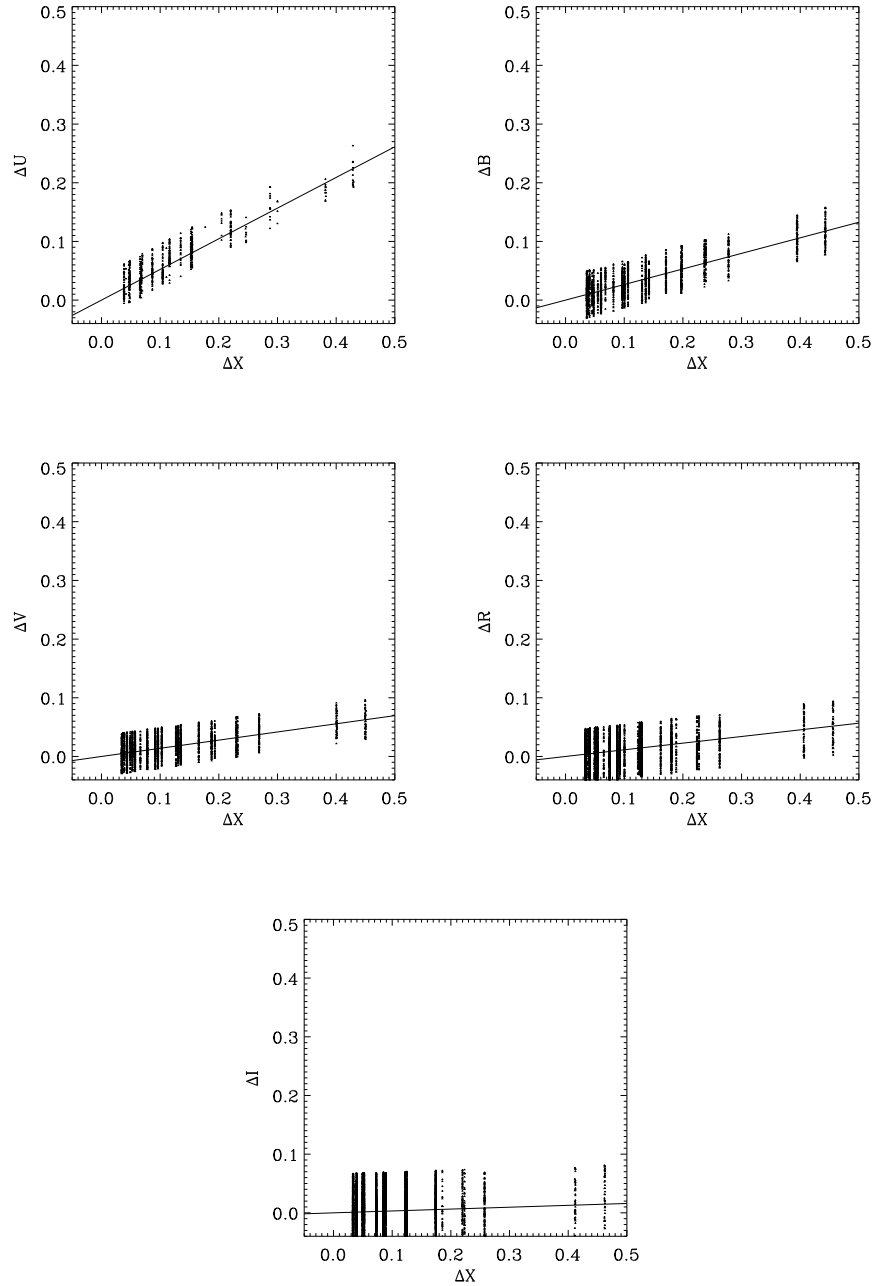
Figura 3.2: Ajustes da determinação dos coeficientes de absorção atmosférica para a noite de 18 de abril de 2009. Foram feitas 5 observações do campo na região do aglomerado ASCC-93, 5 observações para o campo do aglomerado ESO 383-10 e 3 observações para o campo do aglomerado ESO 435-09. Todos os dados foram usados no mesmo gráfico.
