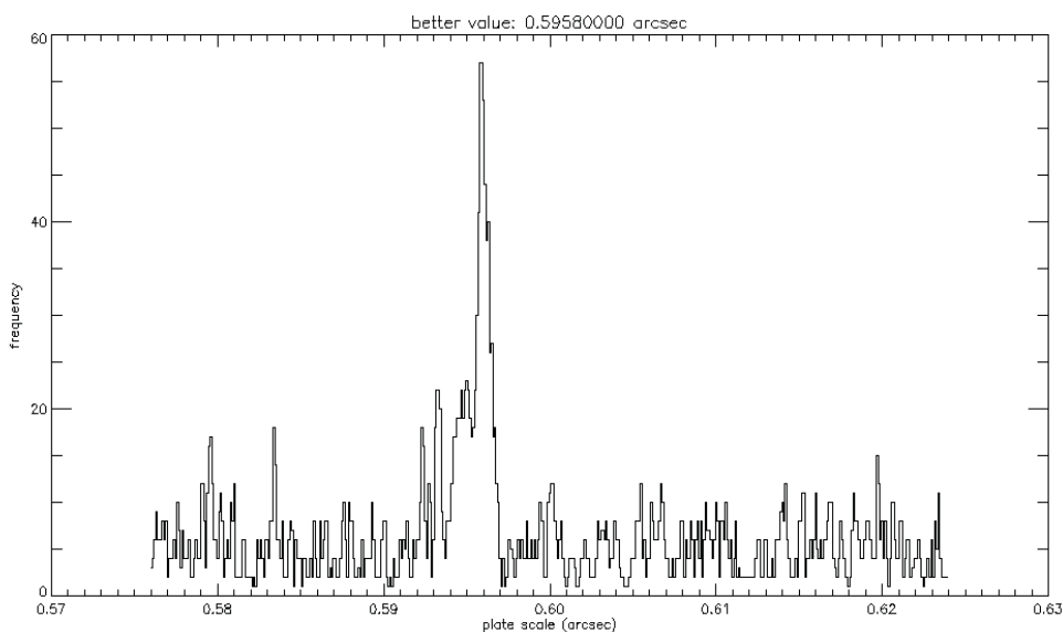
Figura 2.11: Histograma do teste de escala realizado pelo Astrometry , para o campo do aglomerado ESO 275-01, observado em 10 de maio de 2009. Foram verificados valores para a escala de placa que vão de 0.5760'' \text{ pixel}^{-1} a 0.6240'' \text{ pixel}^{-1} em passos de 0.0001'' \text{ pixel}^{-1} .
