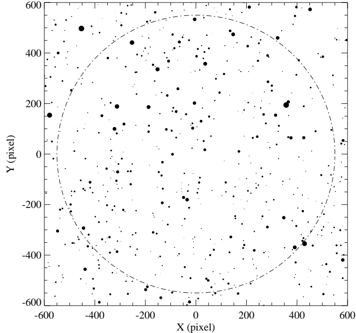
Figura 4.1: Mapa do campo do aglomerado Collinder 275 gerado a partir da lista de estrelas mostradas no CMD. O círculo tracejado indica a região do aglomerado. A escala de placa é igual a 0.600 segundos de arco por pixel. O leste aponta para cima e o norte aponta para a esquerda na figura.
