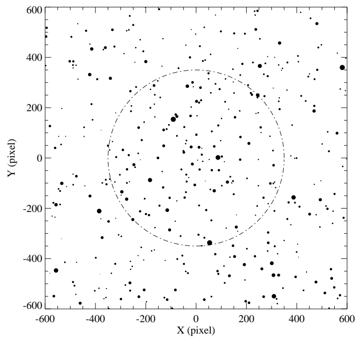
Figura 4.28: Mapa do campo do aglomerado ESO 332-20 gerado a partir da lista de estrelas mostradas no CMD. O círculo tracejado indica a região do aglomerado. A escala de placa é igual a 0.600 segundos de arco por pixel. O leste aponta para cima e o norte aponta para a esquerda na figura.
