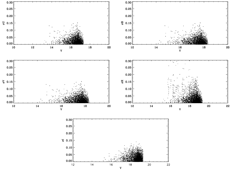
Figura 3.9: Erros estatísticos típicos associados às magnitudes instrumentais, determinados a partir das medidas do campo na região do aglomerado ESO 275-01, observado 9 vezes na noite de 10 de maio.
