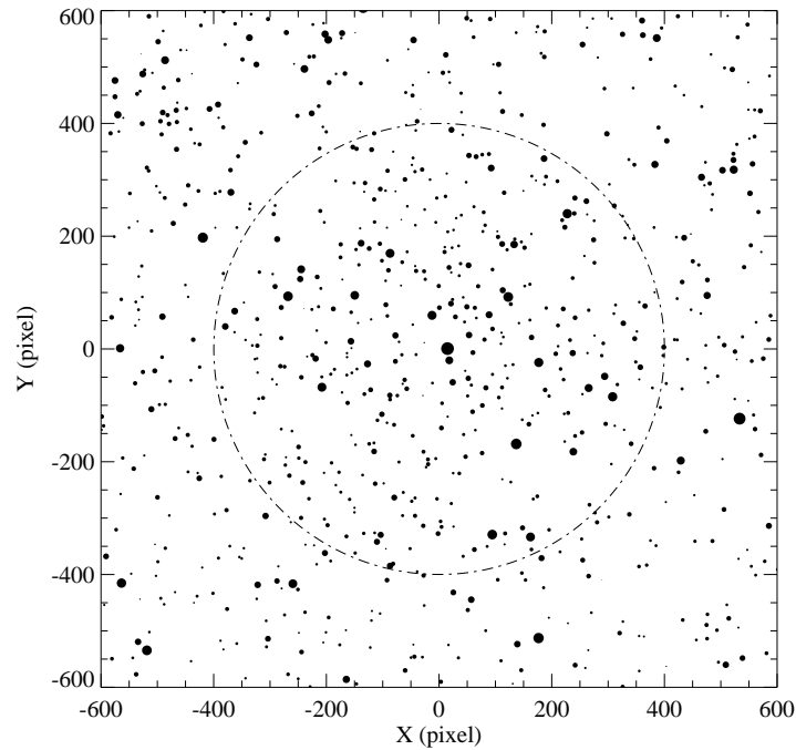
Figura 4.12: Mapa da região do aglomerado Trumpler 25, gerado a partir dos dados das estrelas que aparecem no CMD. O círculo tracejado indica a região do aglomerado. A escala de placa é 0.600 segundos de arco por pixel, o leste aponta para cima e o norte aponta para a esquerda na figura.
