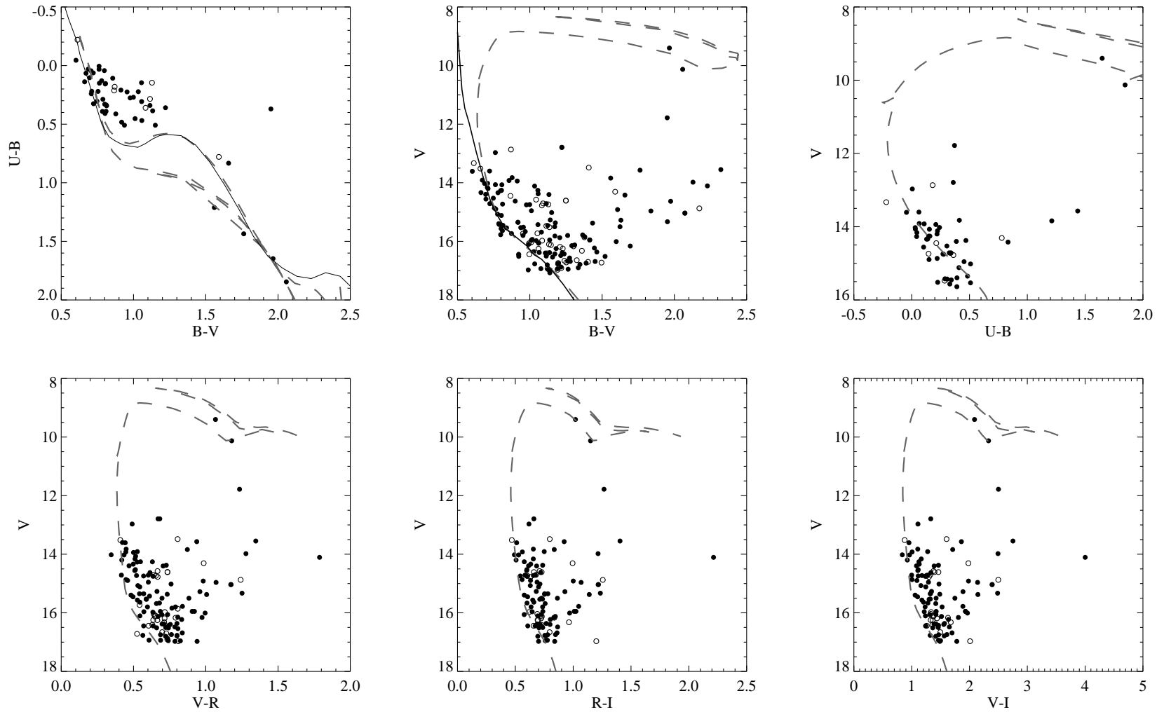
Figura 4.11: Diagramas fotométricos para Ruprecht 170. Os ajustes correspondem a E_{(B-V)} = 0.83 mag, d = 1980 pc e \log t = 7.55
