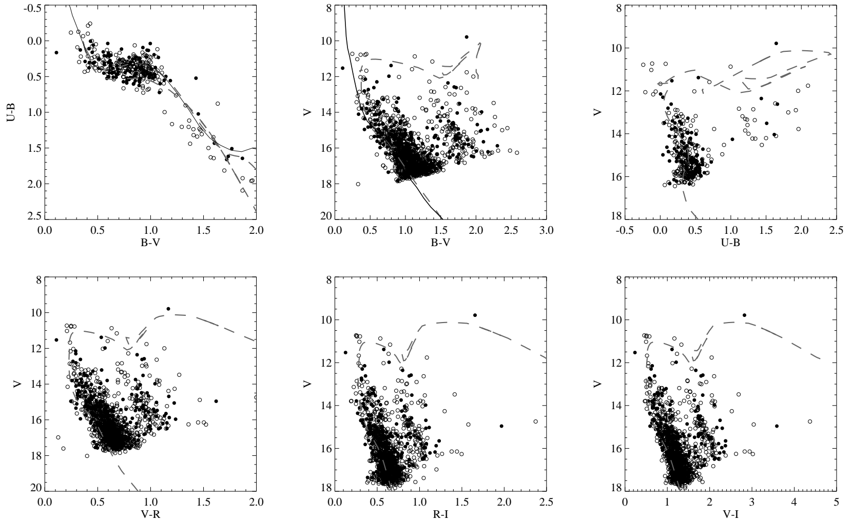
Figura 4.9: Diagramas fotométricos para Ruprecht 117. Os ajustes correspondem a E_{(B-V)} = 0.46 mag, d = 2070 pc e \log t = 8.30
