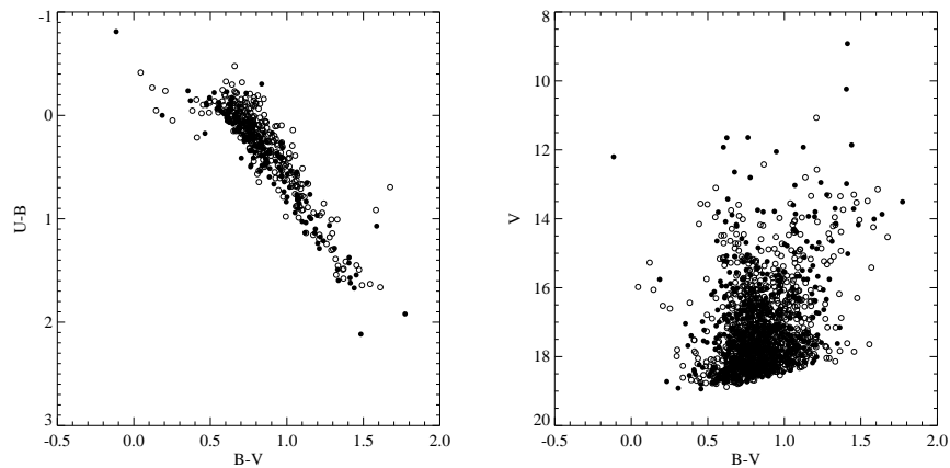
Figura 4.16: Diagramas cor-cor e cor-magnitude para o campo do aglomerado ESO 335-05. Os círculos pretos representam as estrelas na região do aglomerado, definida por seu diâmetro aparente e suas coordenadas centrais.
