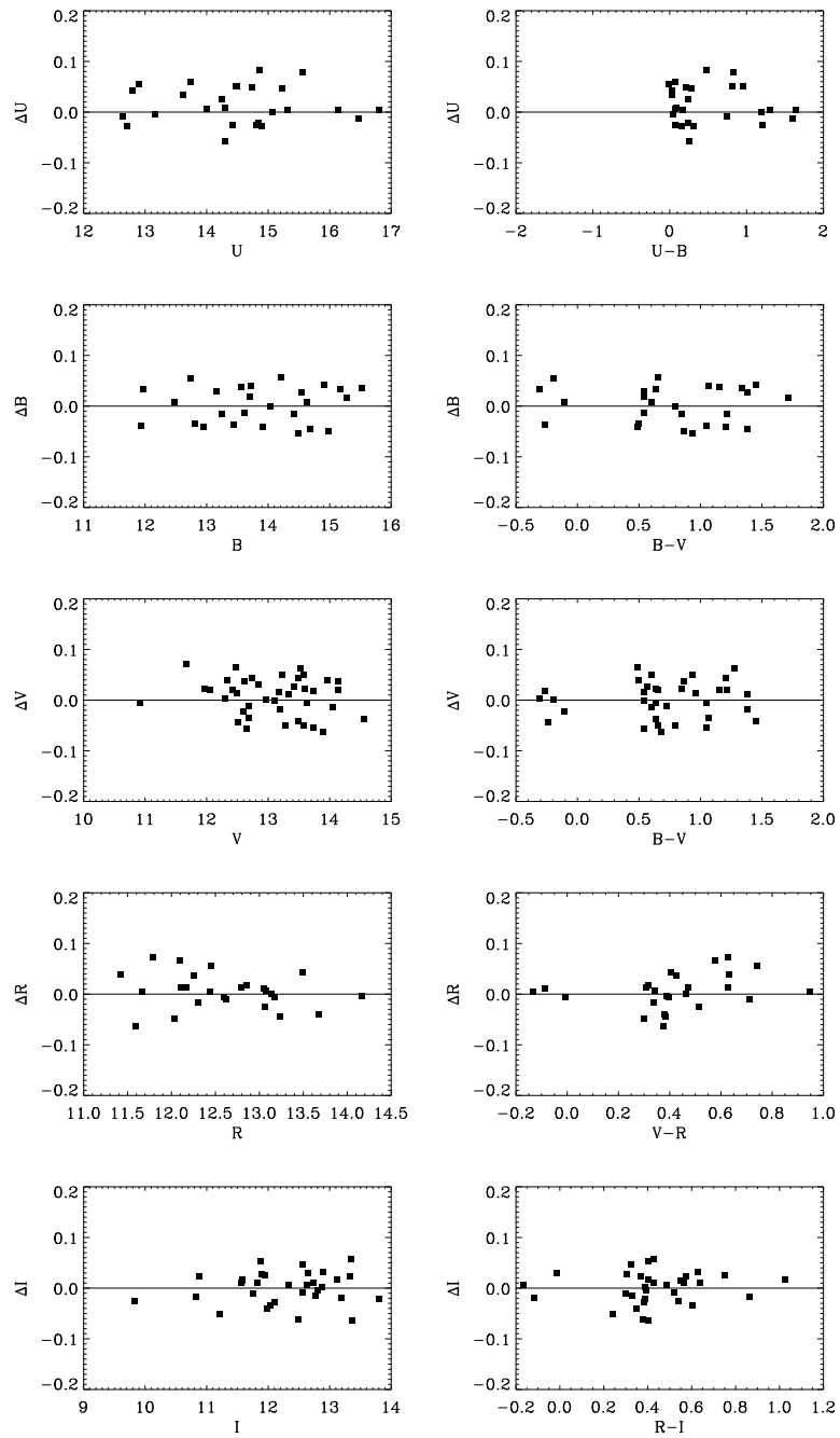
Figura 3.6: Resíduo dos ajustes para a noite de 18 de abril de 2009.
