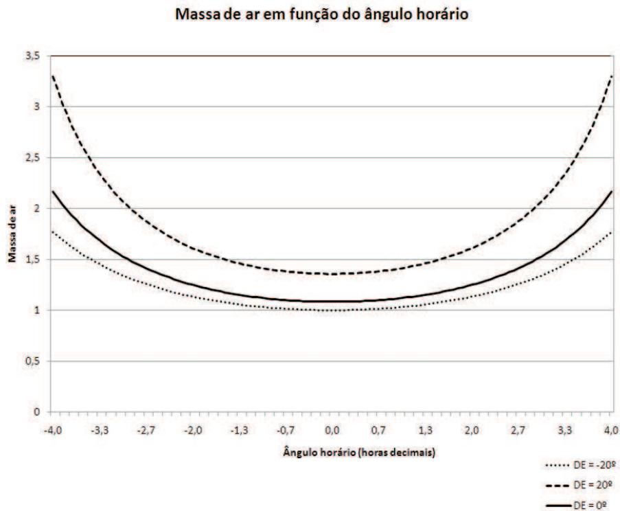
Figura 2.3: Massa de ar em função do ângulo horário para estrelas com diferentes declinações, observadas a partir do OPD. Foram consideradas três estrelas com declinações iguais a 0, 20 e -20 graus, respectivamente.
