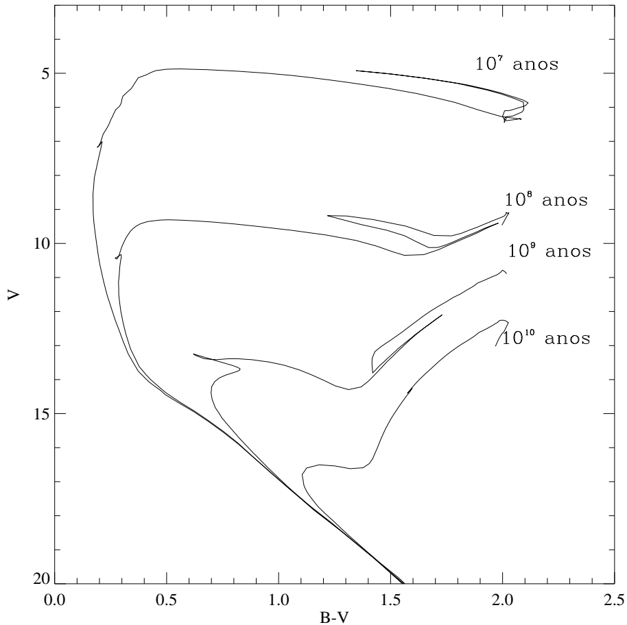
Figura 3.12: Isócronas para diferentes idades de um aglomerado.
