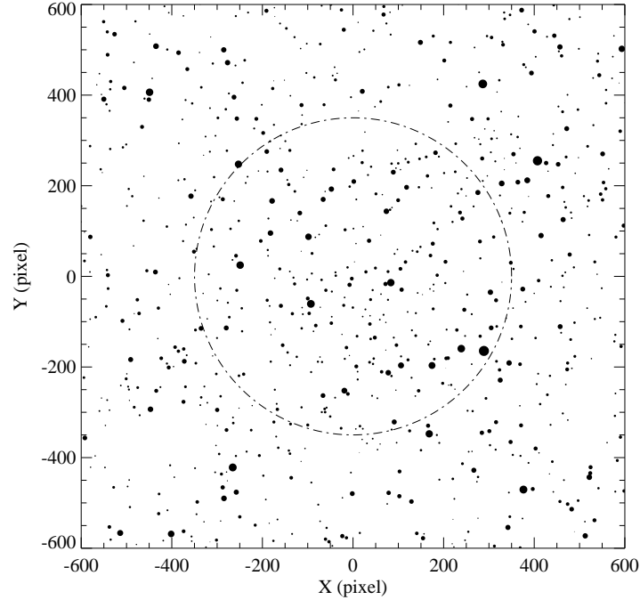
Figura 4.19: Mapa da região do aglomerado Ruprecht 176, gerado a partir dos dados das estrelas que aparecem no CMD. O círculo tracejado indica a região do aglomerado. A escala de placa é 0.600 segundos de arco por pixel, o leste aponta para cima e o norte aponta para a esquerda na figura.
