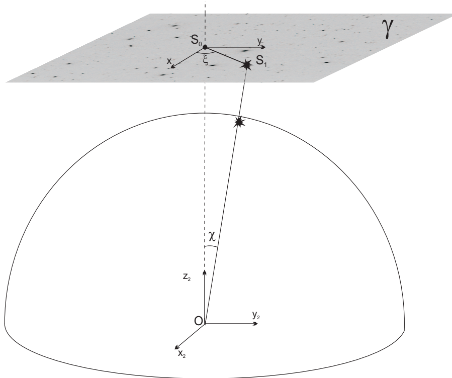
Figura 2.10: Representação do sistema de coordenadas após as operações de rotação realizadas durante a astrometria.
