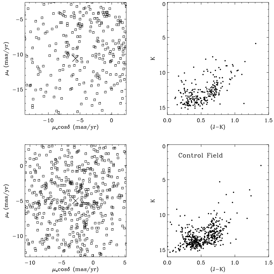
Figura 4.15: VPDs e CMDs para o campo do aglomerado ESO 137-23 e para o campo de controle
