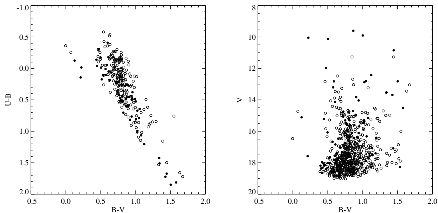
Figura 4.26: Diagramas cor-cor e cor-magnitude para as estrelas no campo do aglomerado ESO 281-24. Os círculos pretos representam as estrelas pertencentes ao aglomerado, considerando-se apenas critérios espaciais.
