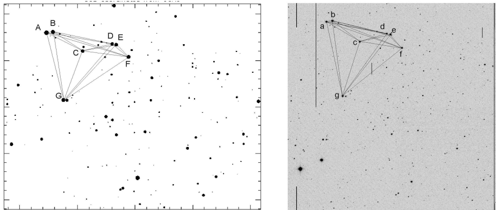
Figura 2.12: À esquerda: projeção de um campo padrão de Landolt (2007). À direita: imagem observada do mesmo campo.
