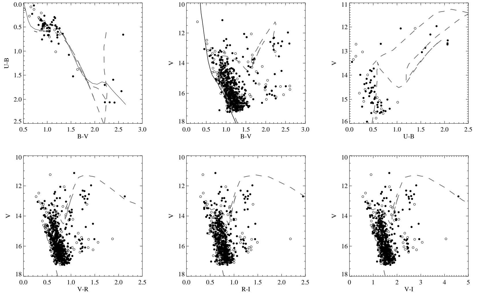
Figura 4.13: Diagramas fotométricos para Trumpler 25. Os ajustes correspondem a E_{(B-V)} = 0.65 mag, d = 1800 pc e \log t = 8.85
