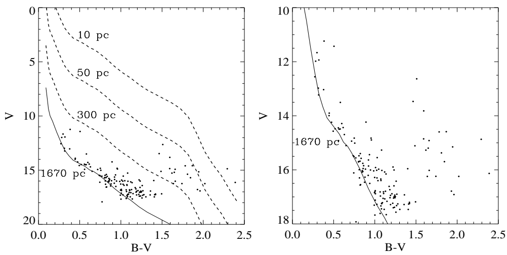
Figura 3.11: Diagrama cor-magnitude para o ESO 275-01. À esquerda: os dados do aglomerado são representados por pontos. As linhas tracejadas representam a ZAMS com os valores da magnitude V corrigidos para diferentes distâncias, indicadas no diagrama. A linha contínua representa a ZAMS para uma distância de 1670 pc, considerado o melhor ajuste. À direita: o mesmo diagrama foi feito com uma escala diferente para mostrar a qualidade do ajuste. Apenas a ZAMS corrigida para uma distância de 1670 pc foi representada no diagrama por uma linha contínua.
