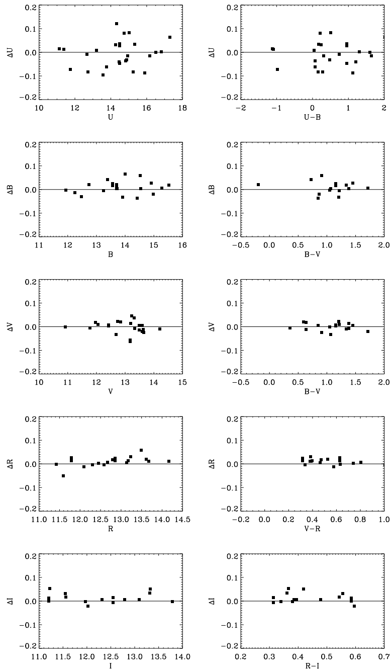
Figura 3.5: Resíduo dos ajustes para a noite de 17 de abril de 2009.
