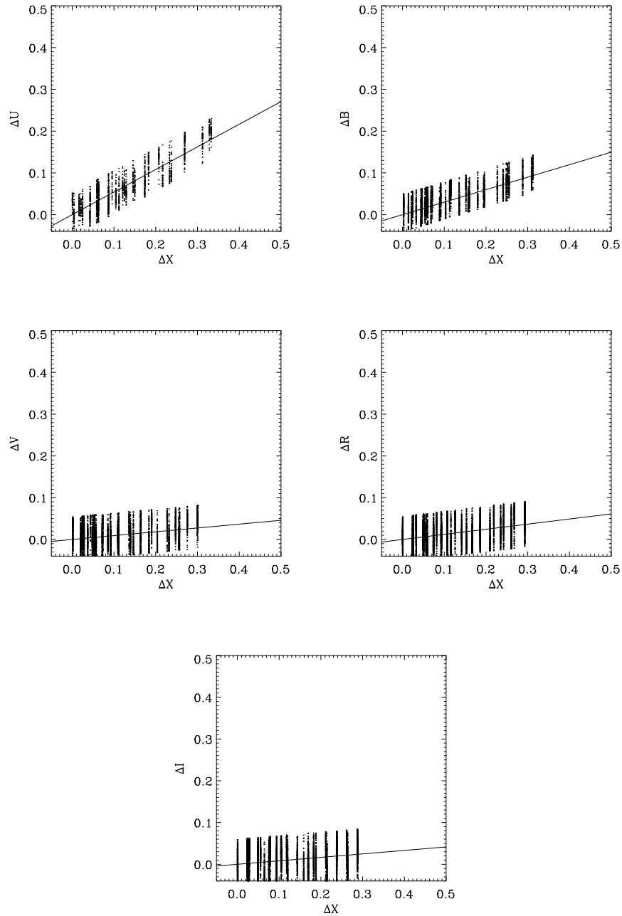
Figura 3.4: Ajustes da determinação dos coeficientes de absorção atmosférica para a noite de 10 de maio de 2009. O campo do aglomerado ESO 275-01 foi observado 9 vezes no total.
