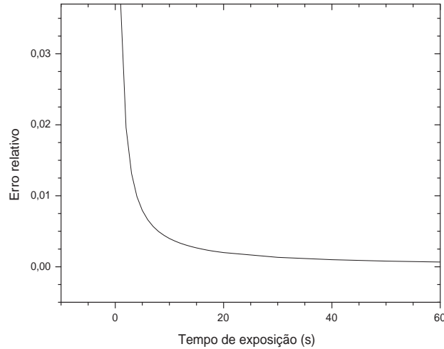
Figura 2.2: Erro relativo do fluxo de uma estrela devido ao tempo de abertura e fechamento do obturador, em função do tempo de exposição.
