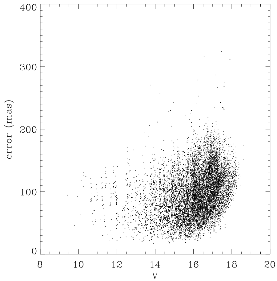
Figura 2.16: Distribuição típica dos erros astrométricos em função da magnitude V .
