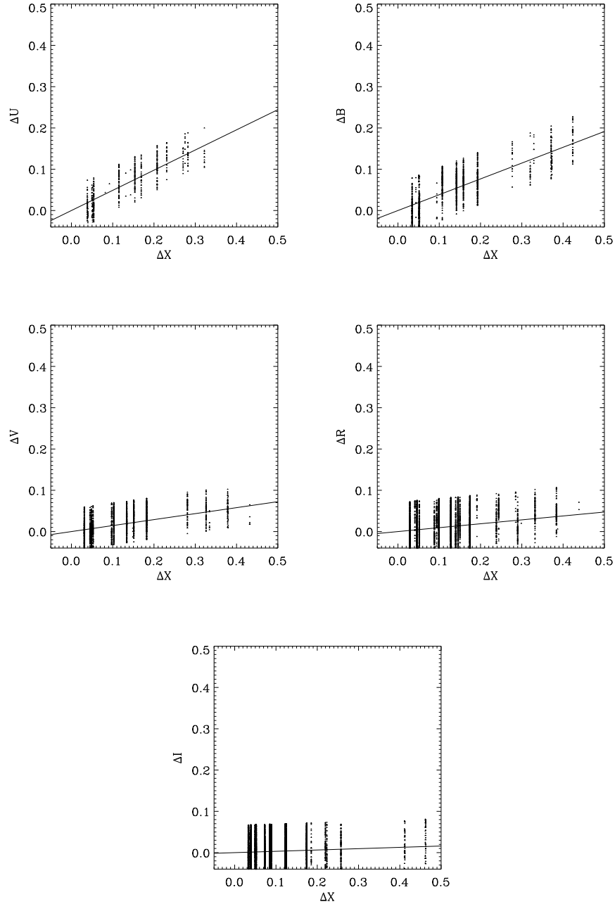
Figura 3.3: Ajustes da determinação dos coeficientes de absorção atmosférica para a noite de 19 de abril de 2009. O campo na região do aglomerado ASCC-93 foi observado 4 vezes e o campo do aglomerado ESO 435-09 foi observado 7 vezes. Os dados foram reunidos no mesmo gráfico.
