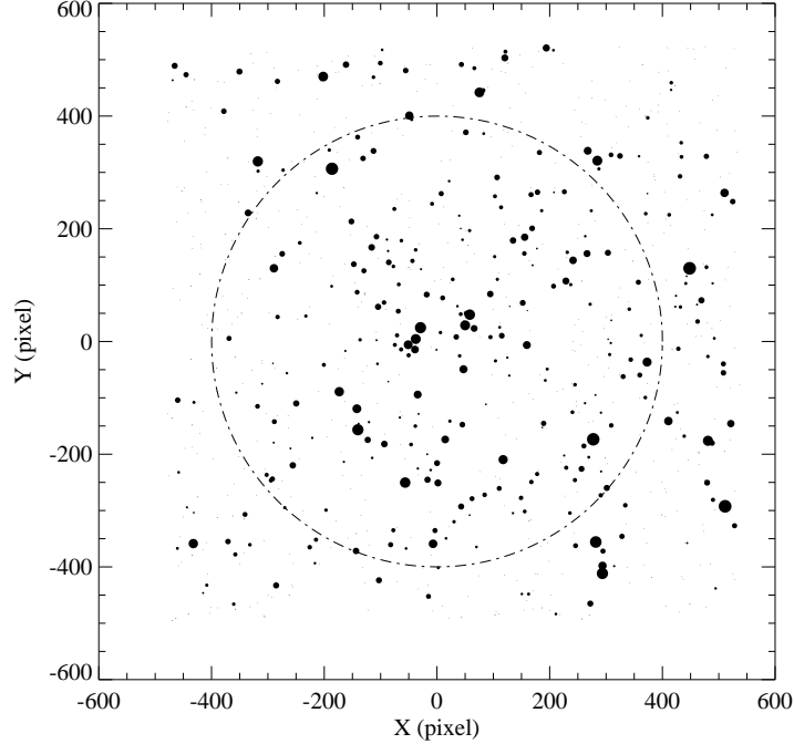
Figura 4.3: Mapa do campo do aglomerado ESO 275-01. O círculo tracejado indica a região do aglomerado. A escala de placa é 0.600 segundos de arco por pixel, o leste aponta para cima e o norte aponta para a esquerda na figura.
