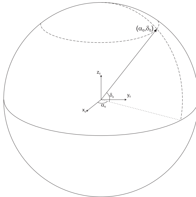
Figura 2.6: Representação da Esfera Celeste
