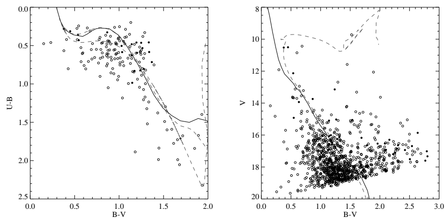
Figura 4.31: Diagramas fotométricos para o aglomerado Loden 1202. Os ajustes correspondem a E_{(B-V)} = 0.39 mag, d = 780 pc e \log t = 8.55 anos.
