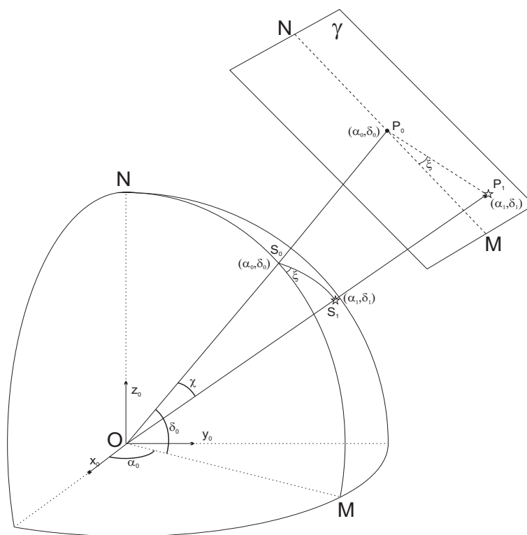
Figura 2.7: Esquema da projeção gnomônica de dois pontos da Esfera Celeste
