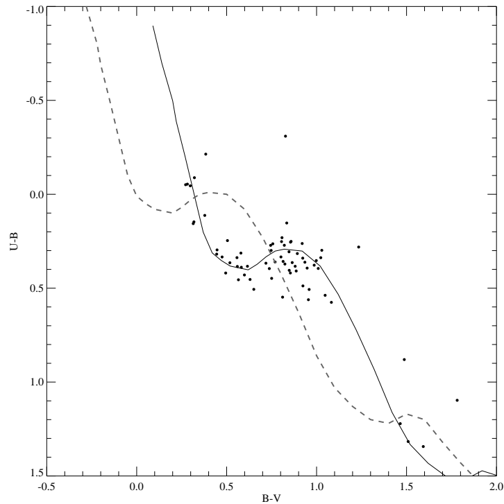
Figura 3.10: Diagrama (U - B) \times (B - V) para os dados do campo do aglomerado ESO 275-01, observado em 10 de maio. A linha tracejada representa a ZAMS sem excesso de cor e a linha contínua é a ZAMS corrigida para um excesso de cor igual a 0.42 magnitudes.
