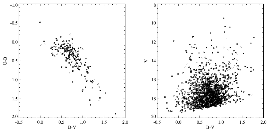
Figura 4.14: Diagramas cor-cor e cor-magnitude para o campo do aglomerado ESO 137-23. Os círculos pretos representam as estrelas na região do aglomerado, definida por seu diâmetro aparente e suas coordenadas centrais.
