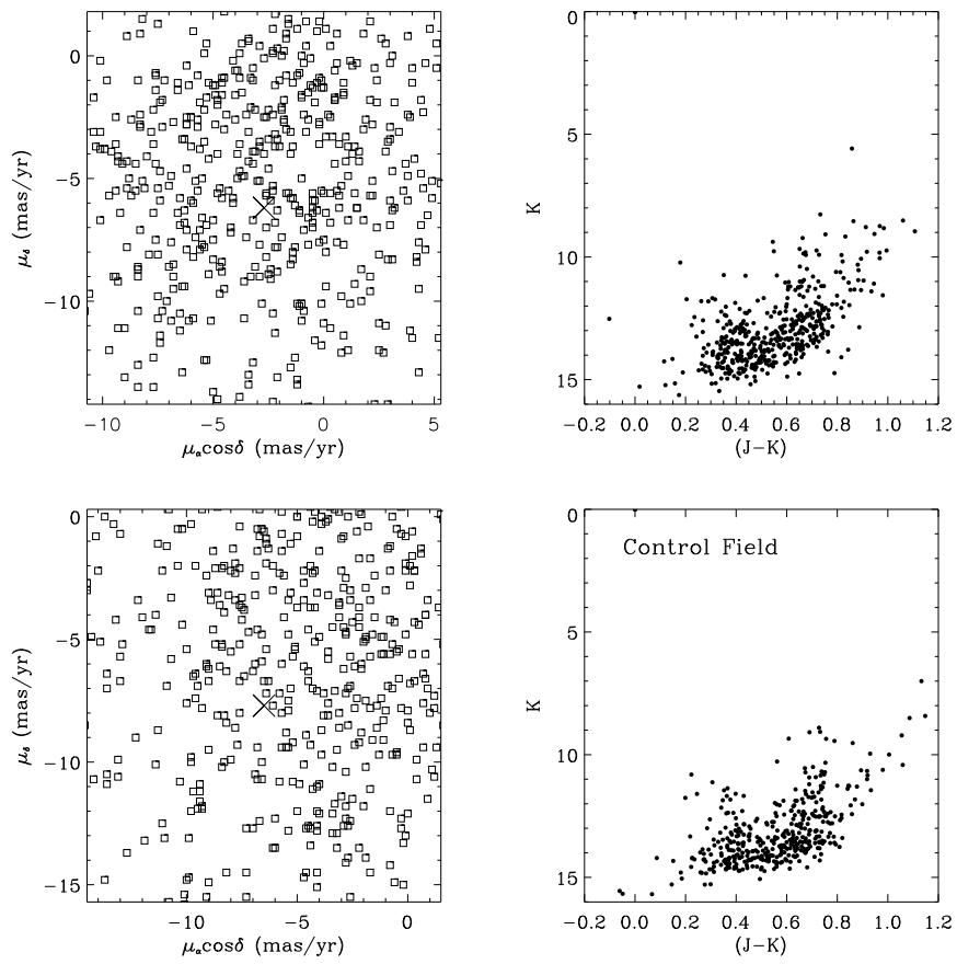
Figura 4.17: VPDs e CMDs para o campo do aglomerado ESO 335-05 e para o campo de controle.
