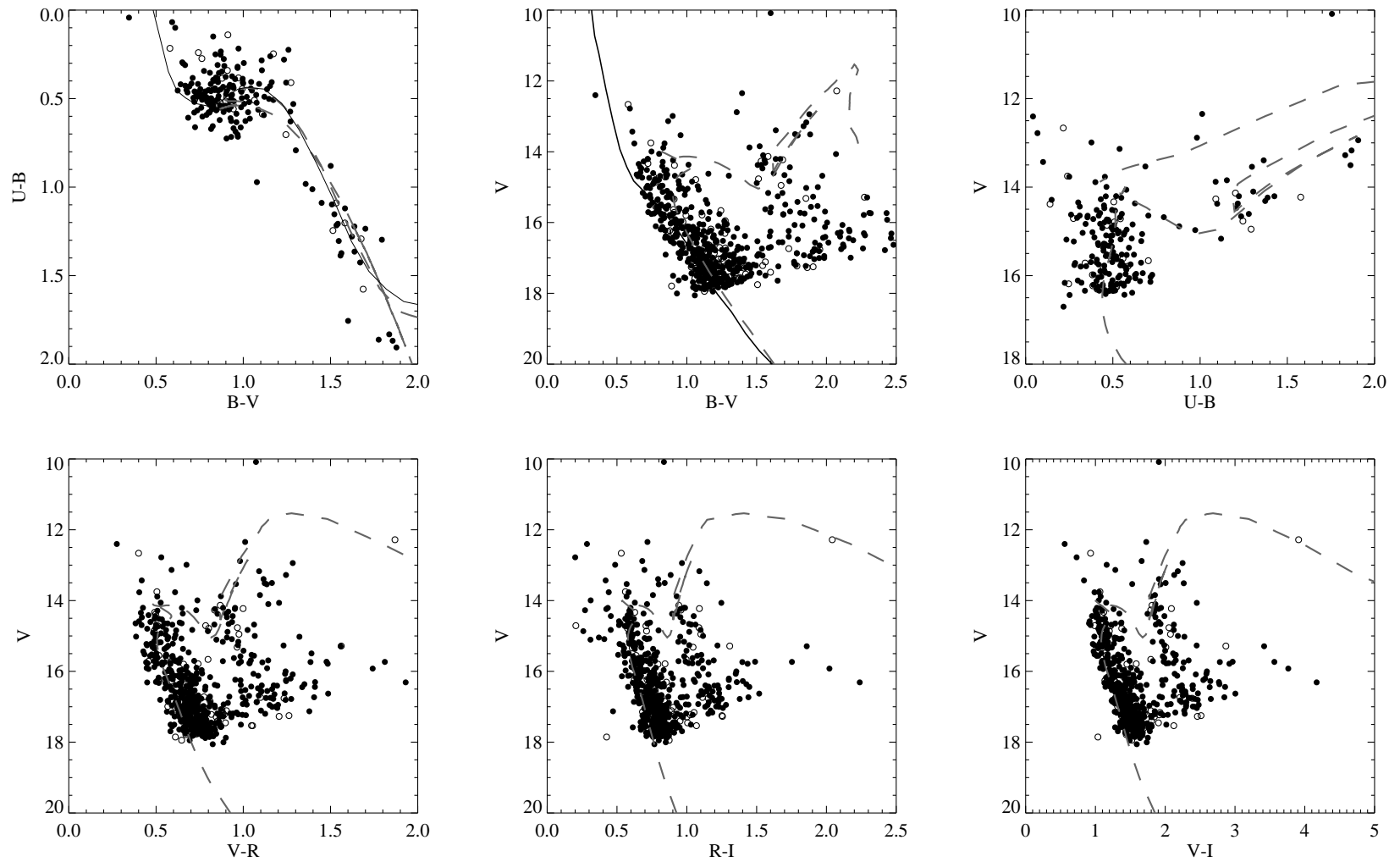
Figura 4.7: Diagramas fotométricos para Ruprecht 112. Os ajustes correspondem a E_{(B-V)} = 0.62 mag, d = 1910 pc e \log t = 9.00
