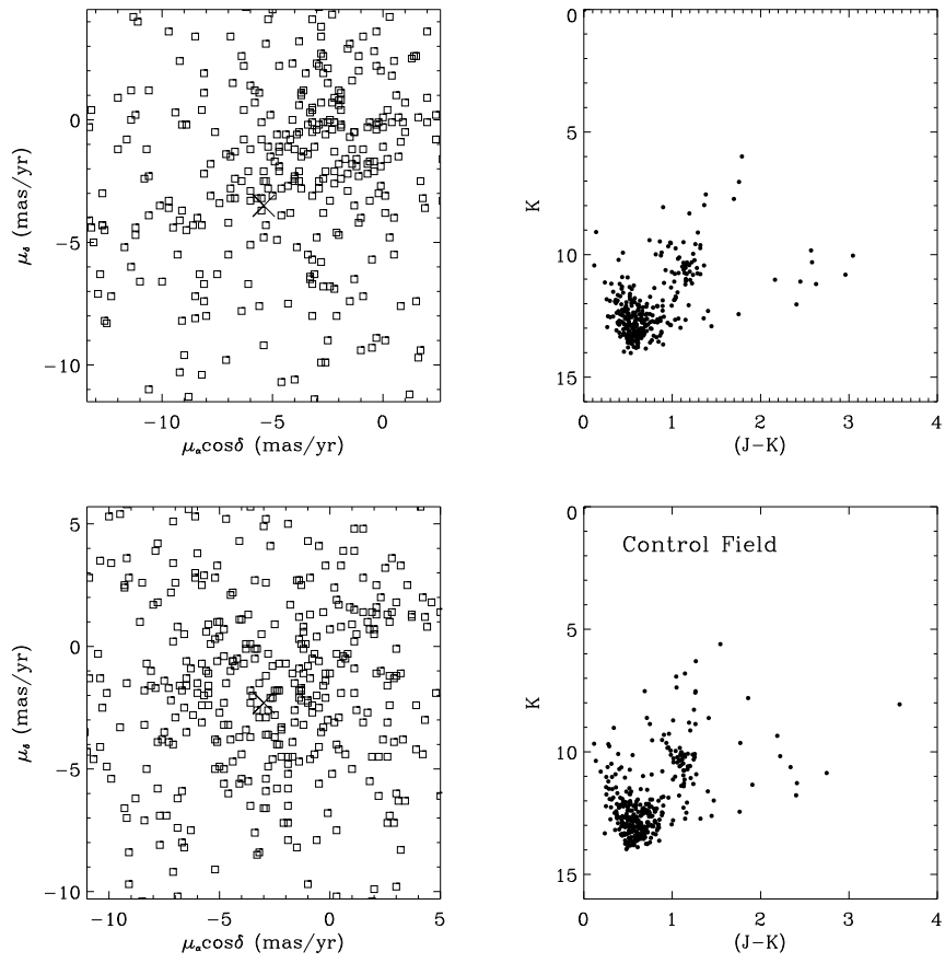
Figura 4.23: VPDs e CMDs para o campo do ESO 134-12 e para o campo de controle.
