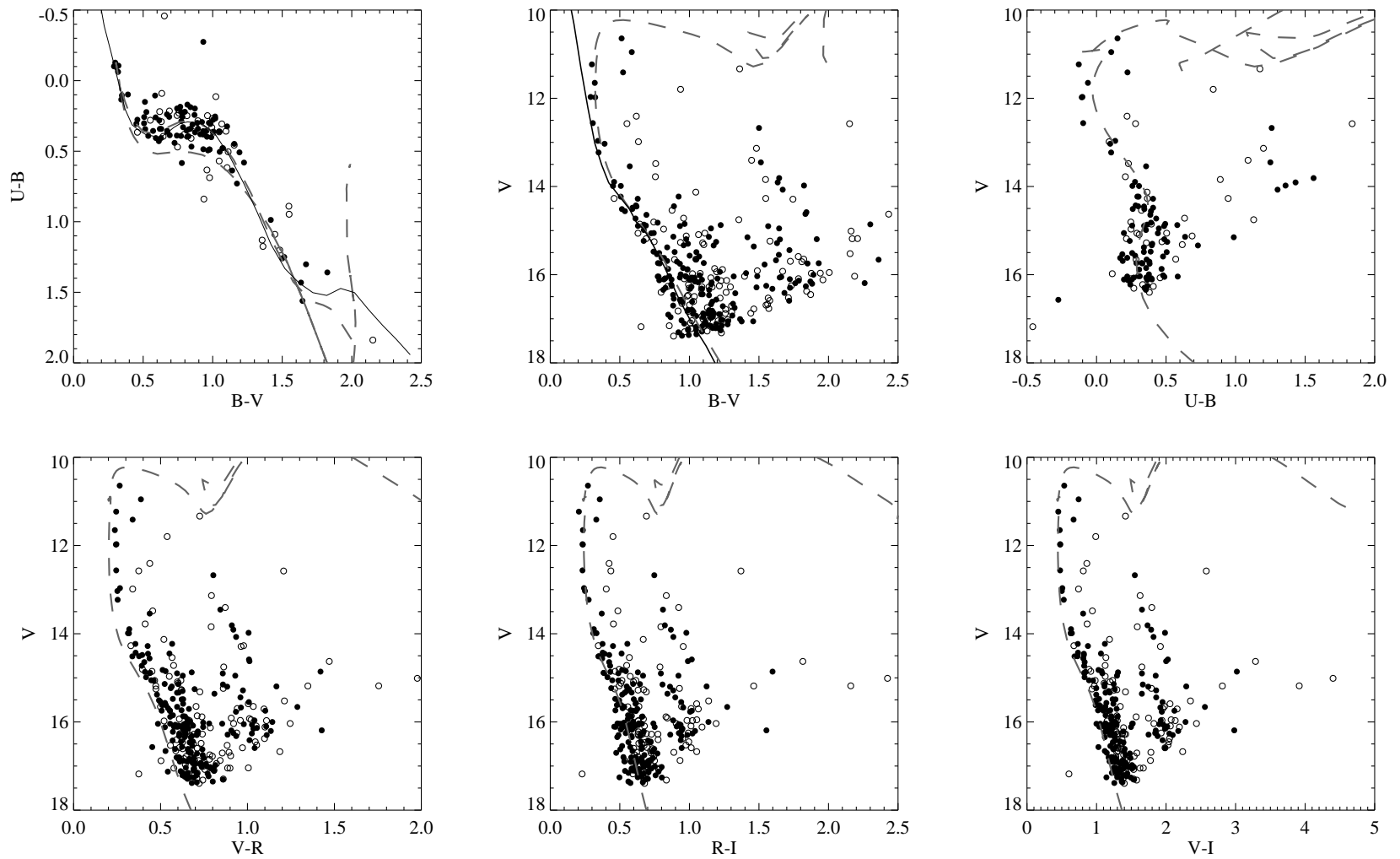
Figura 4.5: Diagramas fotométricos para o ESO 275-01. Os ajustes correspondem a E_{(B-V)} = 0.42 mag, d = 1670 pc e \log t = 8.25
