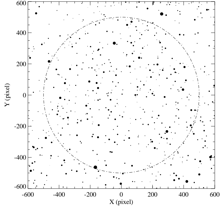
Figura 4.6: Mapa da região do aglomerado Ruprecht 112, gerado a partir dos dados das estrelas que aparecem no CMD. O círculo tracejado indica a região do aglomerado. A escala de placa é 0.600 segundos de arco por pixel, o leste aponta para cima e o norte aponta para a esquerda na figura.
