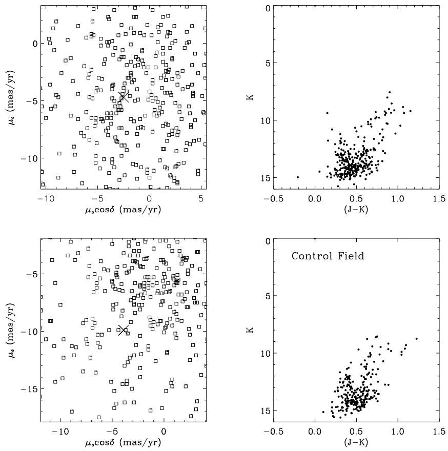
Figura 4.27: VPDs e CMDs para o campo do aglomerado ESO 281-24 e para o campo de controle.
