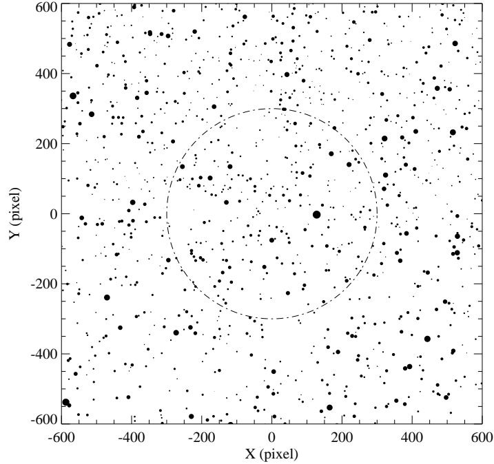
Figura 4.8: Mapa da região do aglomerado Ruprecht 117, gerado a partir dos dados das estrelas que aparecem no CMD. O círculo tracejado indica a região do aglomerado. A escala de placa é 0.600 segundos de arco por pixel, o leste aponta para cima e o norte aponta para a esquerda na figura.
