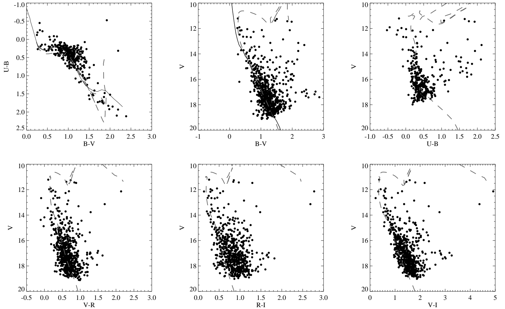
Figura 4.33: Diagramas fotométricos para o aglomerado Ruprecht 133. Os ajustes correspondem a E_{(B-V)} = 0.30 mag, d = 1670 pc e \log t = 8.50 anos.
