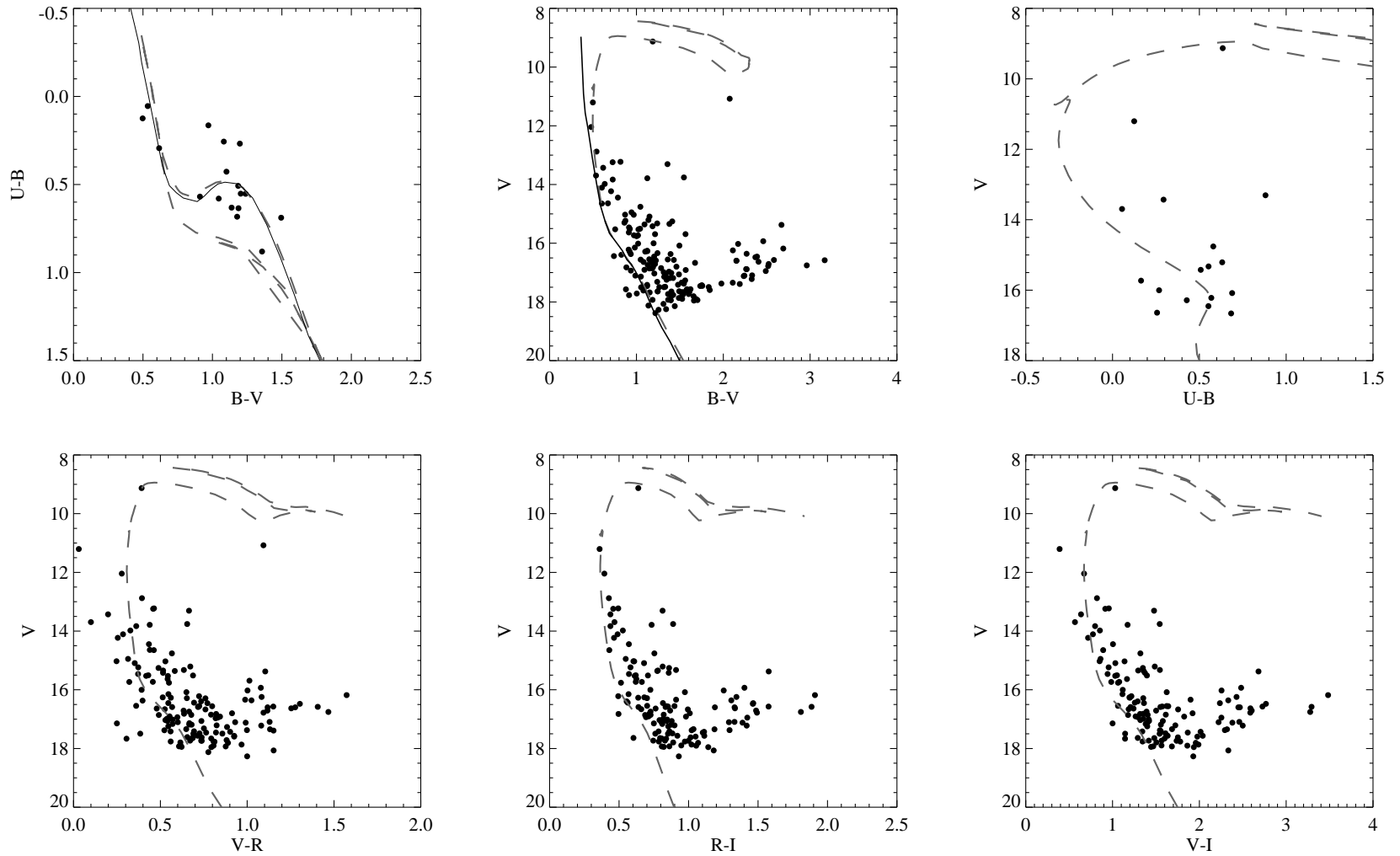
Figura 4.29: Diagramas fotométricos para o aglomerado ESO 332-20. Os ajustes correspondem a E_{(B-V)} = 0.69 mag, d = 2540 pc e \log t = 7.55 anos.
