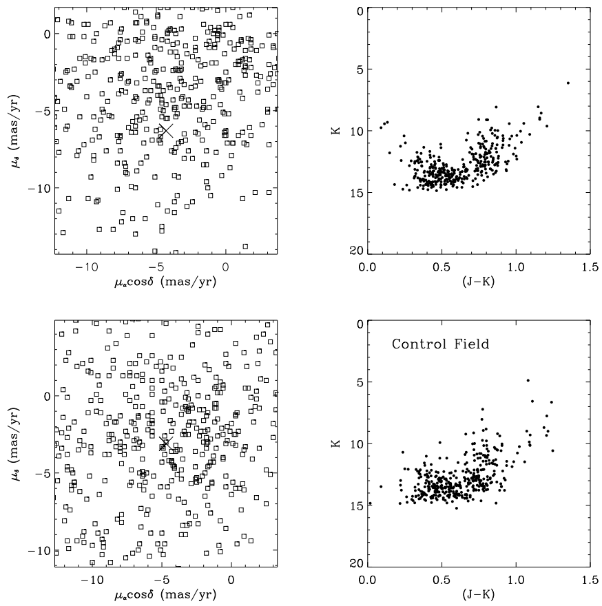
Figura 4.22: VPDs e CMDs para o aglomerado ESO 065-07 e para o campo de controle
