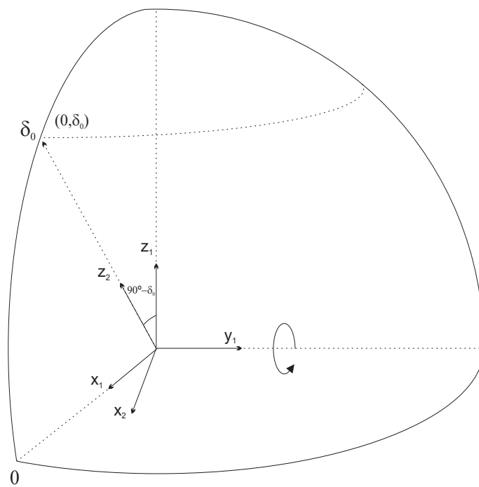
Figura 2.9: Rotação do sistema de referências em torno do eixo y_1 . O ângulo de rotação é igual ao complemento da declinação de apontamento.
