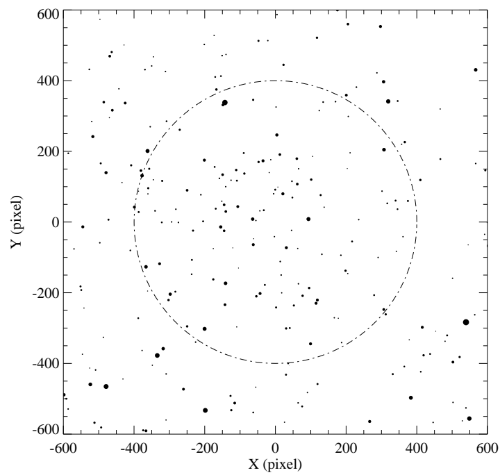
Figura 4.24: Mapa da região do aglomerado ESO 134-12, gerado a partir dos dados das estrelas que aparecem no CMD. O círculo tracejado indica a região do aglomerado. A escala de placa é 0.600 segundos de arco por pixel, o leste aponta para cima e o norte aponta para a esquerda na figura.
