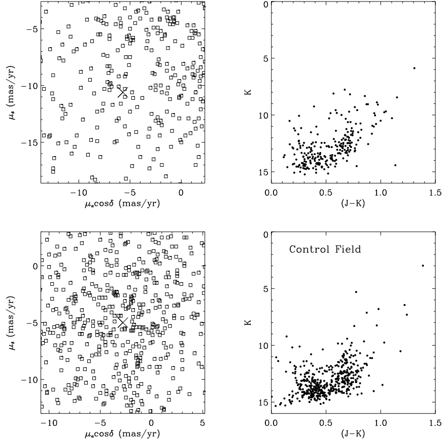
Figura 3.14: Identificação de aglomerados abertos a partir da análise do VPD e do CMD. Os dados cinemáticos e fotométricos em JHKs foram fornecidos pelo UCAC3. Diagrama superior à esquerda : Diagrama de movimentos próprios (VPD) para um campo de 20' \times 20' na região do aglomerado aberto ESO 137-23, obtido a partir dos dados de estrelas com movimentos próprios entre \bar{\mu}_{\alpha,\delta} \pm 8 \text{ msa ano}^{-1} , em que \bar{\mu}_{\alpha,\delta} é a moda para os movimentos próprios em \alpha e \delta , respectivamente. Diagrama superior à direita : Diagrama cor-magnitude (CMD) obtido a partir dos dados das estrelas no VPD, para o campo do aglomerado. Diagrama inferior à esquerda : O mesmo que o diagrama superior à esquerda, porém, para o campo de controle. Diagrama inferior à direita : O mesmo que o diagrama superior à direita, porém, para o campo de controle.
