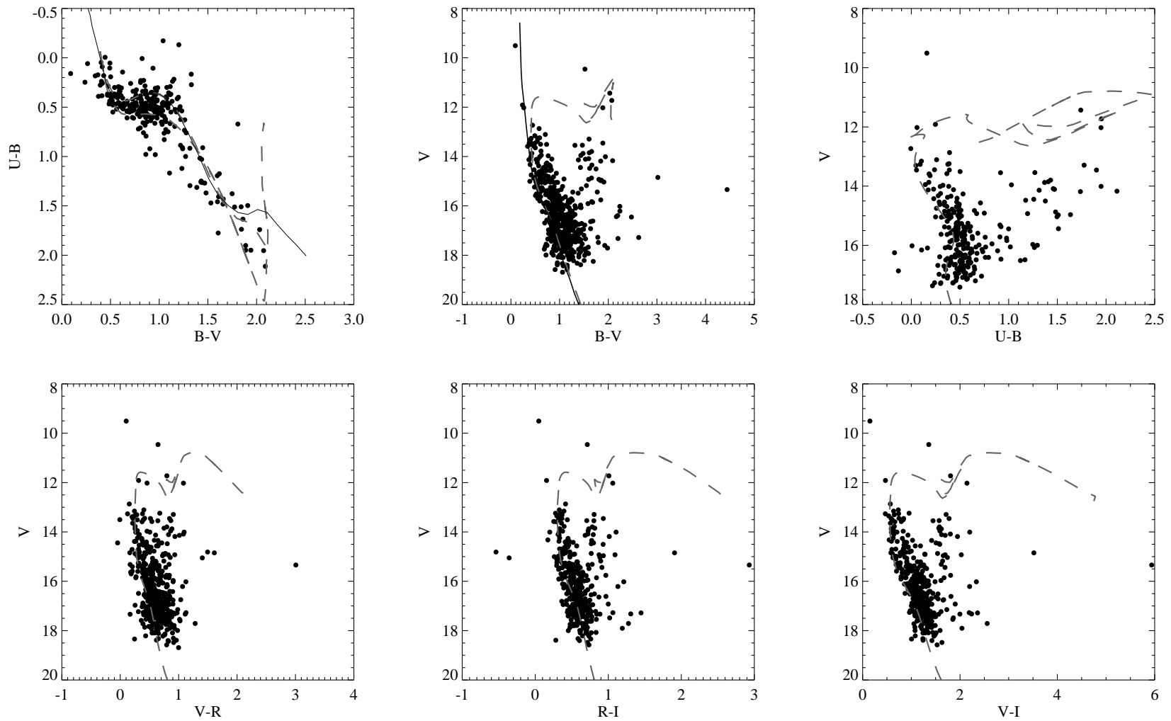
Figura 4.20: Diagramas fotométricos para Ruprecht 176. Os ajustes correspondem a E_{(B-V)} = 0.51 mag, d = 2740 pc e \log t = 8.20
