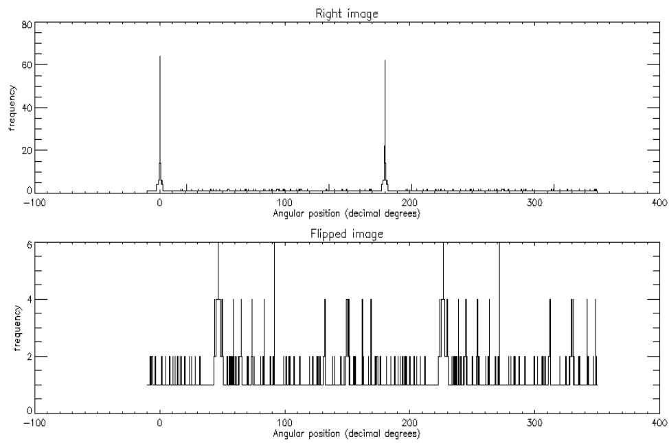
Figura 2.13: Histograma do número de elementos em W \cap V em função do ângulo \alpha , para o campo do aglomerado ESO 275-01, observado em 10 de maio.
