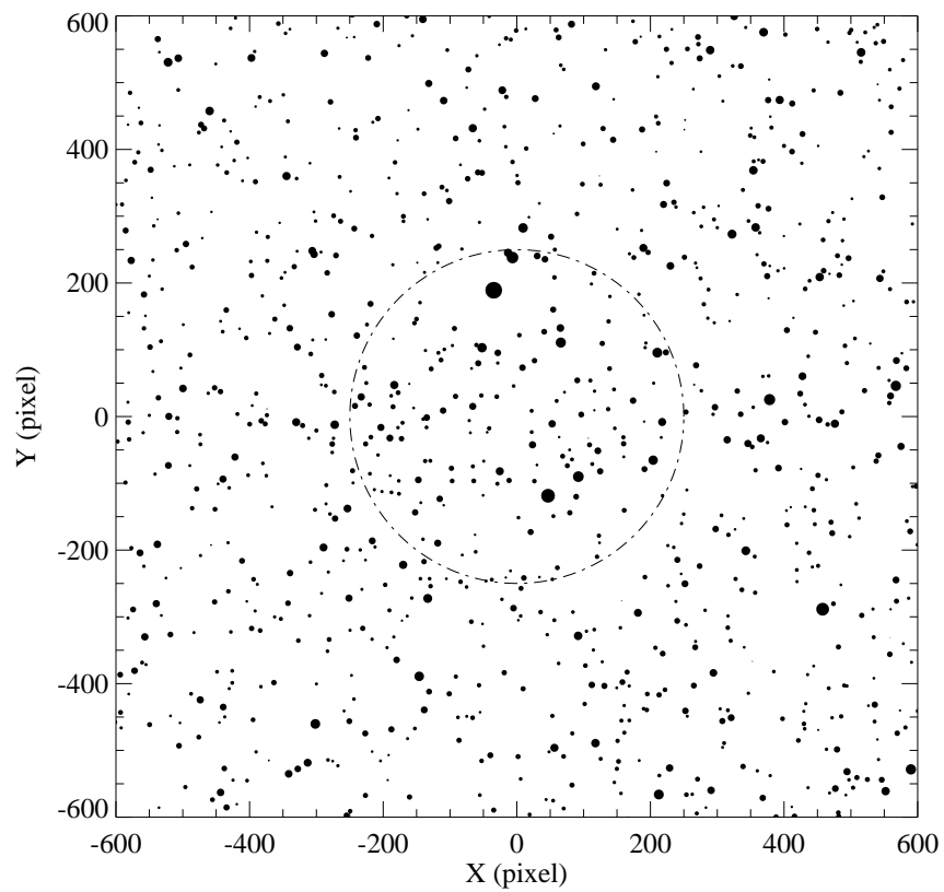
Figura 4.32: Mapa do campo do aglomerado Ruprecht 133 gerado a partir da lista de estrelas mostradas no CMD. O círculo tracejado indica a região do aglomerado. A escala de placa é igual a 0.600 segundos de arco por pixel. O leste aponta para cima e o norte aponta para a esquerda na figura.
