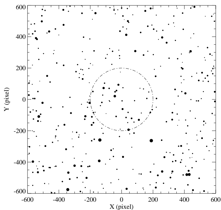
Figura 4.30: Mapa do campo do aglomerado Loden 1202, gerado a partir da lista de estrelas mostradas no CMD. O círculo tracejado indica a região do aglomerado. A escala de placa é igual a 0.600 segundos de arco por pixel. O leste aponta para cima e o norte aponta para a esquerda na figura.
