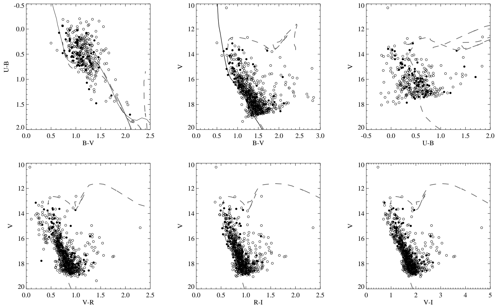
Figura 4.25: Diagramas fotométricos para ESO 134-12. Os ajustes correspondem a E_{(B-V)} = 0.83 mag, d = 2340 pc e \log t = 8.35
