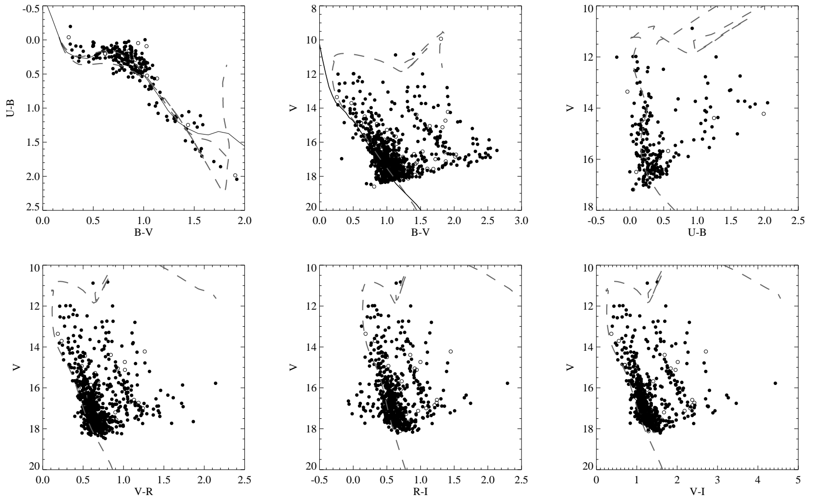
Figura 4.2: Diagramas fotométricos para o aglomerado Collinder 275. Os ajustes correspondem a E_{(B-V)} = 0.24 mag, d = 1920 pc e \log t = 8.45 anos.
