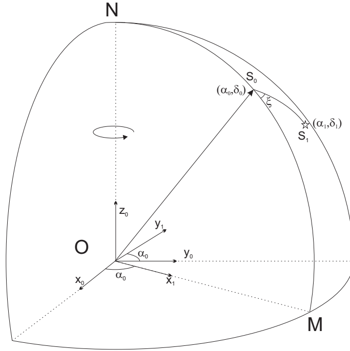
Figura 2.8: Rotação do sistema de referências em torno do eixo z . O ângulo de rotação é igual ao ângulo da ascensão reta do apontamento.
