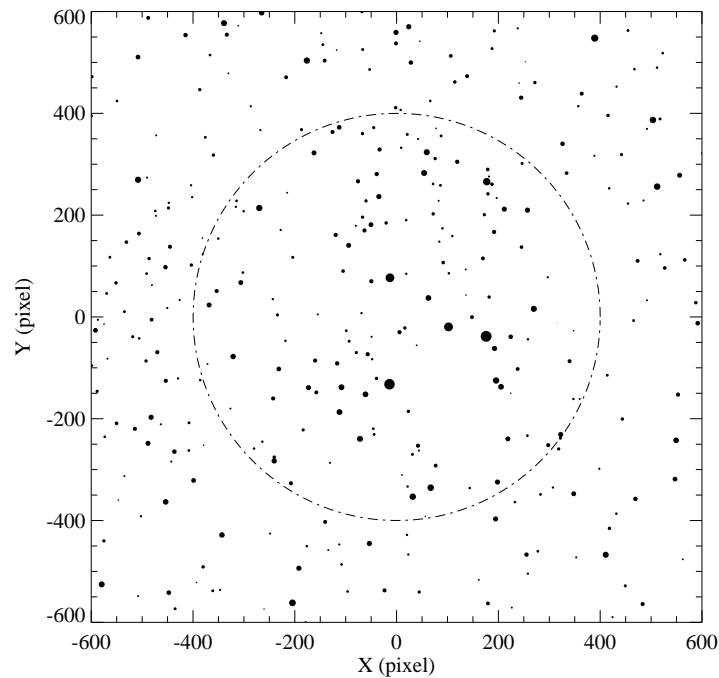
Figura 4.10: Mapa da região do aglomerado Ruprecht 170, gerado a partir dos dados das estrelas que aparecem no CMD. O círculo tracejado indica a região do aglomerado. A escala de placa é 0.600 segundos de arco por pixel, o leste aponta para cima e o norte aponta para a esquerda na figura.
