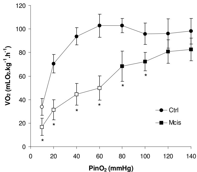
FIGURA 11. Efeito da redução gradual das tensões de oxigênio da água de entrada do respirômetro ( P_{in}O_2 – mmHg) sobre o consumo de oxigênio ( \dot{V}O_2 – mL O_2 \cdot kg^{-1} \cdot h^{-1} ) dos grupos controle, Ctrl ( n = 8 ) e exposto à microcistina, Mcis ( n = 8 ) de O. niloticus . Valores médios \pm 1 D.P. *: diferença significativa entre os grupos experimentais. Os símbolos vazios indicam diferenças significativas em relação à normóxia ( p < 0,05 ).
