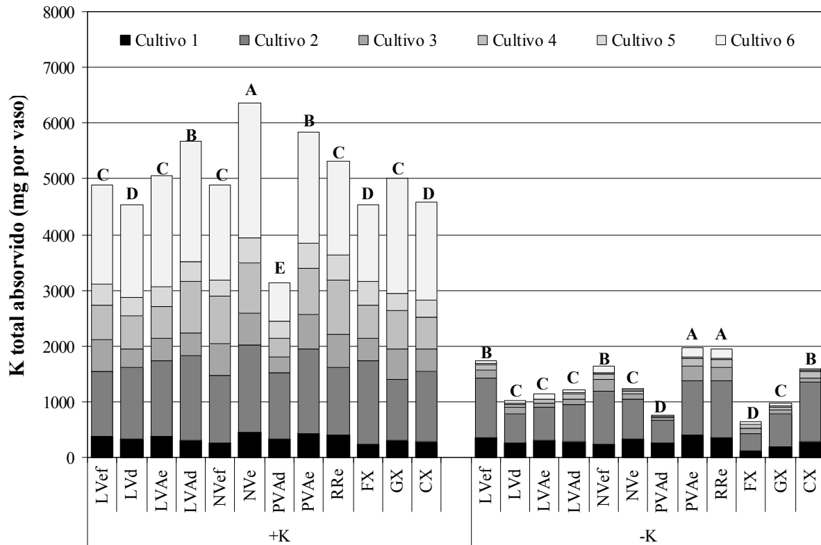
FIGURA 4. Potássio total absorvido em cada cultivo e acumulado na parte aérea das plantas nos diferentes solos coletados no Estado do Paraná com (+K) e sem (-K) fertilização potássica.
