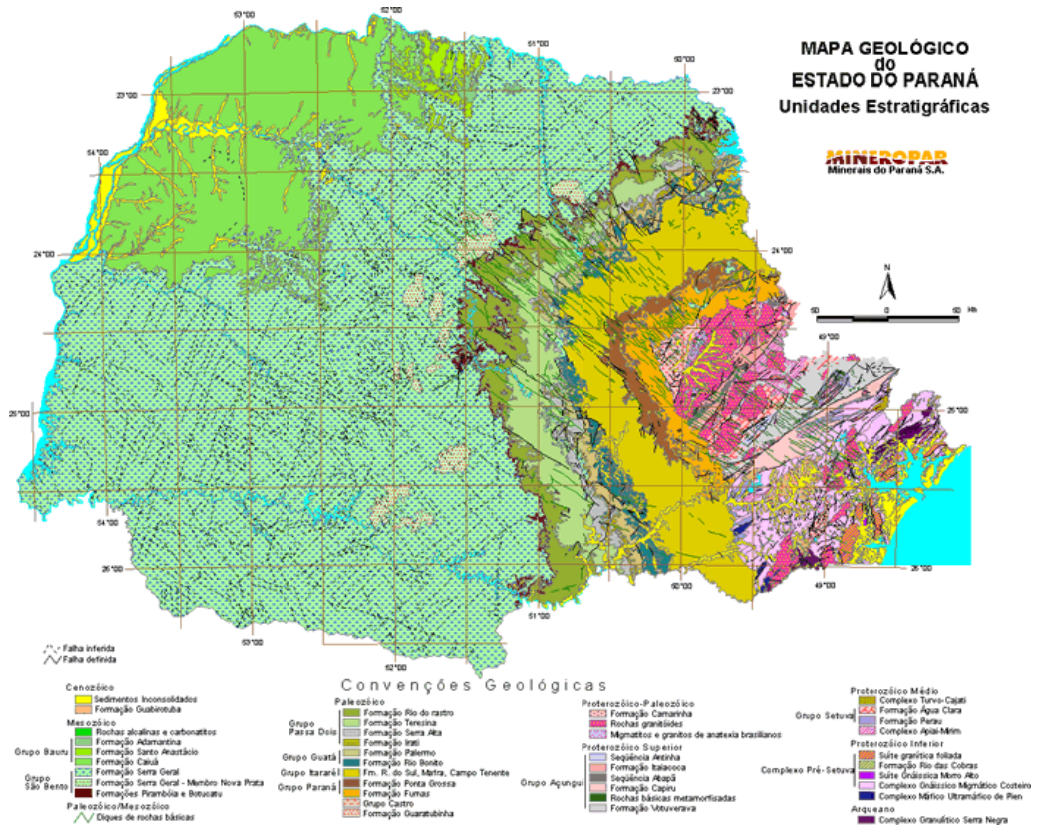
APÊNDICE 7. Mapa geológico do Estado do Paraná. Unidades estratigráficas. Fonte: MINEROPAR (2009).
