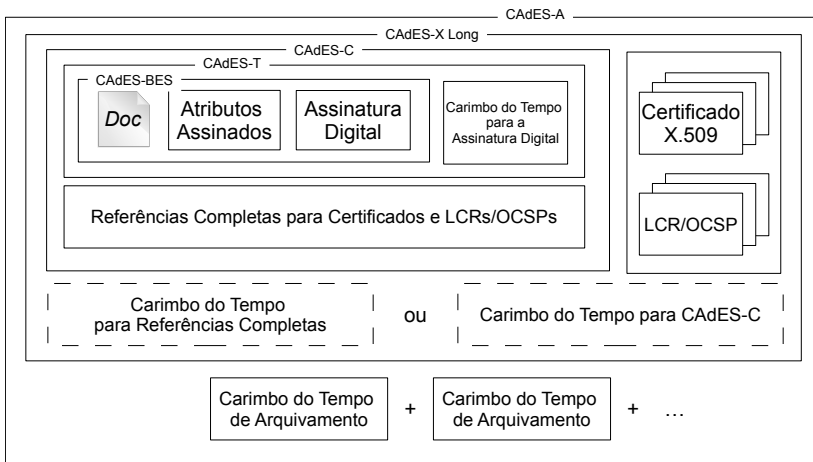
Figura 3.9: Perfil CADES-A.
