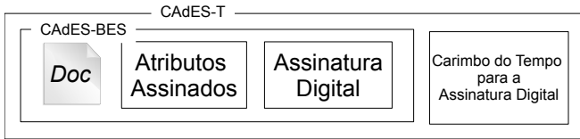
Figura 3.6: Perfil CAAdES-T.
