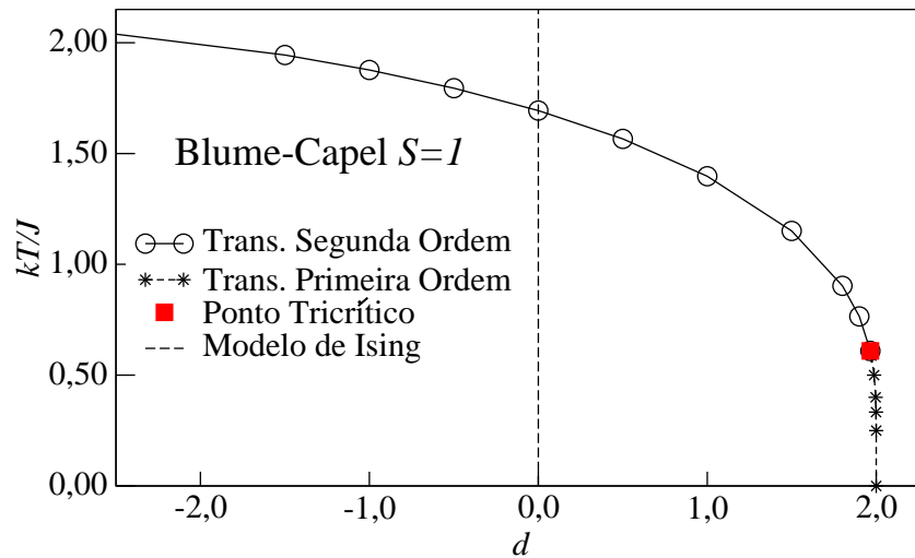
Figura 2.2: Diagrama de fases do modelo de Blume-Capel S = 1 , os dados foram retirados da ref. [40].
