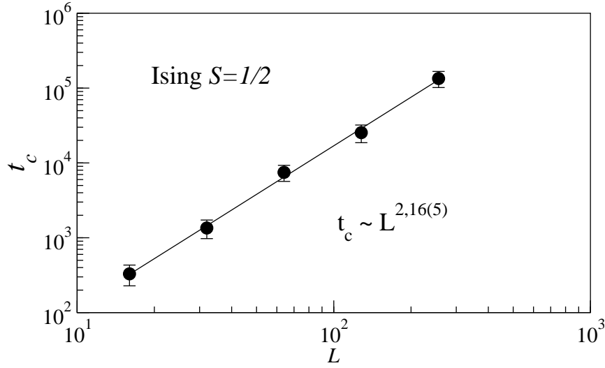
Figura 6.6: Tempo de relaxação t_c em função do tamanho da rede L para o modelo de Ising S=1/2 em T = T_c . Este gráfico foi feito para os seguintes tamanhos de rede ( L = 16, 32, 64, 128 e 256 ) e média sobre 1000 amostras.
