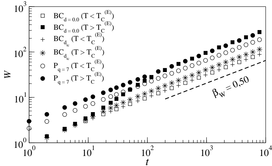
Figura 6.7: Rugosidade W em função do tempo t para o modelo de BC e Potts em T \neq T_c . Este gráfico foi feito para um tamanho de rede L = 64 . Foram feitas médias com 100 amostras.
