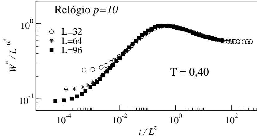
Figura 7.20: Colapso da rugosidade sem ruído W^* em função do tempo t para modelo de Relógio com p = 10 com vários tamanhos da rede L . z é o expoente dinâmico e \alpha^* e o expoente da rugosidade sem ruído. As médias foram feitas com M = 2000 amostras com um tempo de t = 2 \times 10^4 PMC.
