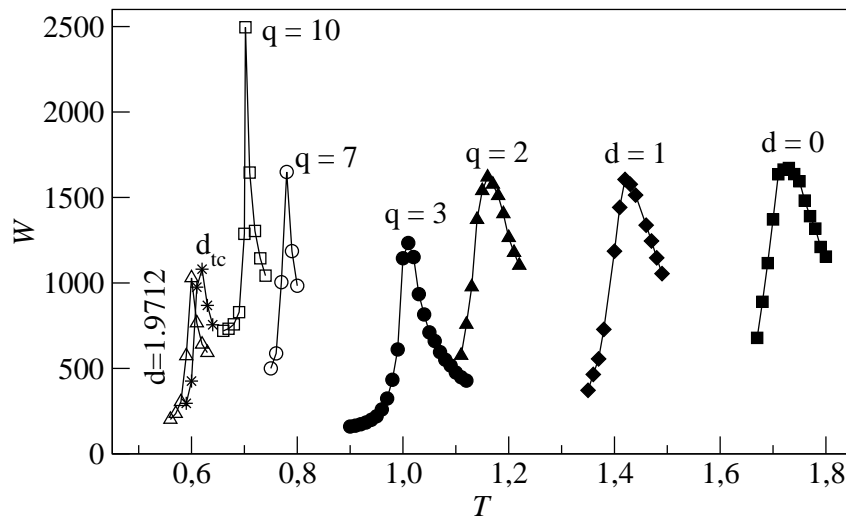
Figura 6.11: Rugosidade W em função da Temperatura T para o modelo de Blume-Capel S=1 ( d = 0, 1.0, 1.9655 e 1.9712 ) e Potts com q estados ( q = 2, 3, 7 e 10 ). O tempo esperado para o sistema termalizar foi t = 20000 PMC e as médias foram feitas sobre 200 amostras.
