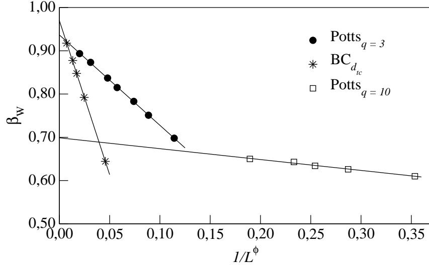
Figura 6.9: Expoente de crescimento \beta_W em função de 1/L^\phi para o modelo de Blume-Capel S = 1 ( d_{tc} ) e modelo de Potts ( q = 3 e q = 10 ) em T = T_c . Este gráfico foi feito para vários tamanhos de rede ( L=32, 48, 64, 128 e 256 ), as linhas são os valores da extrapolação ( L \rightarrow \infty ). Foram feitas médias com 1000 amostras em todos os tamanhos.
