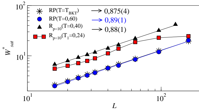
Figura 7.19: Comportamento do valor de saturação da rugosidade sem ruído W^* em função de vários tamanhos da rede L . As curvas mostradas são dos modelos de Relógio com p = 10 ( T = 0,24 e T = 0,40 ) e Rotor Planar ( T = 0,60 e T = T_{BKT} ). Os valores mostrados são dos expoentes da rugosidade sem ruído. As barras de erro são menores que o tamanho dos símbolos. As médias foram feitas com M = 100 - 2000 amostras com um tempo de t = 10^5 - 10^7 PMC .
