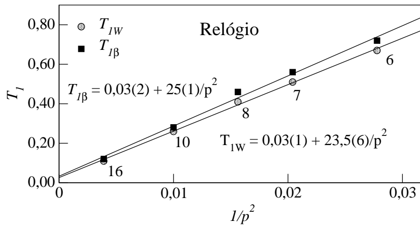
Figura 7.14: Temperatura de transição T_1 em função de 1/p^2 para o modelo de Relógio com p estados. As linhas contínuas são os ajustes dos pontos, as médias foram feitas com M = 2000 amostras com um tempo de t = 2 \times 10^4 PMC.
