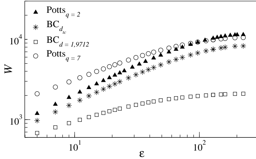
Figura 6.2: Comportamento da rugosidade com a escala \varepsilon para os modelos de Blume-Capel com spin S e Potts com q estados para q = 2 (segunda ordem), d = 1.9655 (ponto tricrítico) e d = 1.9712 e q = 7 (primeira ordem). Este gráfico foi feito para um tamanho típico de rede ( L = 224 ). Foram feitas médias com 100 amostras .
