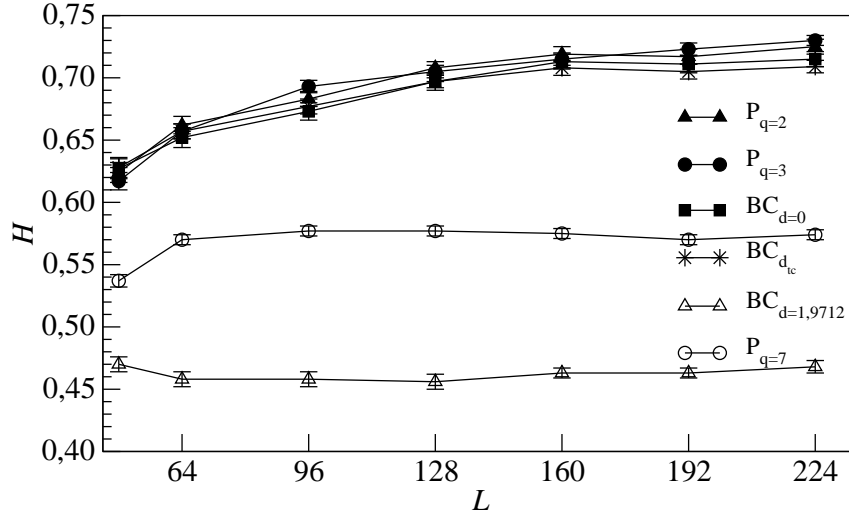
Figura 6.3: Expoente de Hurst H em função do tamanho da rede L para o modelo de Potts com q estados e Blume-Capel spin- S . A menor rede corresponde a L = 48 . Foram feitas médias com 100 amostras.
