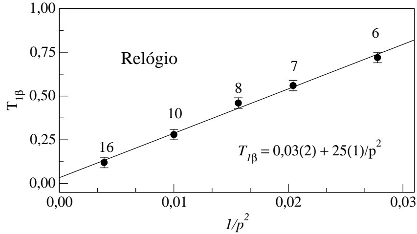
Figura 7.11: Temperatura de transição T_1 em função de 1/p^2 para o modelo de Relógio com p estados em uma rede de tamanho L = 32 . A linha contínua é o ajuste linear dos pontos e as médias foram feitas com M = 10^4 amostras com um tempo de t = 200 PMC.
