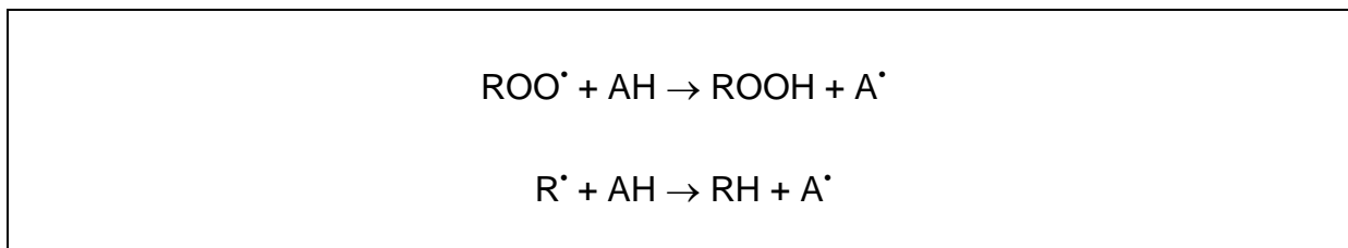
Figura 12: Mecanismo de ação para antioxidantes primários. Onde: \text{ROO}^\bullet e \text{R}^\bullet são radicais livres, \text{AH} é o antioxidante com um hidrogênio ativo e \text{A}^\bullet é radical inerte.
