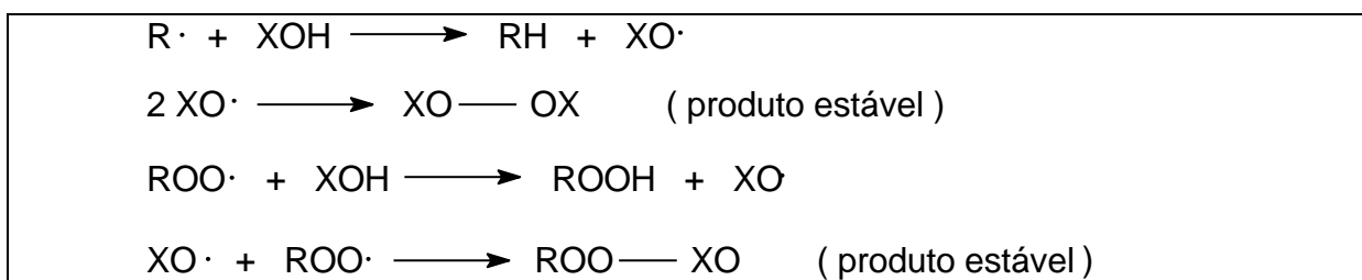
Figura 7: Ilustração do mecanismo de atuação do aditivo antioxidante (XOH) na supressão de radicais livres (R·, XO·, ROO·) e conseqüente retardamento do envelhecimento do OMI.
