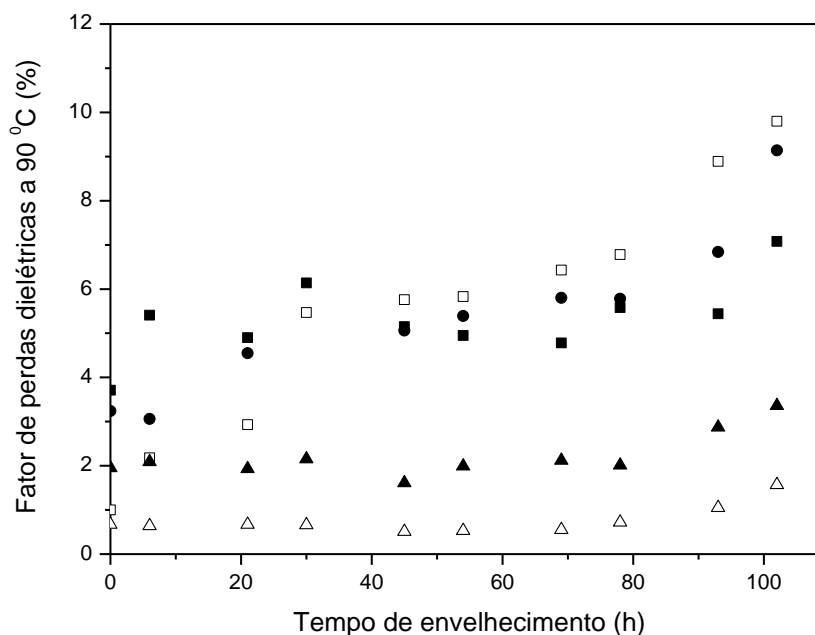
Figura 19: Efeito do envelhecimento acelerado dos óleos não-aditivados sobre o fator de perdas dielétricas a 90 °C: (■) OV-1; (▲) OV-2; (●) OV-3; (□) OVI-A e (Δ) OVI-B.
