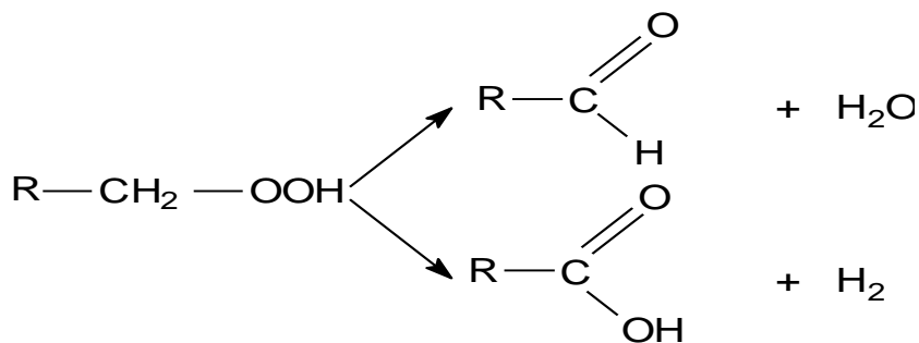
Figura 5: Produtos de oxidação do OMI.
