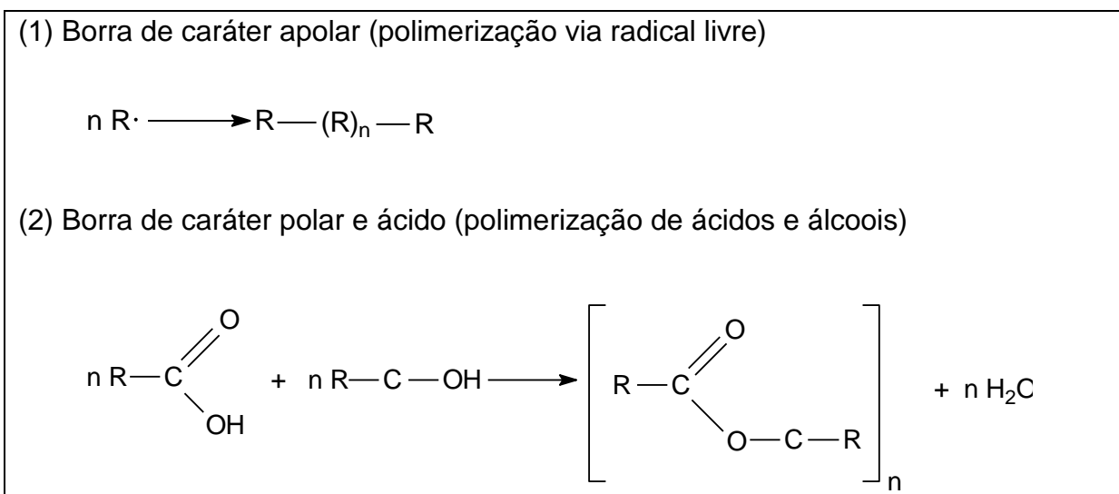
Figura 6: Esquema ilustrativo das reações de formação da borra, a partir dos compostos de oxidação do OMI.
