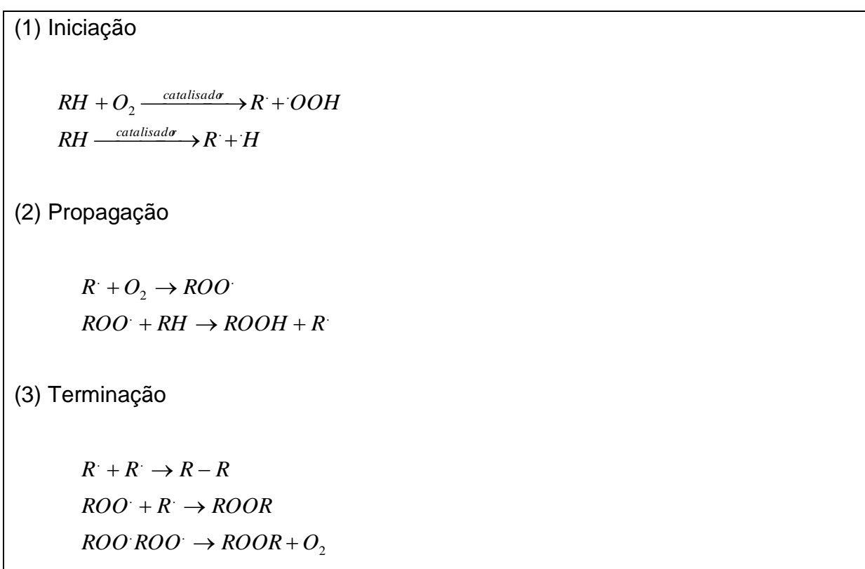
Figura 10: Etapas do processo de autoxidação de óleos insaturados.
