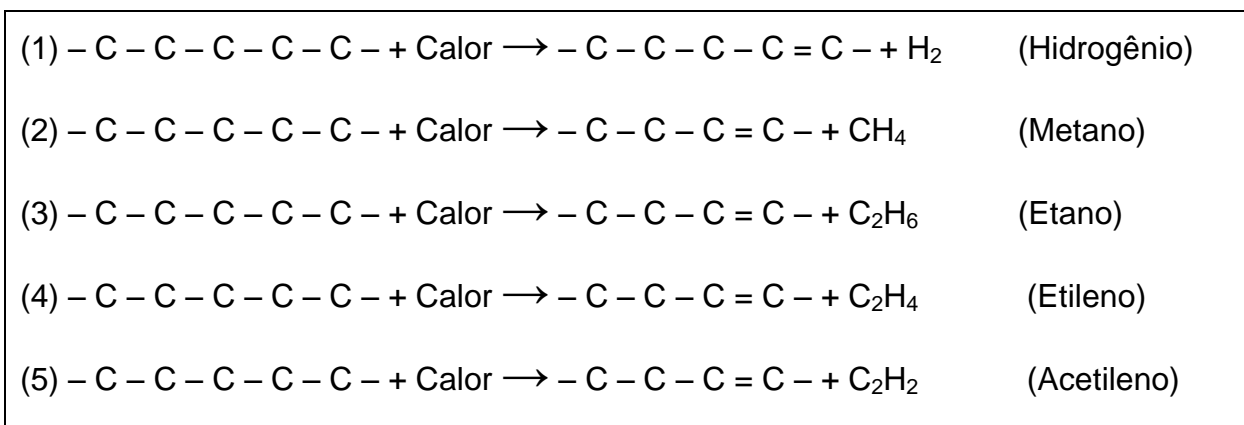
Figura 8: Reações de Pirólise do OMI.
