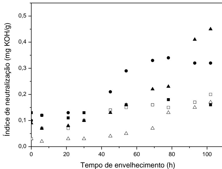
Figura 17: Efeito do envelhecimento acelerado dos óleos não-aditivados sobre o índice de neutralização: (■) OV-1; (▲) OV-2; (●) OV-3; (□) OVI-A e (△) OVI-B.
