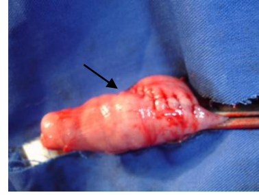
Figura 14- Sutura Termino-lateral
