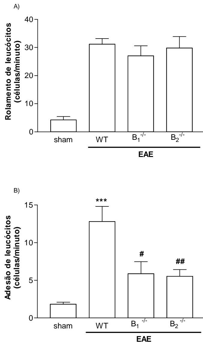
Figura 25. Análise in vivo do recrutamento de leucócitos na microvasculatura cerebral de animais knockout para os receptores B 1 e B 2 da bradicinina. A análise foi realizada, utilizando a técnica de microscopia intravital, através da contagem do número de leucócitos em rolamento (A) e aderidos (B) na parede dos vasos da pia-máter dos animais (n=6/ grupo), no 14º dia após a indução. Os resultados foram expressos como n° de células/minuto (media ± EPM), e análise estatística foi realizada pelo teste não-paramétrico ANOVA, indicando: ***P < 0,001 para os diferentes grupos comparados ao grupo sham e ##P < 0,01 para os grupos knockout comparados com os animais WT.
