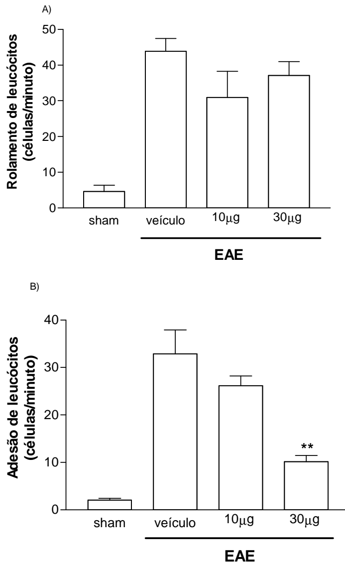
Figura 20. Efeito da proteína mutante P8A sobre o recrutamento de leucócitos na microvasculatura cerebral de animais com EAE. No 14 o dia após a imunização com MOG 35-55, camundongos EAE (n=6/grupo) foram tratados com 10µg e 30µg i.p de P8A uma hora antes do procedimento de microscopia intravital. Foram avaliados in vivo os eventos de rolamento (A) e adesão (B) de leucócitos nos vasos da pia-máter. E, os resultados foram expressos em número de células/minuto (média ± EPM). A análise estatística foi realizada pelo teste ANOVA não-paramétrico, indicando *P < 0,05 em comparação com o grupo EAE tratado com PBS.
