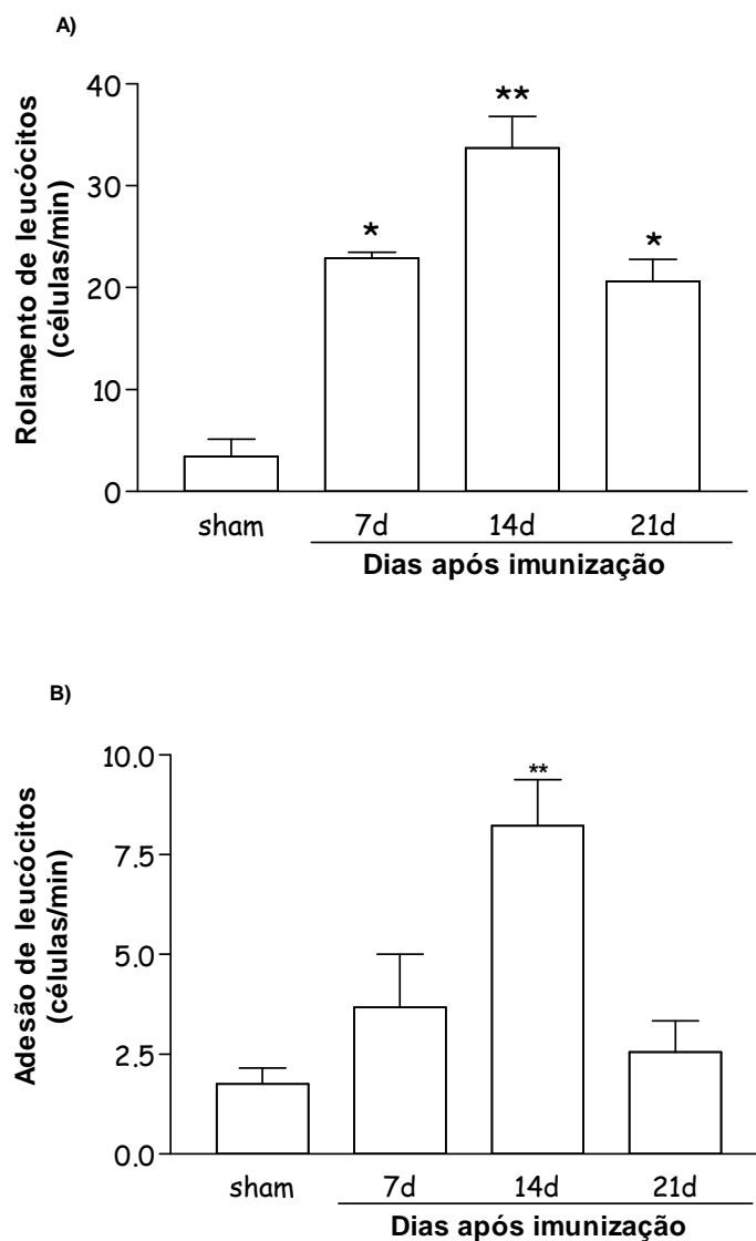
Figura 14. Análise in vivo do recrutamento de leucócitos na microvasculatura cerebral de camundongo com EAE. A análise foi realizada, utilizando a técnica de microscopia intravital, que permitiu a contagem do número de leucócitos em rolamento (A) e aderidos na parede dos vasos (B) da pia-máter dos animais (n=7/grupo). O estudo ocorreu nos dias 7, 14 e 21 após a imunização. Os resultados foram expressos como n° de células/minuto (media \pm EPM), e o teste não-paramétrico ANOVA indicou: ***P < 0,001 em relação ao grupo controle.
