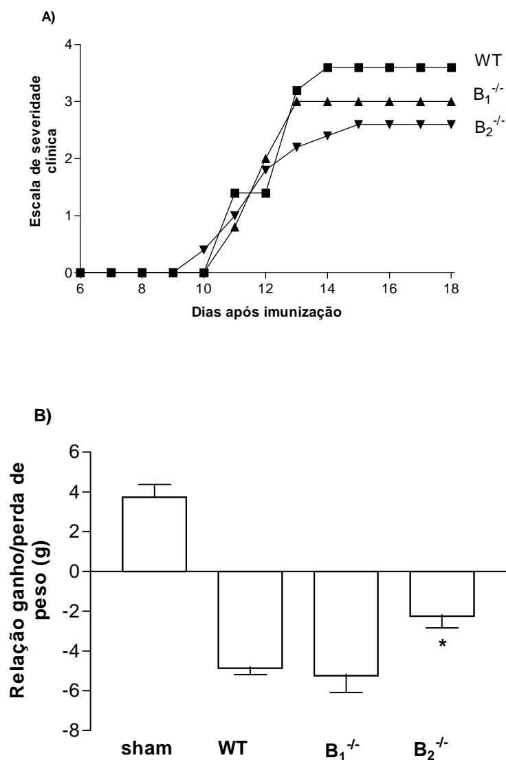
Figura 23. Avaliação do perfil clínico do modelo de EAE em animais knockout para os receptores B 1 e B 2 da bradicinina. Camundongos C57BL/6 X sv129 B 1 -/- , B 2 -/- e WT com EAE (n=7/grupo) foram avaliados durante 22 dias, após a indução com peptídeo MOG 35-55, quanto aos sinais clínicos da doença (A) e quanto à perda de peso corporal (B). Os resultados referentes ao perfil clínico foram expressos baseados numa escala de severidade clínica, previamente descrita (média ± EPM) e, quanto ao peso foi indicada perda e ganho em gramas por grupo (média ± EPM). O teste One-Way ANOVA foi utilizado, indicando *P < 0,05 para o grupo B 2 -/- , comparando com o grupo WT (A e B).
