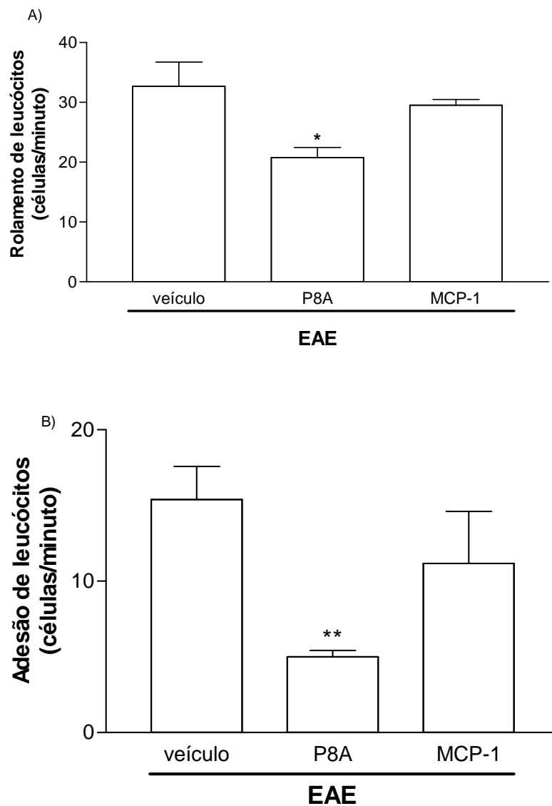
Figura 21. Avaliação in vivo do recrutamento de leucócitos na microvasculatura cerebral de camundongos com EAE a partir do tratamento com CCL2/MCP-1 e P8A. Os animais foram tratados com P8A (T1) e CCL2 (T2), 30µg/dia i.p., 1 hora antes do procedimento de microscopia intravital. Foram avaliados os eventos de rolamento (A) e adesão celular (B) nos vasos da pia-máter. Os resultados foram expressos em no de células/minuto (média ± EPM) e o teste One-Way ANOVA foi utilizado para análise estatística, indicando **P < 0,01 em comparação com o grupo que recebeu o mesmo volume de PBS 1X.
