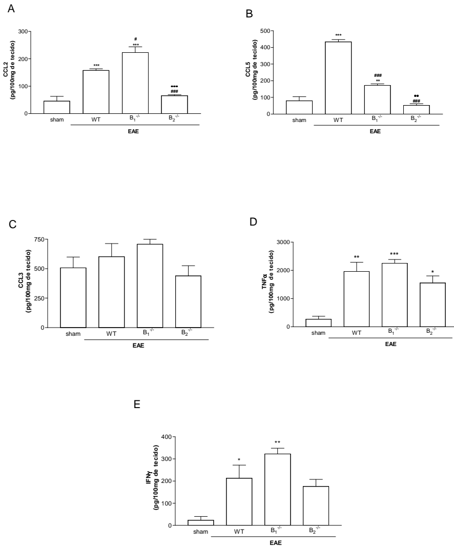
Figura 27. Avaliação do papel dos receptores B 1 e B 2 da bradicinina na regulação da produção de citocinas e quimiocinas no modelo EAE. A produção de citocinas e quimiocinas foi avaliada em homogenato de cérebro de animais EAE WT, B 1 -/- , B 2 -/- e controle (n=6/grupo). As amostras foram referentes ao dia 14 após indução da doença. Os níveis de CCL2 (A), CCL5 (B), CCL3 (C), TNFα (D) and IFNγ (E) foram medidos pelo método de ELISA. Os resultados foram expressos em pg/100mg de tecido (média ± EPM) e o teste One-way ANOVA foi utilizado para análise de significância, indicando: *P<0.05, comparando com o grupo sham; #P<0.05 em relação ao grupo WT e *P<0.05 em relação ao grupo B 1 -/- .
