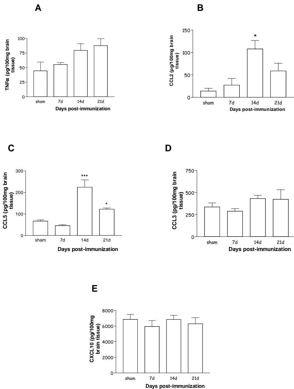
Figura 15. Avaliação da produção de citocinas e quimiocinas no cérebro de camundongos com EAE. Foram incluídos animais com EAE e animais controle (n=5). Os níveis de citocinas e quimiocinas foram medidos em amostras de homogenato de cérebro referentes aos dias 7, 14 e 21 após a imunização, utilizando o método de ELISA para a medida de TNF \alpha (A), CCL2 (B), CCL5 (C), CCL3 (D) e CXCL10 (E). Os resultados foram expressos em pg/100mg de tecido (média \pm EPM). A análise estatística foi feita pelo teste não-paramétrico ANOVA, considerando significativo P<0,05.
