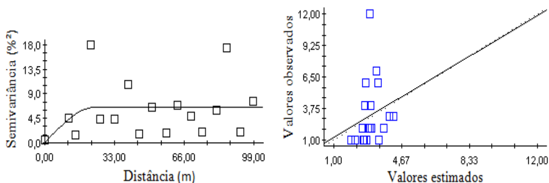
Figura 27. Semivariograma do manganês, na profundidade de 20-40cm, no qual o eixo dos x corresponde a distância (m) e no eixo dos y estão os valores de semivariância (%²). Gráfico de validação do semivariograma.
