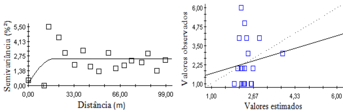
Figura 28. Semivariograma do zinco, na profundidade de 20-40cm, no qual o eixo dos x corresponde a distância (m) e no eixo dos y estão os valores de semivariância (%²). Gráfico de validação do semivariograma.
