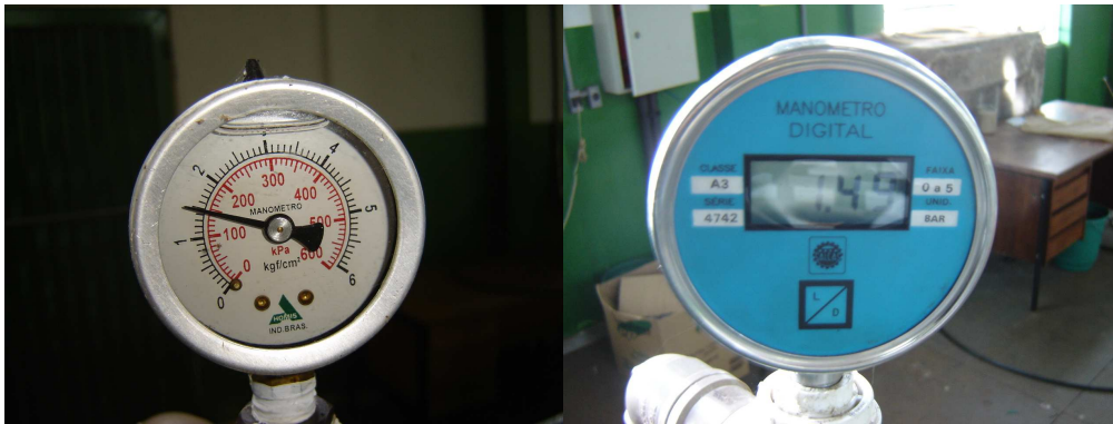
Figura 4 – Vista geral dos manômetros (analógico e digital).
