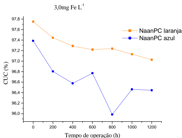
Figura 8 - Valores médios de CUC, para os tubo gotejadores NaanPC Laranja e NaanPC Azul, em função do tempo de operação, na dose de 3,0 \text{ mg L}^{-1} de ferro total.
