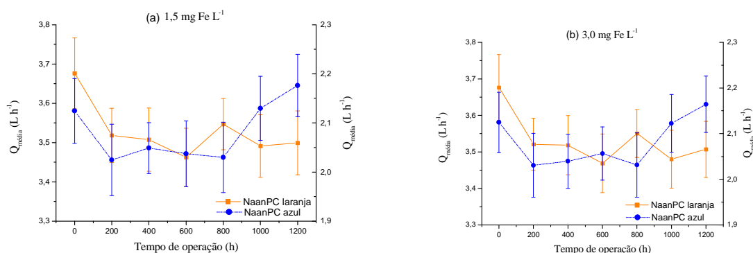
Figura 24 – Comparativo da variao da vazo dos tubo gotejadores NaanPC Azul e NaanPC Laranja, e seus respectivos desvios em funo do tempo de operao, na doses de 1,5 \text{ mg L}^{-1} (a) e 3,0 \text{ mg L}^{-1} (b) de ferro total.
