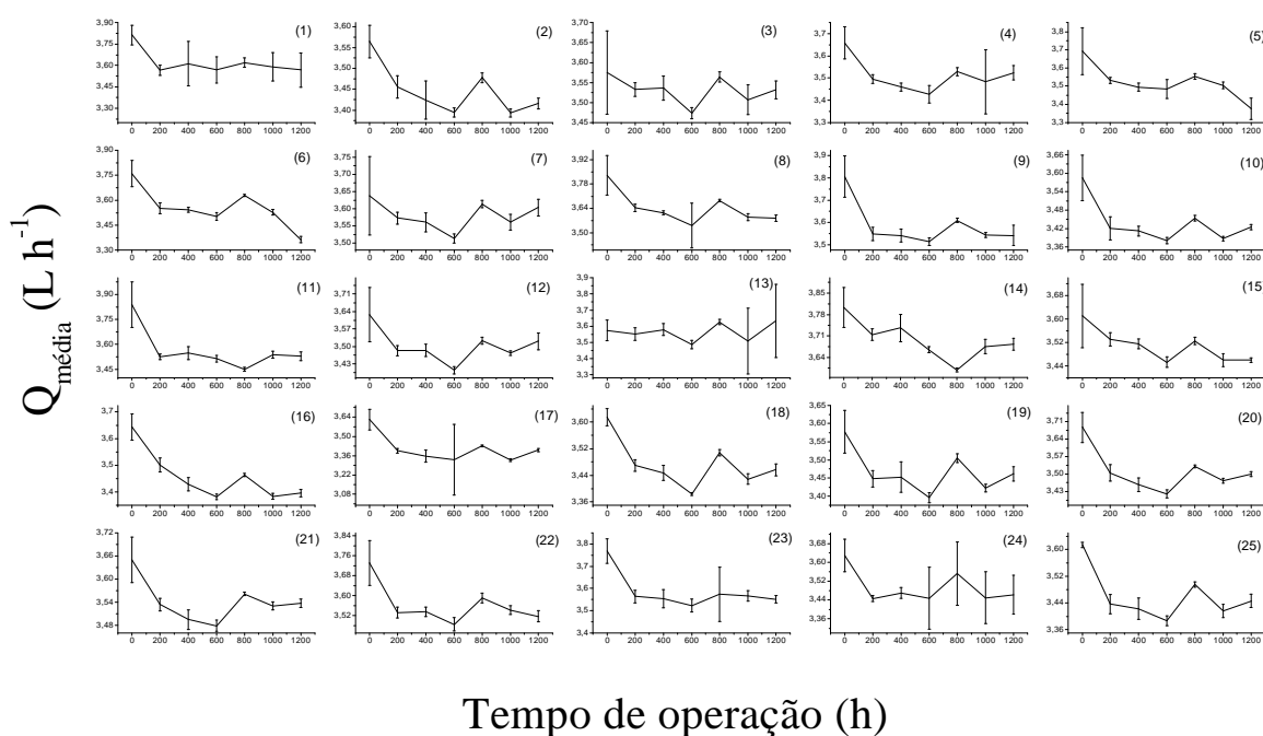
Figura 15 – Valores médios de vazão dos emissores do tubo gotejador NaanPC Laranja, e seus respectivos desvios em função do tempo de operação, na dose de 1,5 \text{ mg L}^{-1} de ferro total.
