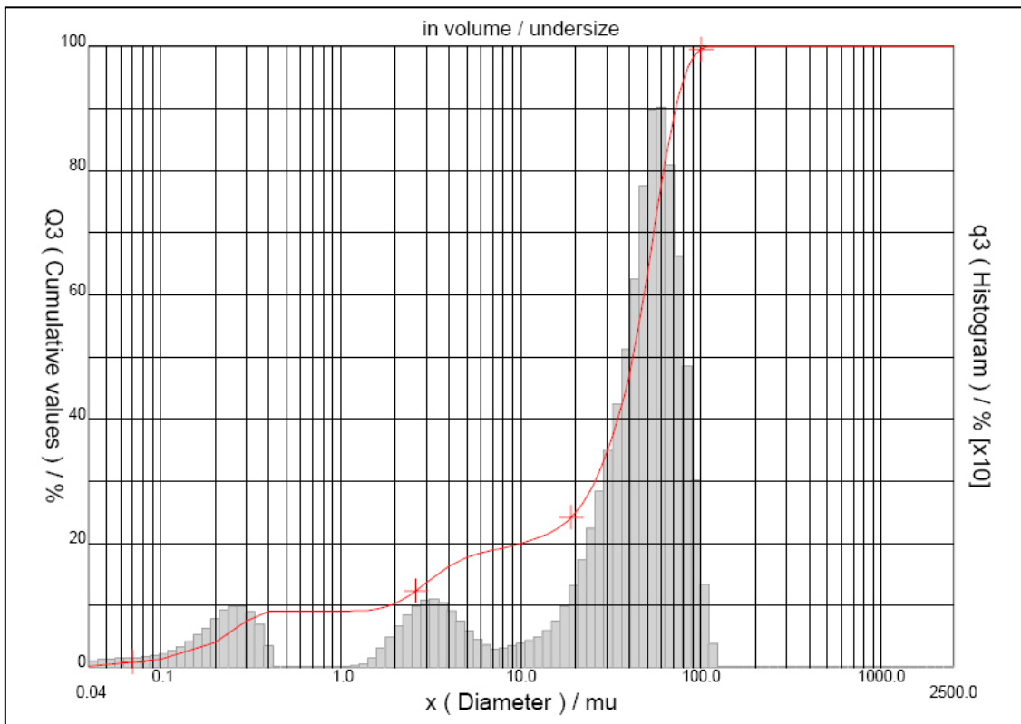
Figura 31. Análise granulométrica do PMMA
