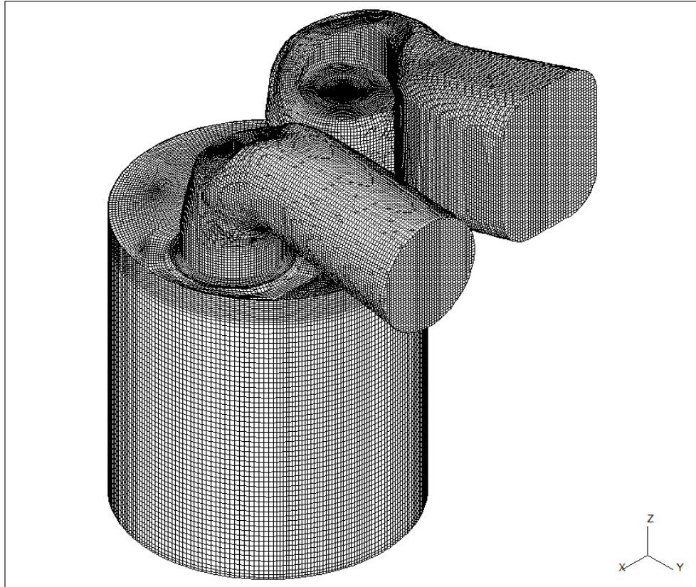
Figura 5.12 - Vista isométrica
