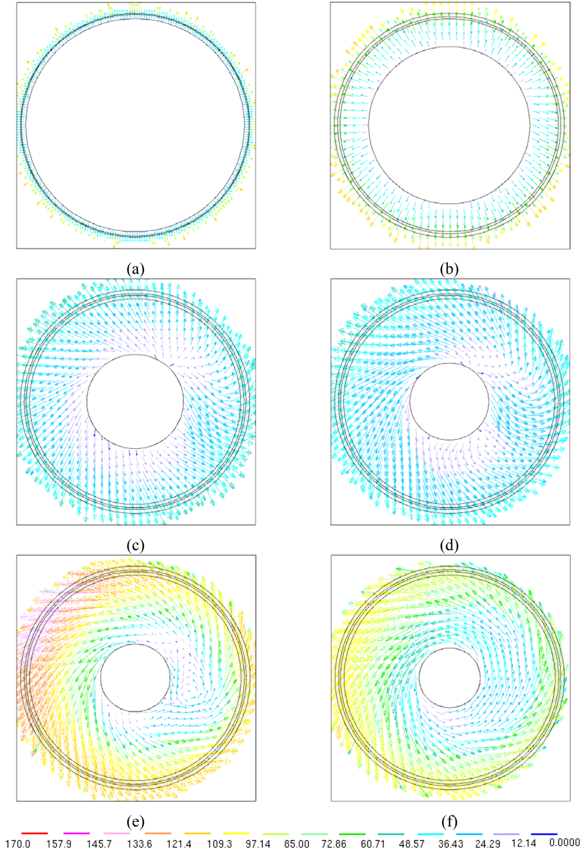
Figura A.6 - Campo de velocidades no corte C-C: (a) em 1080°; (b) 1095°; (c) 1115°; (d) 1130°; (e) 1145°; (f) 1206°
