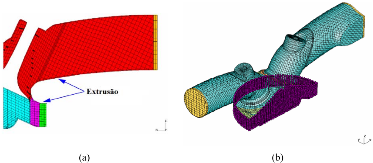
Figura 5.10 - Malha trimmed : (a) extrusão; (b) montagem final [Star-cd Tutorial es-ice, 2008]
