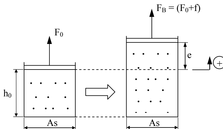
Figura 7: Desenho esquemático da definição da pressão interna do bolsão.
