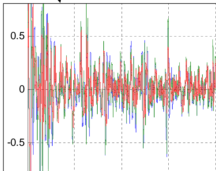
Gráfico 5: Força dinâmica no pneu traseiro para a velocidade de 80 km/h
