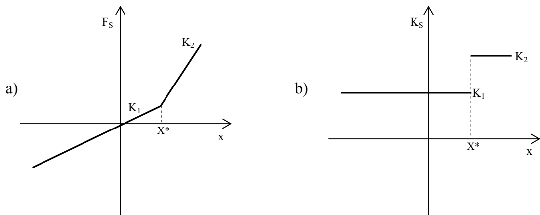
Figura 5: Gráfico característico de suspensão com 2 feixes de molas. a) Gráfico Força x Deformação. b) Gráfico Rigidez x Deformação.
