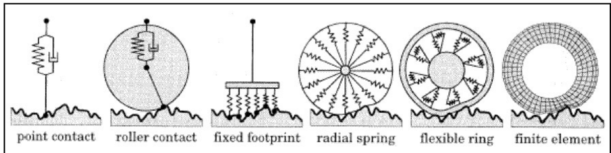
Figura 11: Modelos matemáticos de pneu. Fonte: Kistein, 2005, p. 8
