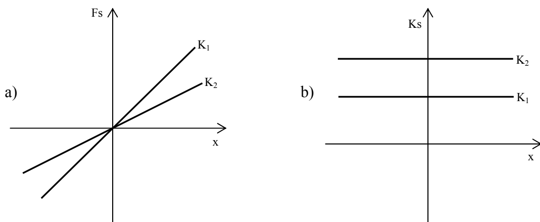
Figura 3: Gráfico característico da mola linear. a) Gráfico Força x Deformação. b) Gráfico Rigidez x Deformação.
