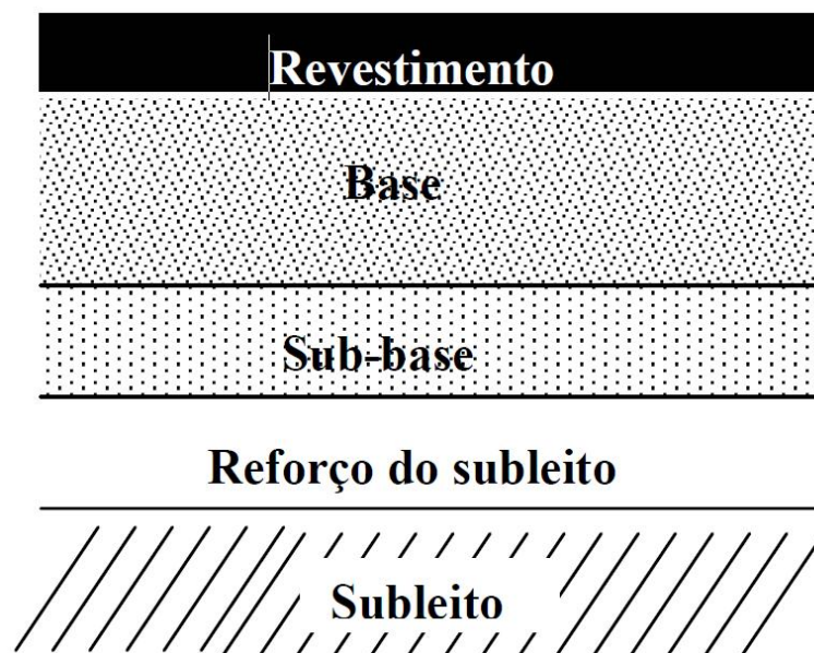
Figura 17: Seção típica de uma estrutura de pavimento flexível para subleito de baixa capacidade.
