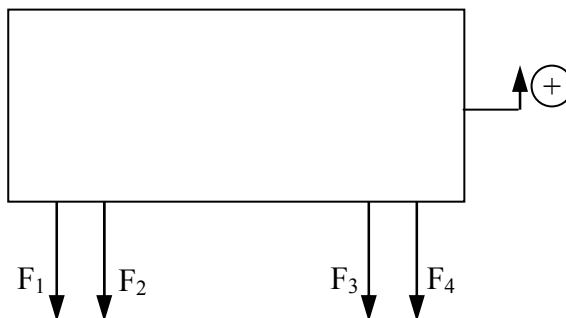
Figura 14: Diagrama de corpo livre da massa suspensa.
