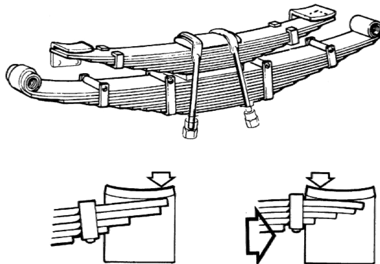
Figura 4: Esquema de suspensão metálica com dois feixes de molas.
