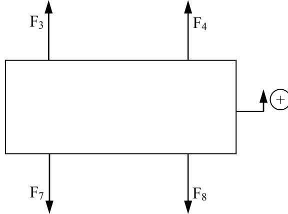
Figura 16: Diagrama de corpo livre da massa não suspensa traseira.
