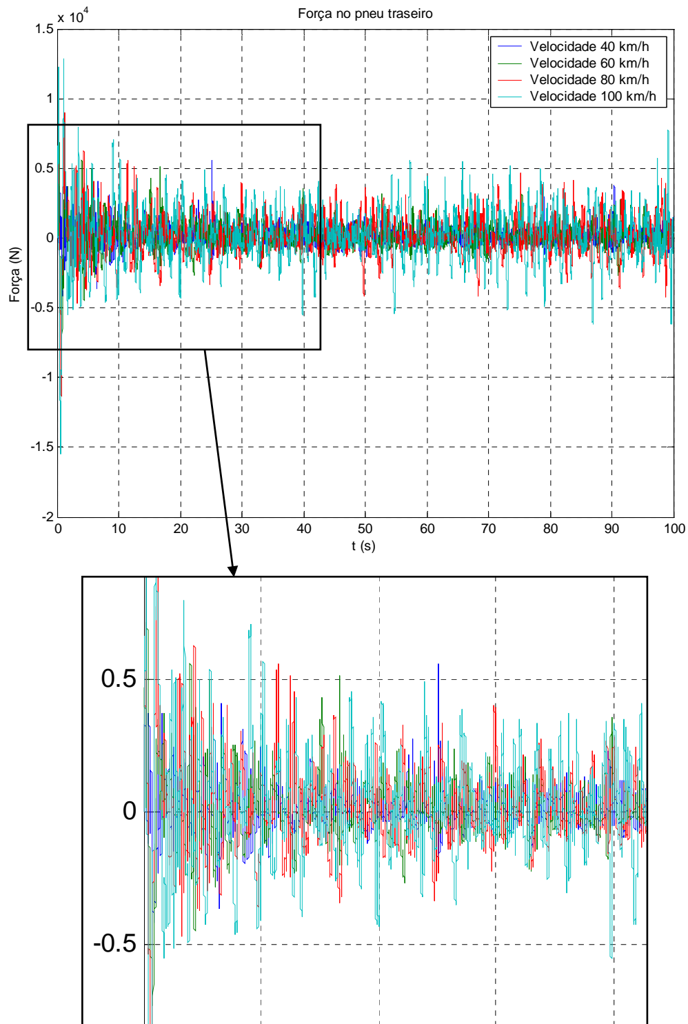
Gráfico 3: Força dinâmica no pneu traseiro para o modelo 3
