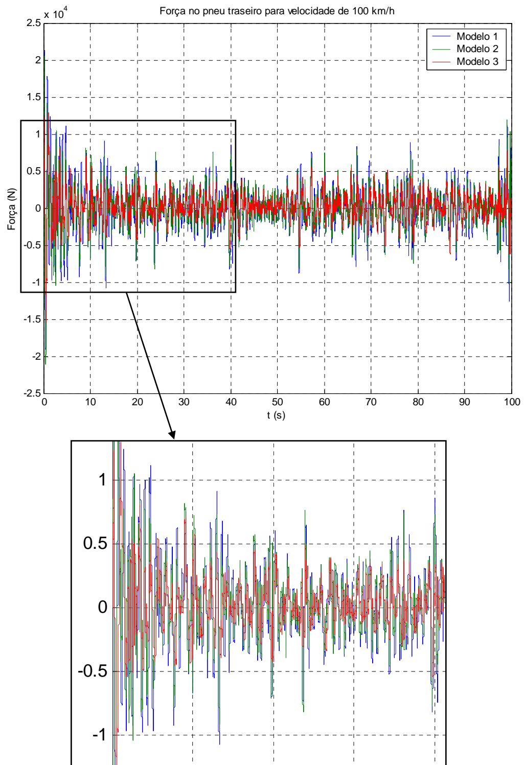
Gráfico 6: Força dinâmica no pneu traseiro para a velocidade de 100 km/h
