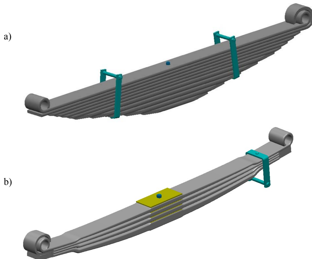
Figura 2: Molas metálicas com feixe de lâminas. a) Conjunto com feixe de lâminas trapezoidais. b) Conjunto com feixe de lâminas parabólicas.
