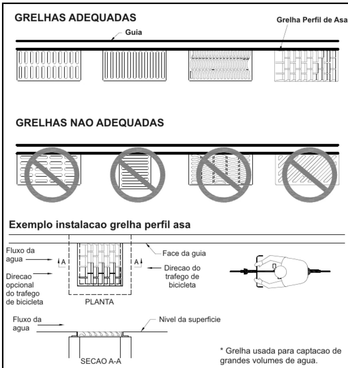
Figura 7.6: Esquemático de grelhas.
