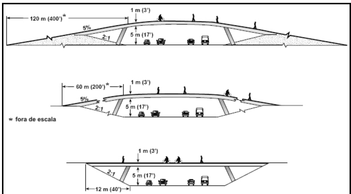
Figura 7.11: Esquemático de passarelas.
