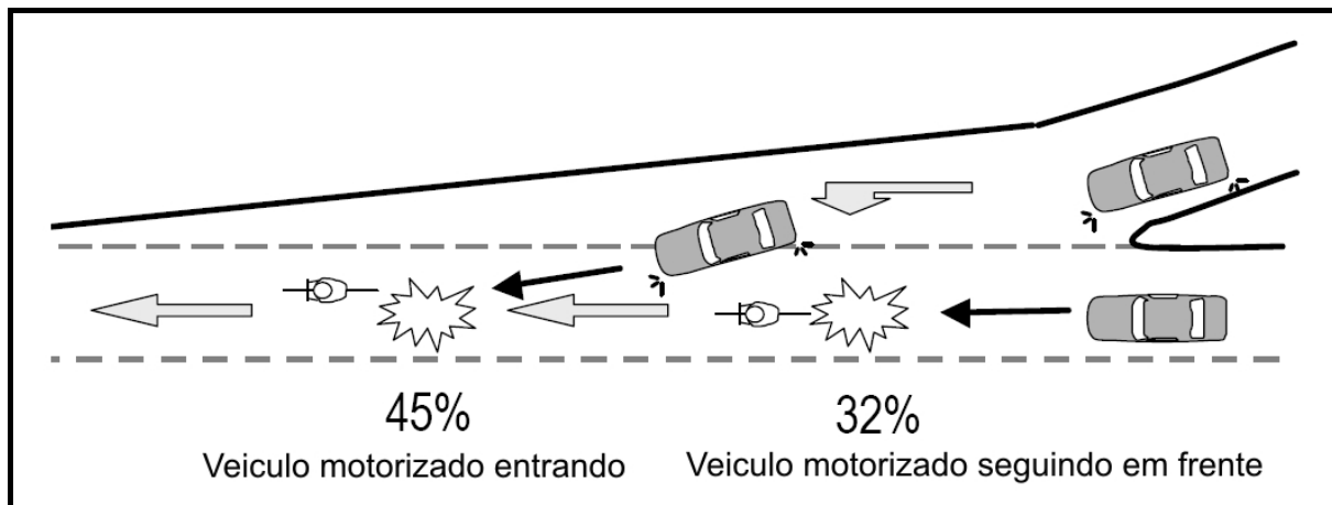
Figura 6.39: Esquemático de acidentes em entrada de via arterial.
