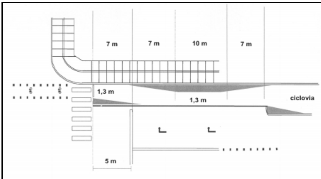
Figura 6.6: Esquemático de interrupção de ciclovia em área de aproximação de interseção.
