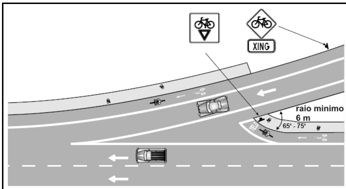
Figura 6.40: Esquemático de interseção em entrada de via expressa.
