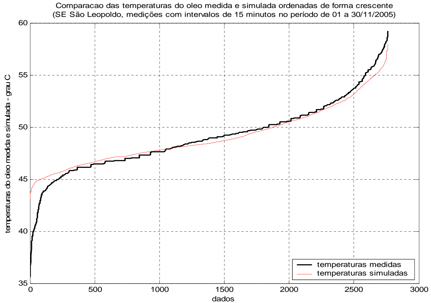
Figura 5.20 – Gráfico comparativo das temperaturas do óleo medidas e simuladas ordenadas de forma crescente. Dados da Subestação São Leopoldo referentes a medições com intervalo de 15 minutos do período de 01 a 30/09/2005.
