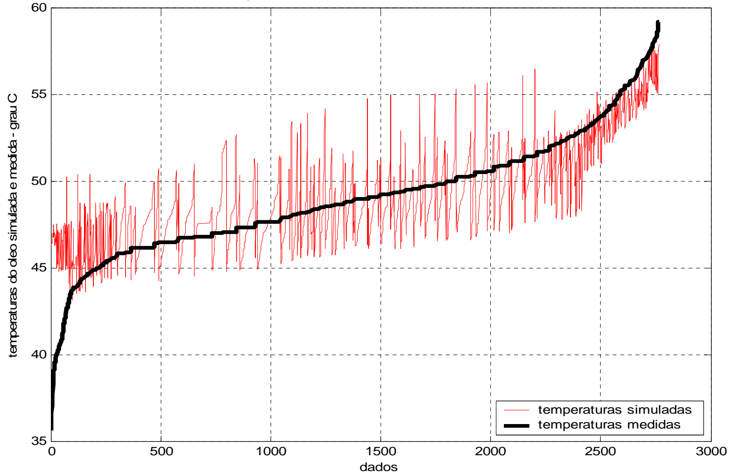
Dispersão da temperatura do óleo simulada comparativamente a temperatura do óleo medida e ordenada na forma crescente (SE São Leopoldo, medições com intervalos de 15 minutos no período de 01 a 30/09/2005)
