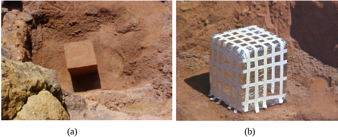
Figura IV.2 – Moldagem do bloco (a); Preparação do bloco para parafinação (b).
