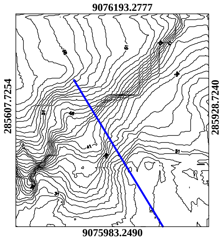
Figura III.17 – Localização do perfil topográfico – Ponto P-02 – encosta sul
