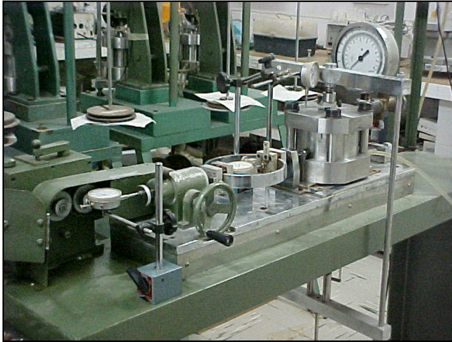
Figura IV.13 – Ensaio de cisalhamento direto com sucção controlada
