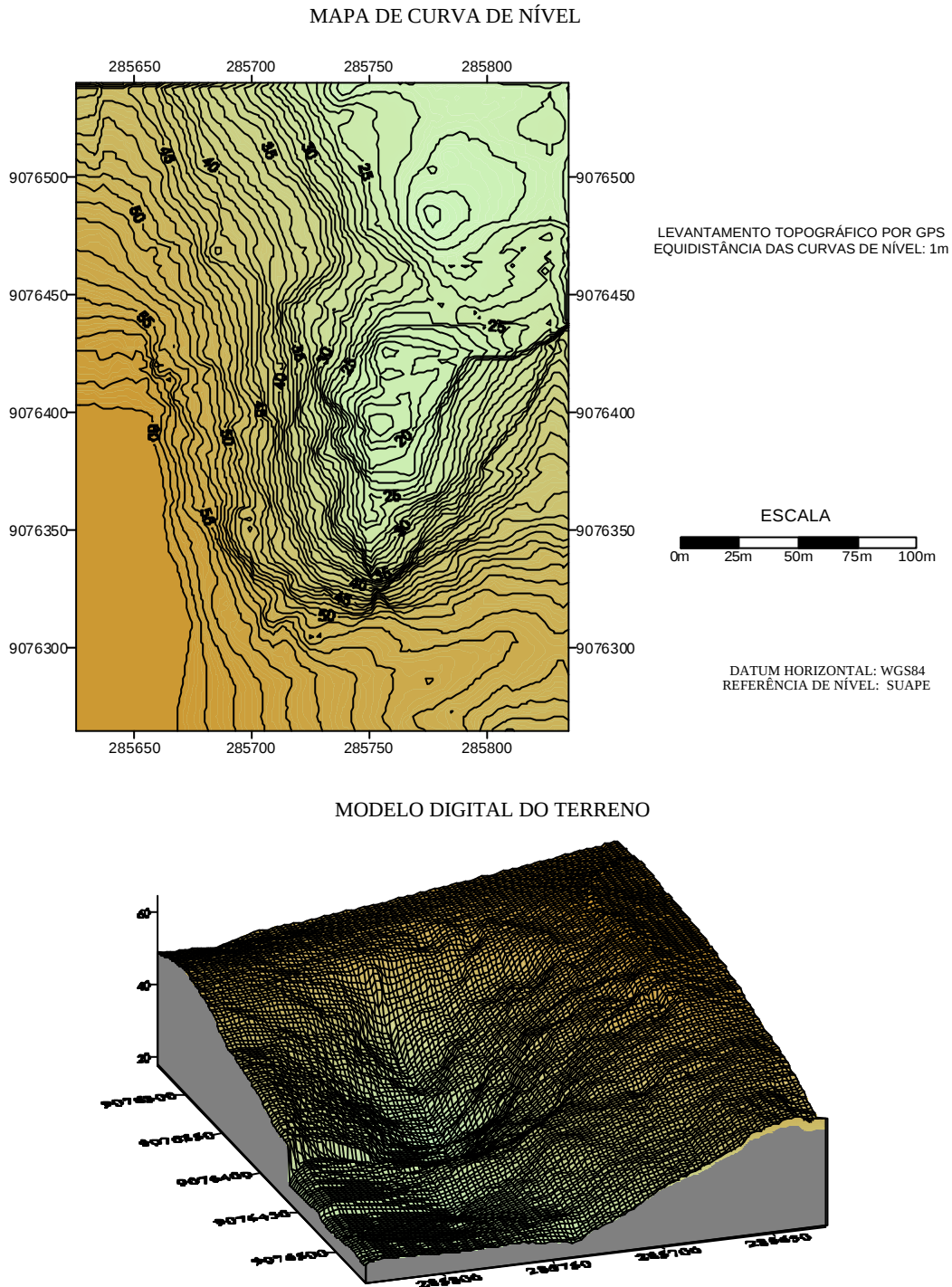
Figura III.19 – Topografia e Modelo Digital do Terreno – Ponto P-01 - encosta central, SILVA (2004).
