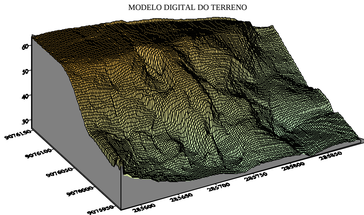
Figura III.20 – Topografia e Modelo Digital do Terreno– Ponto P- 02 - encosta sul, SILVA (2004).
