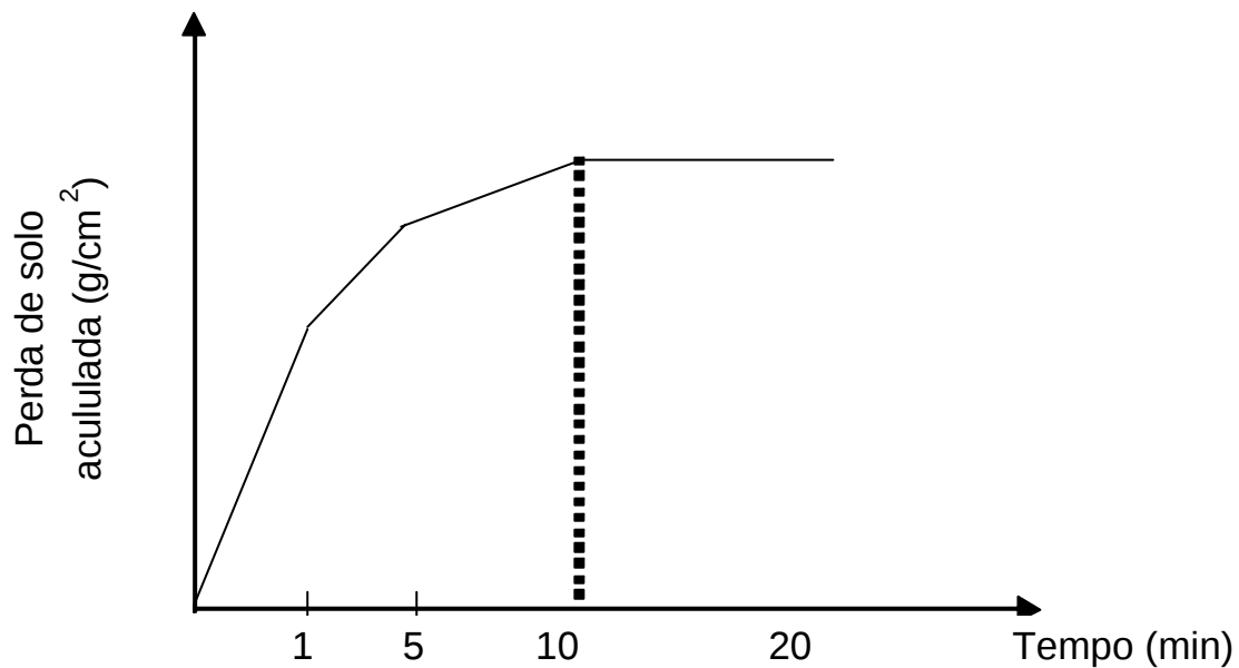
Figura IV.25 – Curva típica de perda de solo acumulada versus tempo do ensaio.
