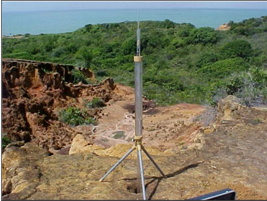
Figura IV.3 – Ensaio de permeabilidade com o Permeâmetro Guelph – Ponto P – 01 - encosta central.
