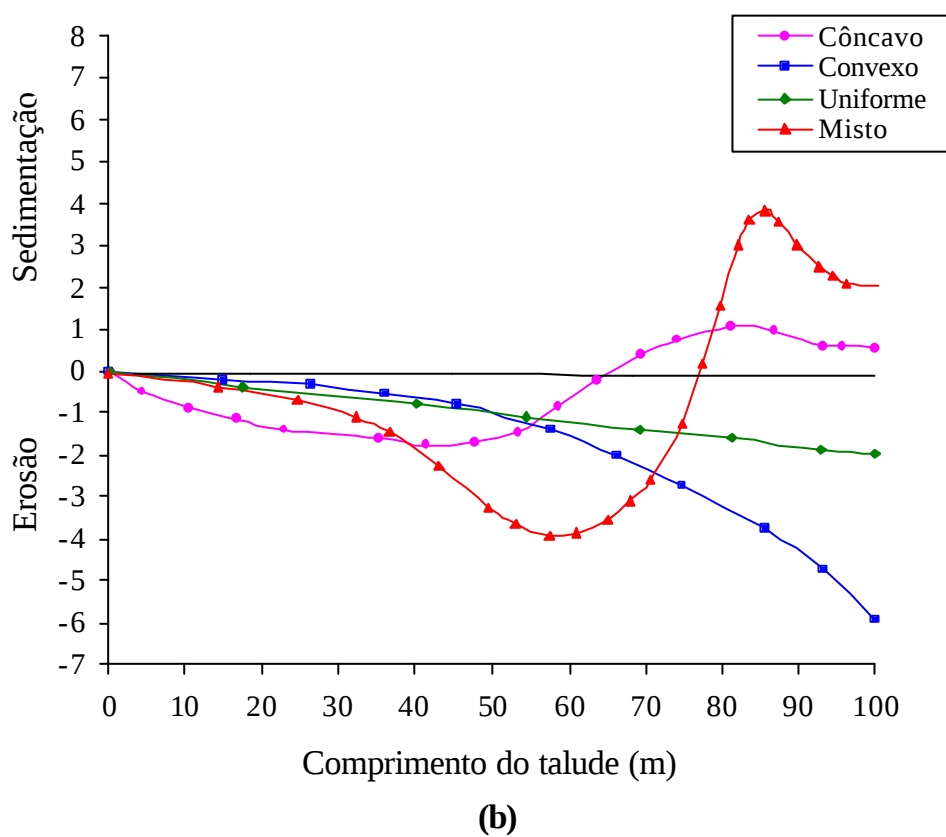
Figura II.8 – (a) Formas típicas de taludes; (b) saldo de materiais erosão/deposição, PERRENS et al. (1984).
