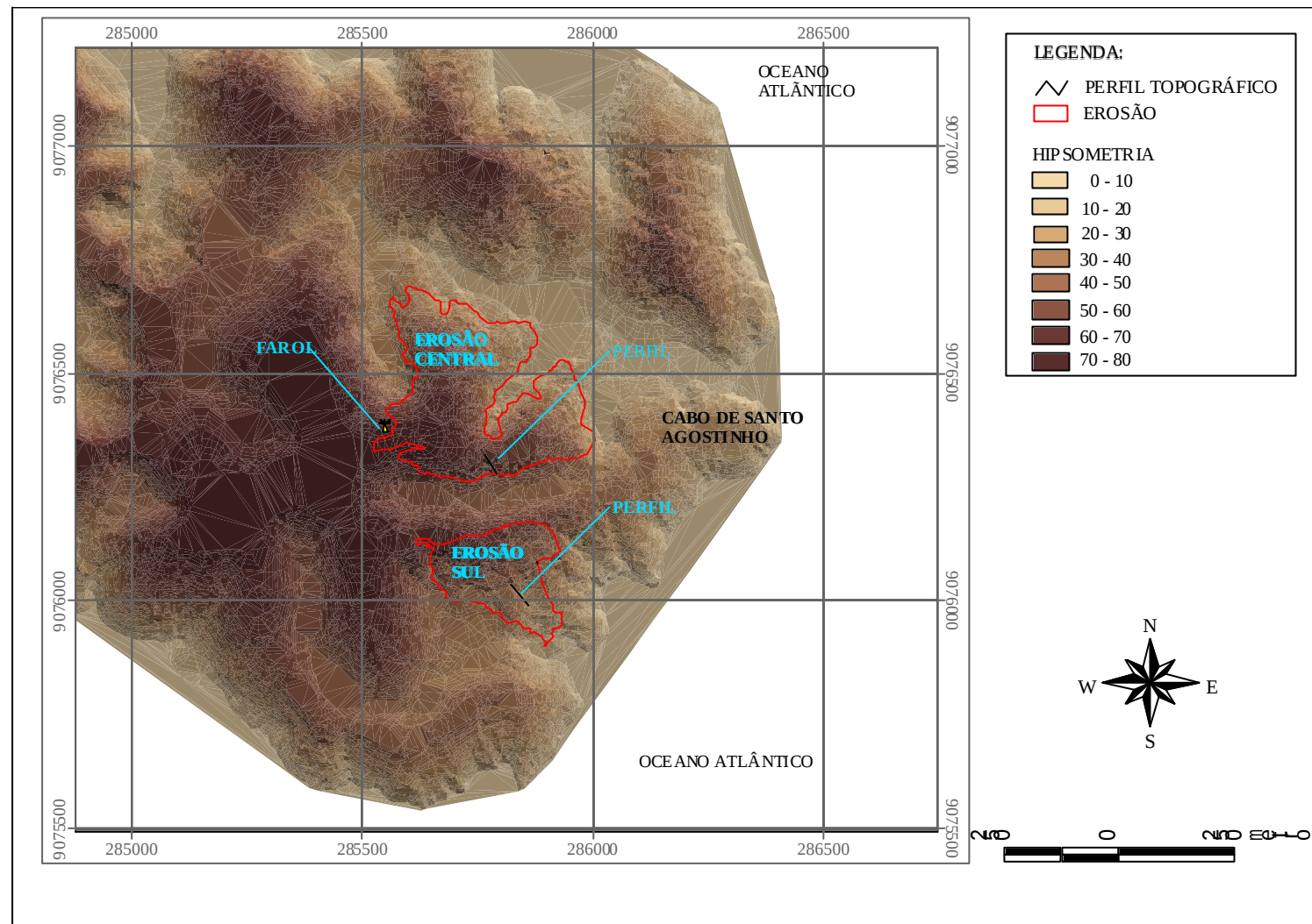
Figura III.14 – Mapa de relevo com locação dos perfis topográficos, SILVA (2004).
