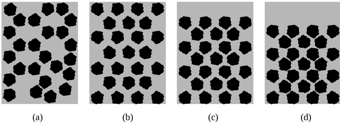
Figura II.10 – Sequência do processo de liquefação, ISHIHARA et al. (1980)
