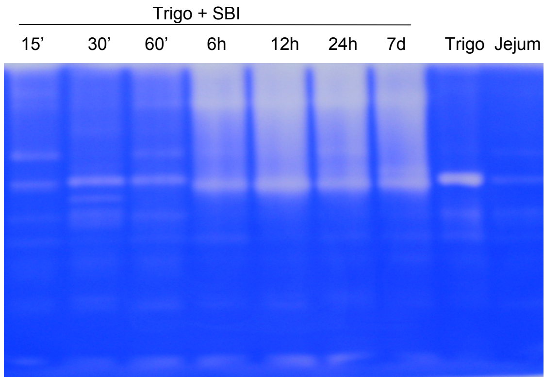
Figura 5 - Curso temporal após a alimentação com inibidor. Zimograma apresenta as diferenças nas atividades proteolíticas em jejum, na alimentação com farelo de trigo e de acordo com o tempo de alimentação em dieta SBI (inibidor de tripsina e de quimotripsina de soja).
