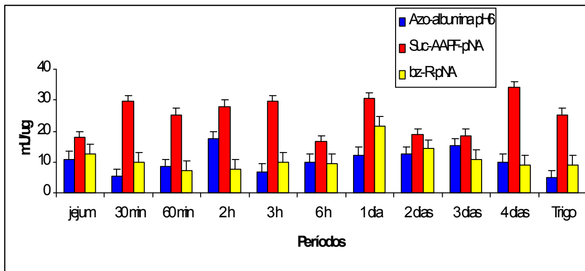
Figura 6: Atividade proteolítica dos homogeneizados intestinais de larvas de T. molitor após alimentação com o inibidor de tripsina e quimotripsina de soja (SBI). O gráfico apresenta as atividades em insetos alimentados após diferentes períodos de tempo. O grupo jejum corresponde aos animais mantidos sete dias sem alimentação, enquanto o grupo trigo corresponde aos animais alimentados com o farelo de trigo.
