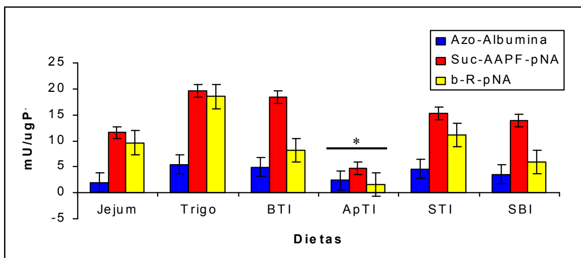
Figura 3 - Atividade proteolítica dos homogeneizados intestinais de larvas de T. molitor alimentadas com diferentes inibidores. O grupo denominado jejum corresponde aos animais mantidos sete dias sem acesso a alimento; o grupo Trigo corresponde aos animais alimentados somente com farelo de trigo, enquanto os grupos BTI, ApTI, STI e SBI correspondem aos animais alimentados em dietas onde os inibidores foram incorporados (na concentração de 0,4% m/m) ao farelo de trigo usado como excipiente.
