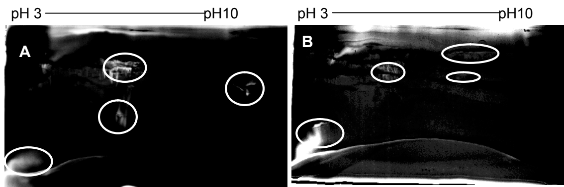
Figura 11 - Zimograma bidimensional. Destacam-se os diferentes “spots” de proteinases (circundados) encontrados no gel de animais alimentados com trigo em A e alimentados com BTI incorporado no trigo em B.
