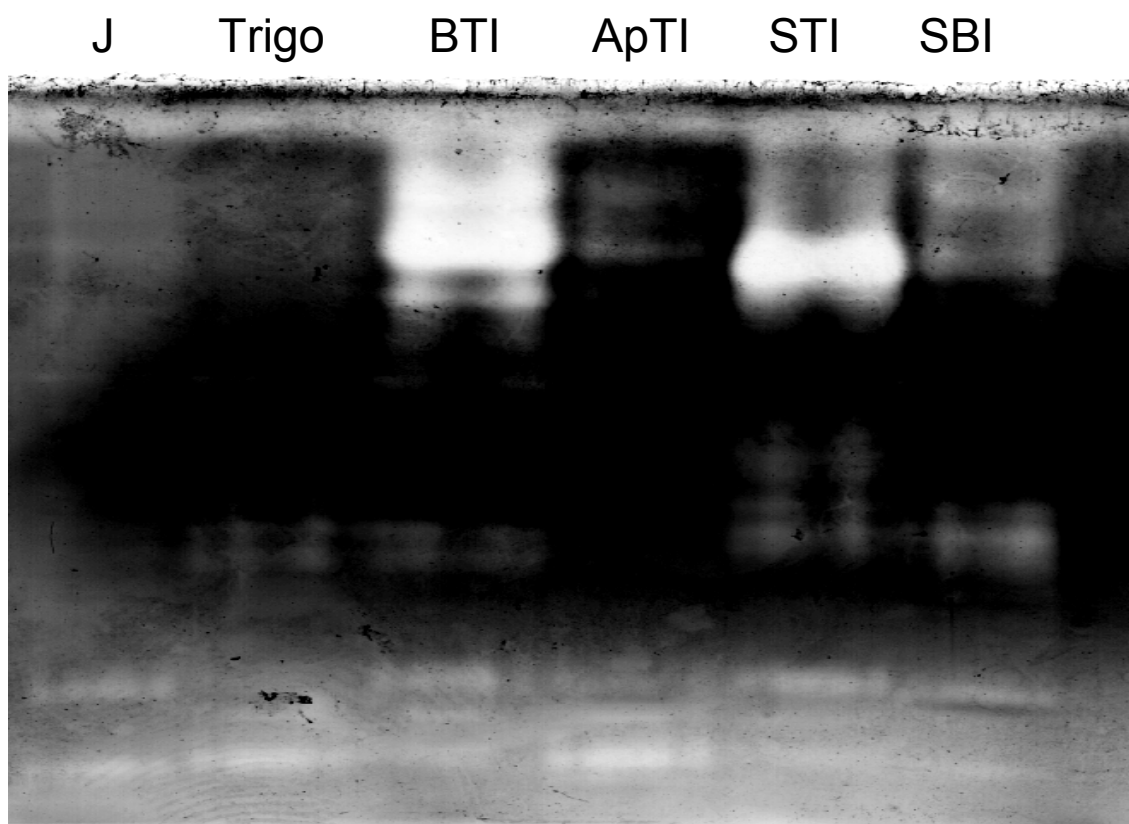
Figura 4 - Comparação entre os padrões de atividade proteolítica de homogeneizados intestinais de larvas de T. molitor mantidas em jejum e alimentadas com farelo de trigo e com dietas contendo inibidores purificados. Os homogeneizados foram obtidos de larvas mantidas em diferentes dietas: jejum (J), trigo (Trigo), BTI (inibidor de tripsina de Phaseolus vulgaris ), ApTI (inibidor de tripsina de Adenantha pavonina ), STI (inibidor de tripsina de soja), SBI (inibidor de tripsina e de quimotripsina de soja). Em cada raia as amostras possuíam a mesma quantidade de proteína.
