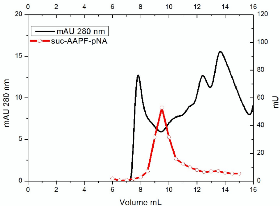
Figura 9 - Perfil da filtração em Gel. Após filtração em gel com a coluna superdex 75, as frações obtidas foram testadas frente ao substrato suc-AAPF-pNA, destaque para aumento de atividade em torno do pico formado em 10 mL de eluição. Curva em preto representa o perfil protéico das frações (mAU 280 nm).
