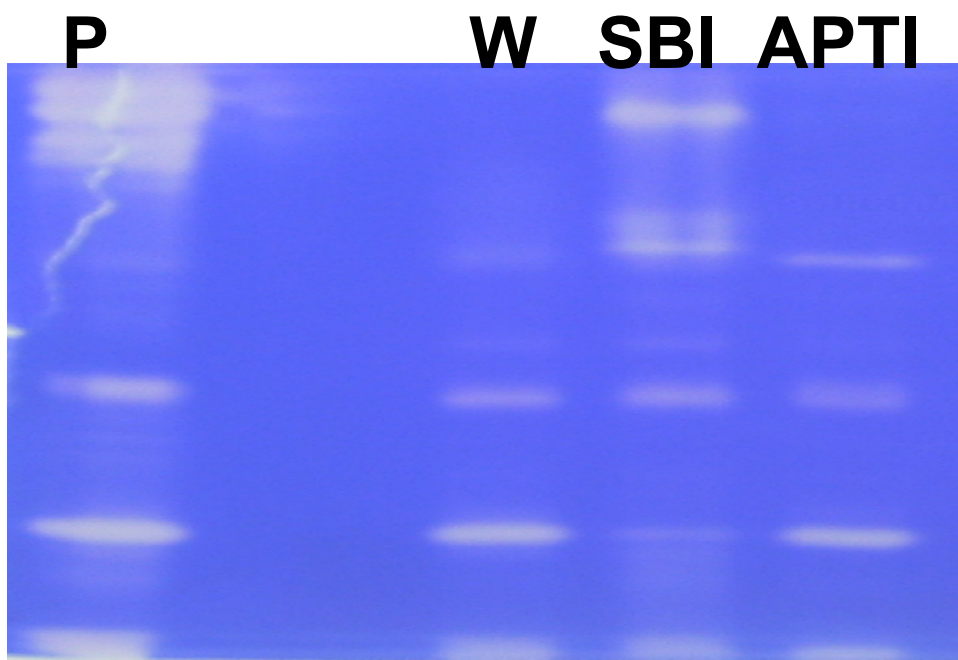
Figura 2 - Comparação entre os padrões de atividade proteolítica de homogeneizados intestinais de larvas de T. molitor alimentadas com farinha de semente do feijão comum ( P. vulgaris ) e com dietas contendo inibidores purificados. Este zimograma mostra o padrão de proteinases em animais alimentados com farinha de P. vulgaris ( P ) em relação ao grupo controle alimentado com farelo de trigo ( W ) e em relação aos animais alimentados com inibidores puros incorporados na dieta controle ( SBI e ApTI ).
