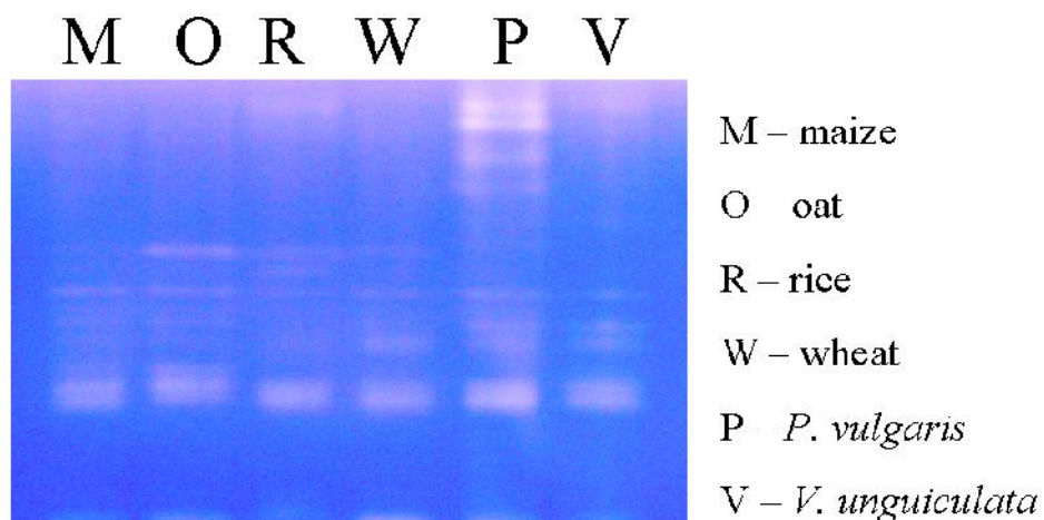
Figura 1 - Padrão de atividade proteolítica de homogeneizados intestinais de larvas de T. molitor alimentadas com farinhas de diferentes sementes. Diferenças na atividade de proteinases intestinais foram observadas quando as larvas foram alimentadas com diferentes dietas. Notar na raia P, que pelo menos quatro proteinases de baixa migração eletroforética mostram maior atividade do que as demais dietas. M, farinha de sementes de milho; O, farinha de sementes de aveia; R, farinha de sementes de arroz; W, farinha de sementes de trigo; P, farinha de sementes de feijão
