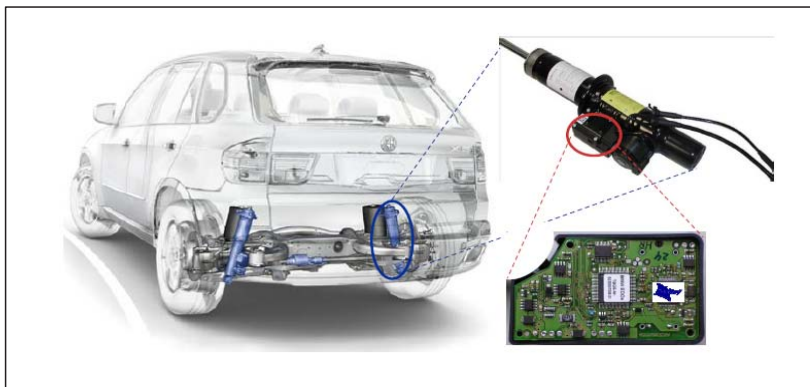
Figura 2.11: Suspensão eletrônica de veículos BMW X5 (SCHEDL, 2007)
