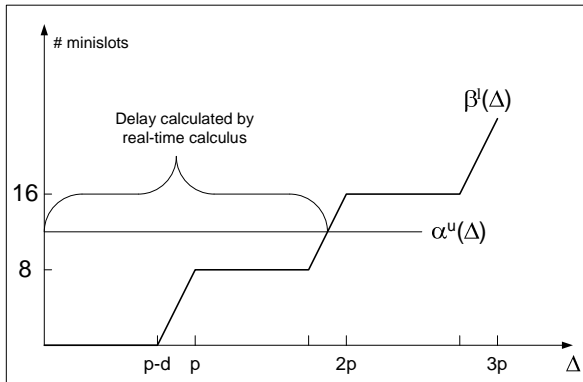
Figura 3.6: Máximo atraso de \alpha^u e \beta^l (HAGIESCU et al., 2007)
