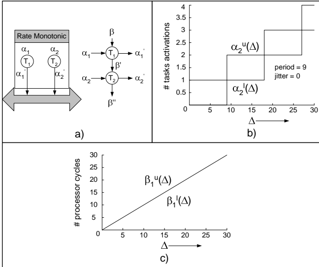
Figura 3.3: a) Escalonamento rate-monotonic para duas tarefas e rede de escalonamento correspondente. b) Curvas \alpha^u e \alpha^l correspondentes a uma ativação periódica. c) Curvas \beta^u e \beta^l para um processador sem carga. (HAGIESCU et al., 2007)
