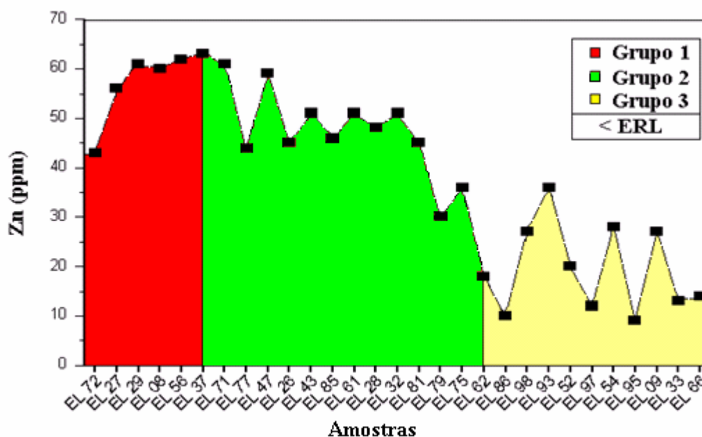
Figura 30 - Dispersão geoquímica do zinco segundo o PC1.
