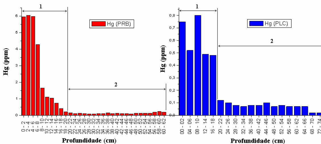
Figura 91 - Variações das concentrações de Hg nos perfis do rio Botafogo (PRB) e Lanço dos Caçõs (PLC)
