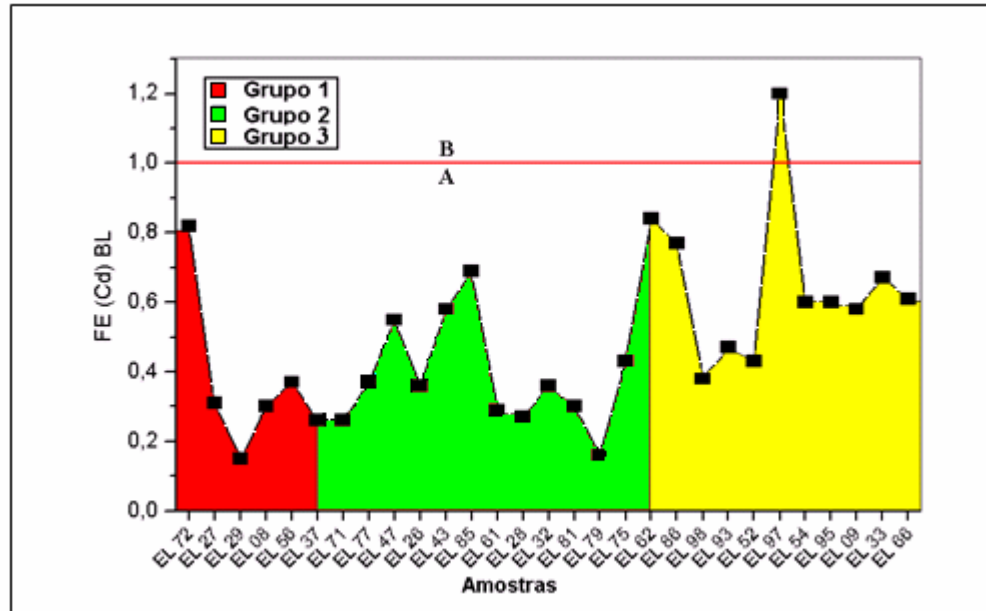
Figura 36 – FE da dispersão geoquímica do cádmio, segundo o PC1.
