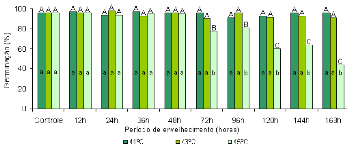
Figura 3 – Porcentagem de germinação de sementes de Vochysia divergens submetidas ao envelhecimento acelerado nas temperaturas de 41, 43 e 45°C, durante 0, 12, 24, 36, 48, 72, 96, 120, 144 e 168 horas. Letras maiúsculas comparam os períodos na mesma temperatura e letras minúsculas comparam as temperaturas no mesmo período, a 5% pelo teste de Scott-Knott.
