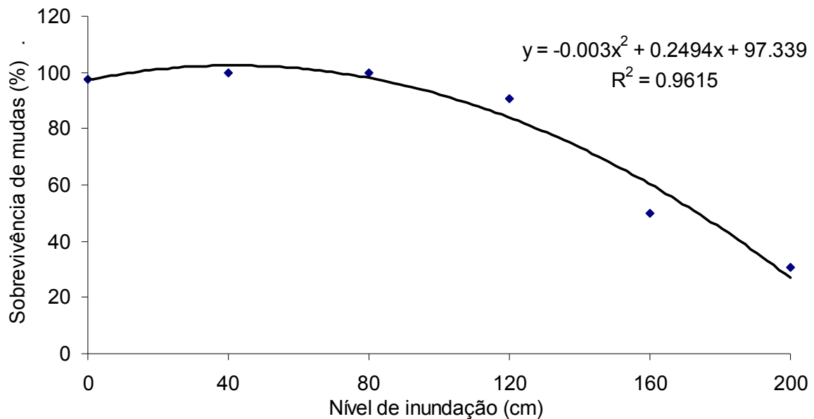
Figura 4 – Varia o da sobreviv ncia de mudas de Vochysia divergens em diferentes n veis de inunda o.
