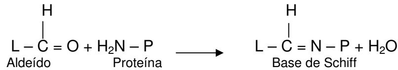
Figura 3 – Formação do complexo base de Schiff.
