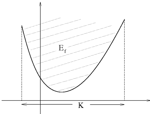
Figura 1.5: Função convexa.
