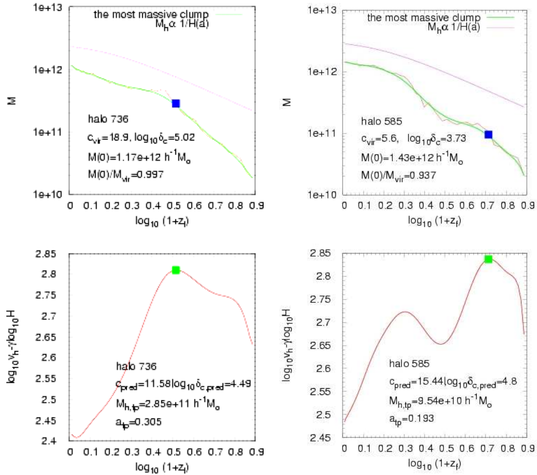
Figura 5.1: Implementação do método proposto por Zhao et al. (2003) (em baixo) para encontrar o turning point , z_{tp} , na curva de acreção de massa do progenitor mais massivo (em cima). A curva suave corresponde ao ajuste de uma curva de Beziér a M(z) medida na simulação. Ambas curvas de acreção resultam em halos de massa \sim 10^{12} h^{-1} M_\odot e ilustram um caso onde há duas fases de acreção distintas e outro caso onde a proposta de Zhao et al. (2003) não se aplica. Os parâmetro de concentração medido e previsto são mostrados nos painéis em cima e em baixo respectivamente.
