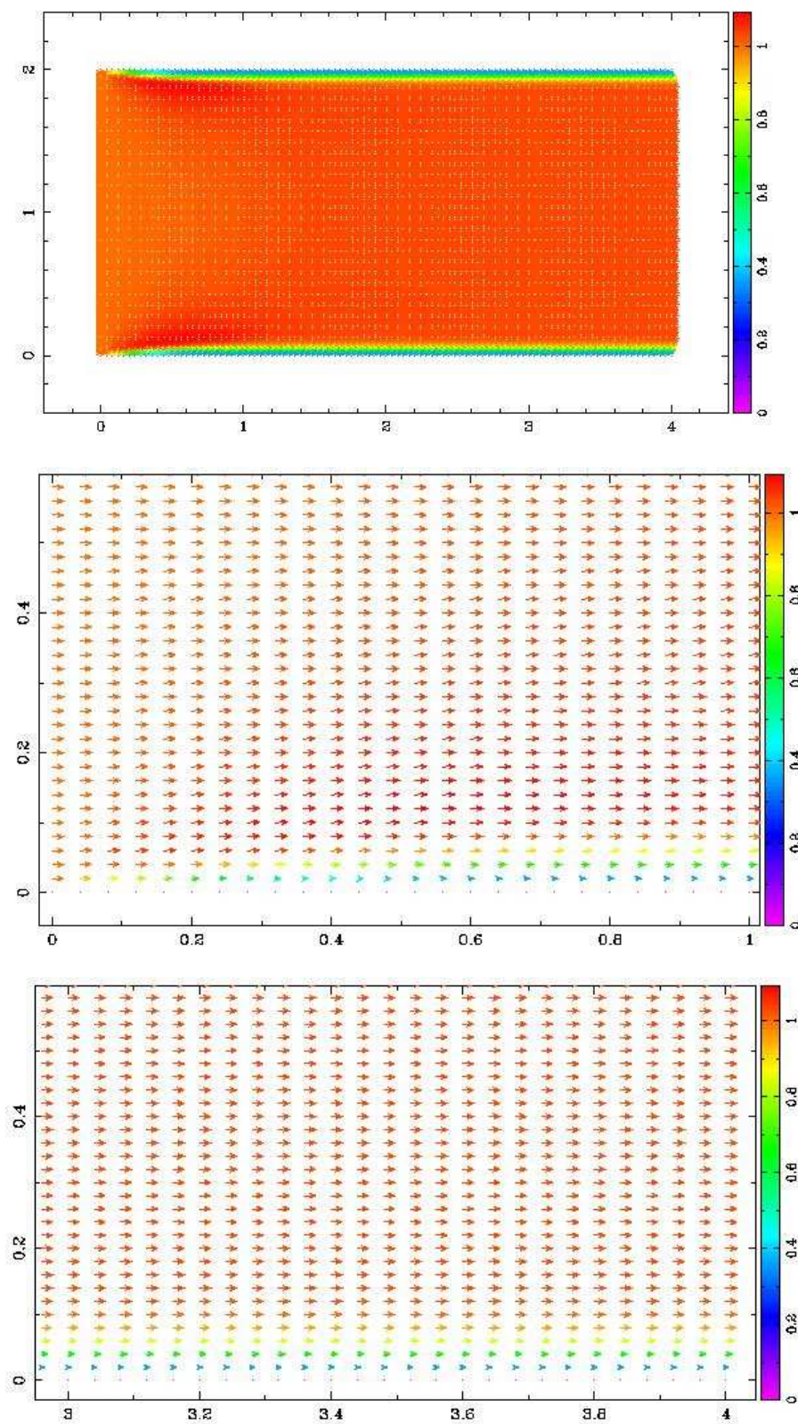
Figura 4.7: Malha com 101 \times 101 pontos com Re = 1000 : (a) domínio completo, (b) ampliação na entrada e (c) ampliação na saída.(onde a escala de cores representa a magnitude dos vetores)
