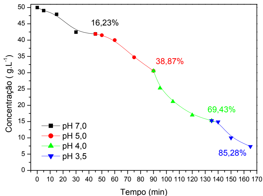
Figura 4.13.: Resultados da adsorção de penG a 4°C na faixa de pH de 3,5 a 7,0 utilizando 2 g de XAD-4 adicionados gradativamente em 40mL de caldo com 50g.L -1 de penG
