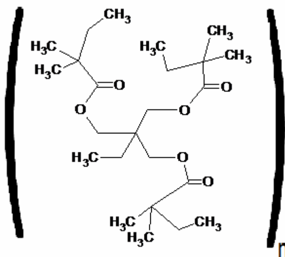
Figura 2.11.: Estrutura química da resina Amberlite XAD-7
