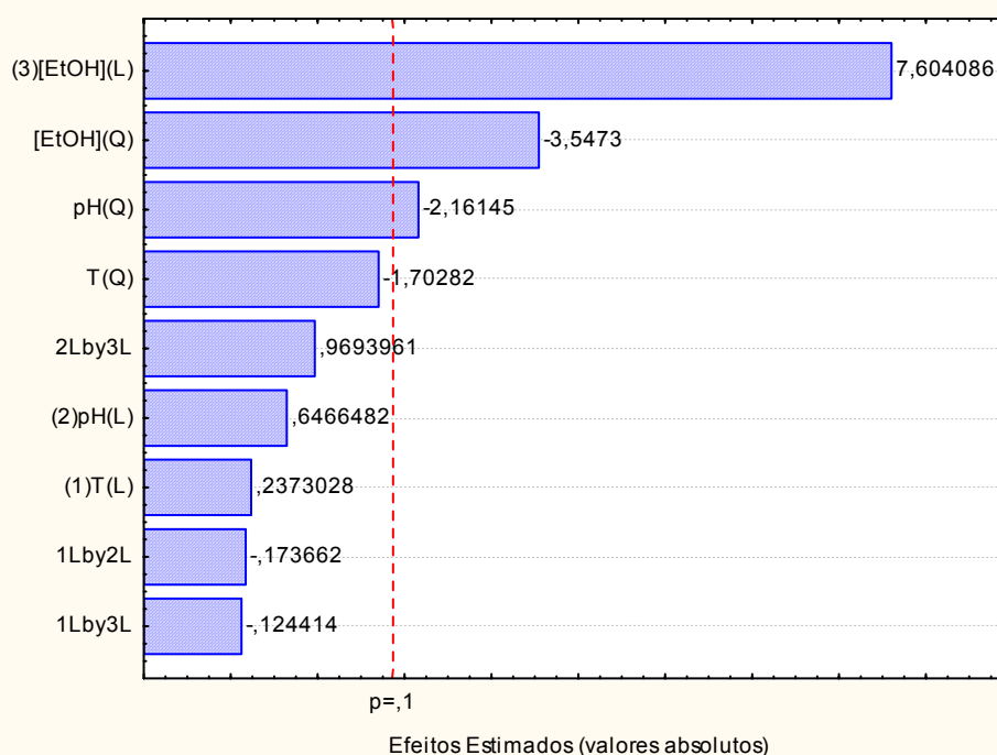
Figura 4.16.:Diagrama de Pareto para o 1º delineamento
