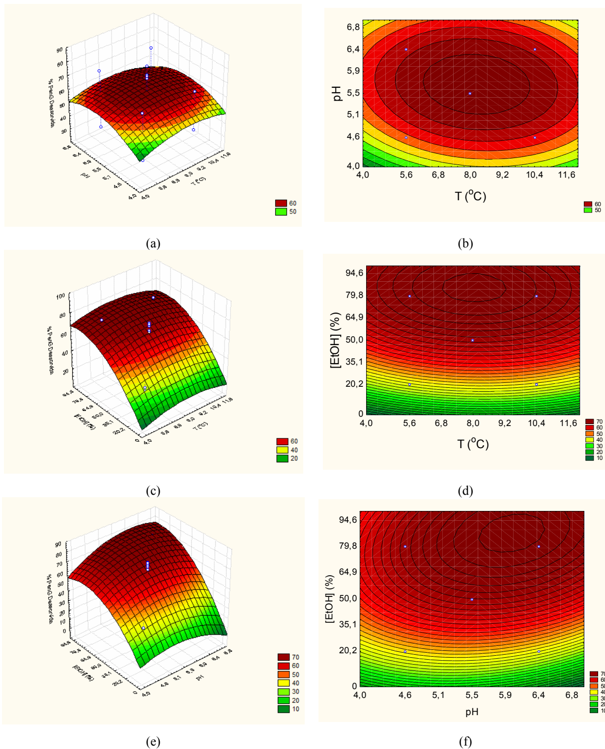
Figura 4.19.: Superfícies de resposta e curva de contorno para a dessorção de penG (%) em função da temperatura e pH (a) e (b), da temperatura e [EtOH] (c) e (d) e do pH e [EtOH] (e) e (f) no 1º delineamento
