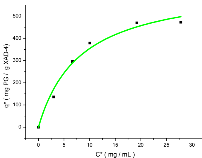
Figura 4.12.: Isotermas de Adsorção- Modelo de Langmuir, utilizando 0,1 g (em base seca) de XAD-4 pré-tratado para 2mL de água deionizada.
