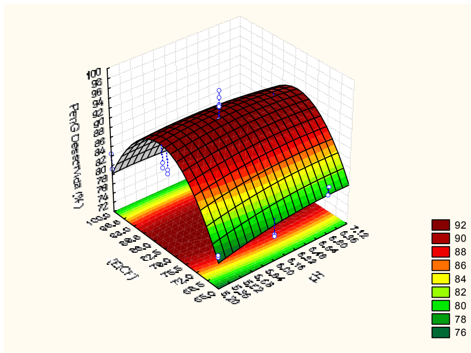
Figura 4.23.: Superfícies de resposta para a dessorção de penG (%) em função da temperatura e [EtOH] no 2º delineamento
