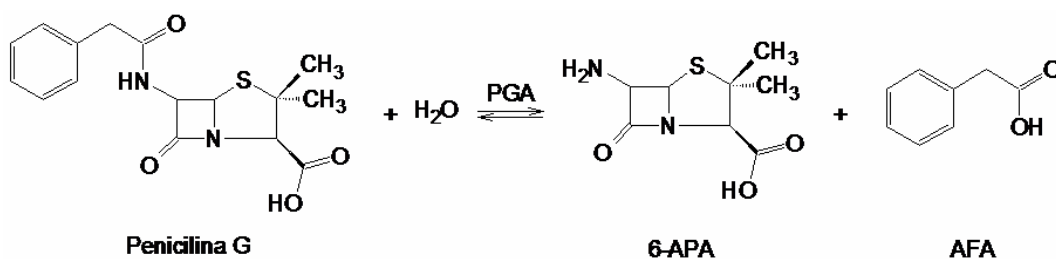
Figura 2.3.: Esquema da hidrólise de penicilina G catalisada pela enzima penicilina G acilase
