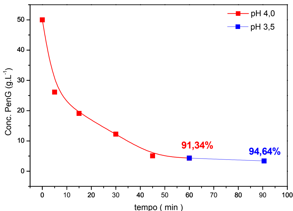
Figura 4.15.: Resultados da adsorção de penG a 4°C na faixa de pH de 3,5 a 4,0 utilizando 1,5g de XAD-4 adicionado em 18mL de caldo com 50 \text{ g.L}^{-1} de penG
