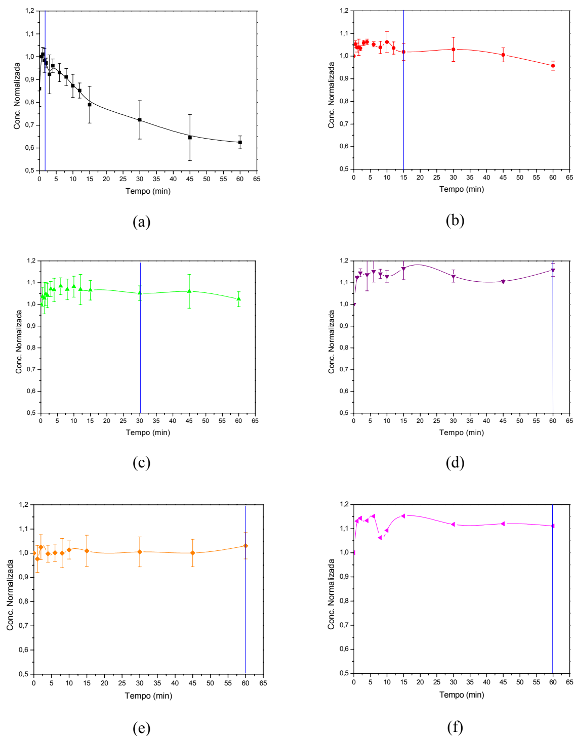
Figura 4.3.: Gráfico da estabilidade de PenG a 4°C em diferentes valores de pH (a) 2,0 (b) 2,5, (c) 3,0, (d) 4,0, (e) 5,0, (f)7,0.
