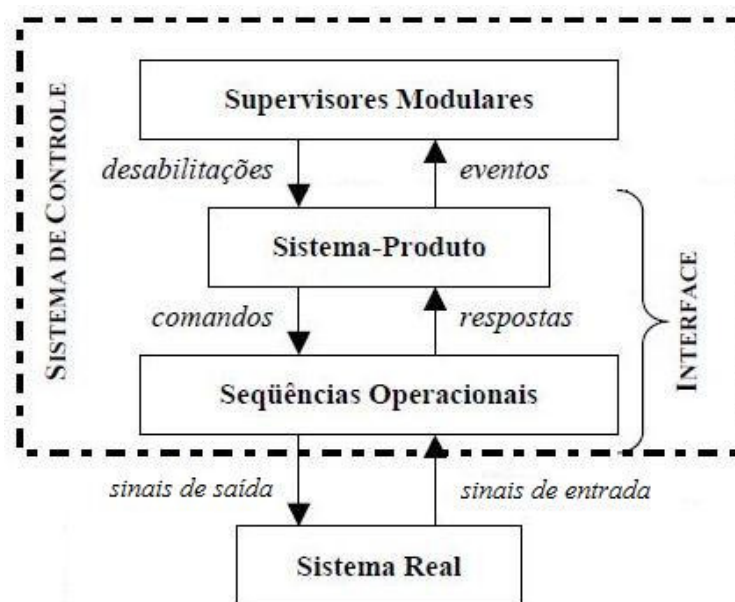
Figura 5.1. Estrutura do sistema de controle (Queiroz, 2000)
