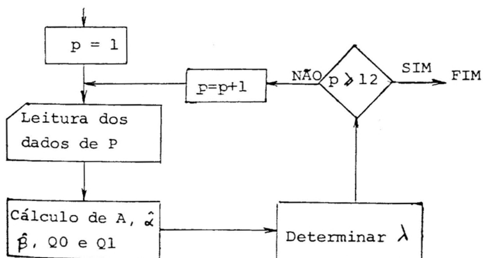
FIGURA 7 - Diagrama de Blocos da Metodologia Utilizada pelo Software Gamma para o Cálculo da Precipitação que Tem 25 % de Probabilidade de Ocorrer.
