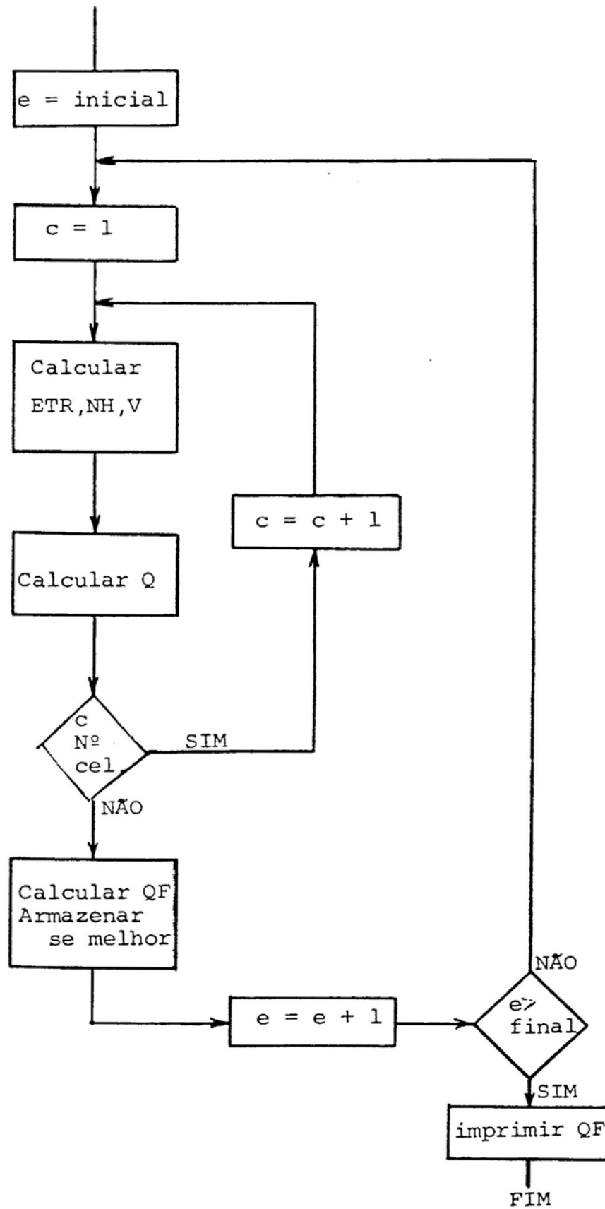
FIGURA 12 - Fluxograma do Programa de Simulação.
