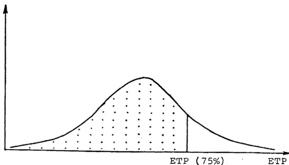
FIGURA 5 - Distribuição dos Dados de Evapotranspiração Potencial e a Posição do Valor que Tem 75 % de Probabilidade de Ocorrer.
