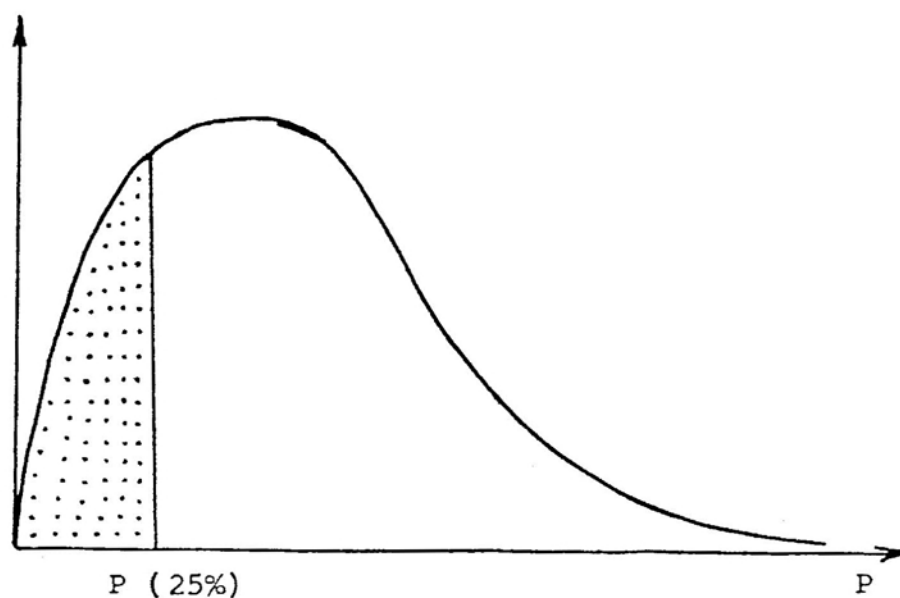
FIGURA 6 - Gráfico da Função de Probabilidade Gama Incompleta.
