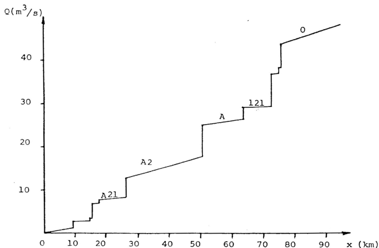
FIGURA 13 - Vazão do Rio Verde Grande em Função da Sua Abscissa, em Seu Trecho de Maior Comprimento, para o Mês de Setembro.
