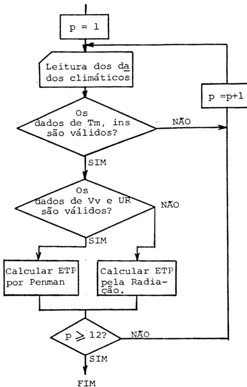
FIGURA 4 - Diagrama de Blocos do Programa GeraETP.
