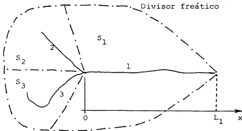
FIGURA 11 - Curso d'Água Hipotético.
