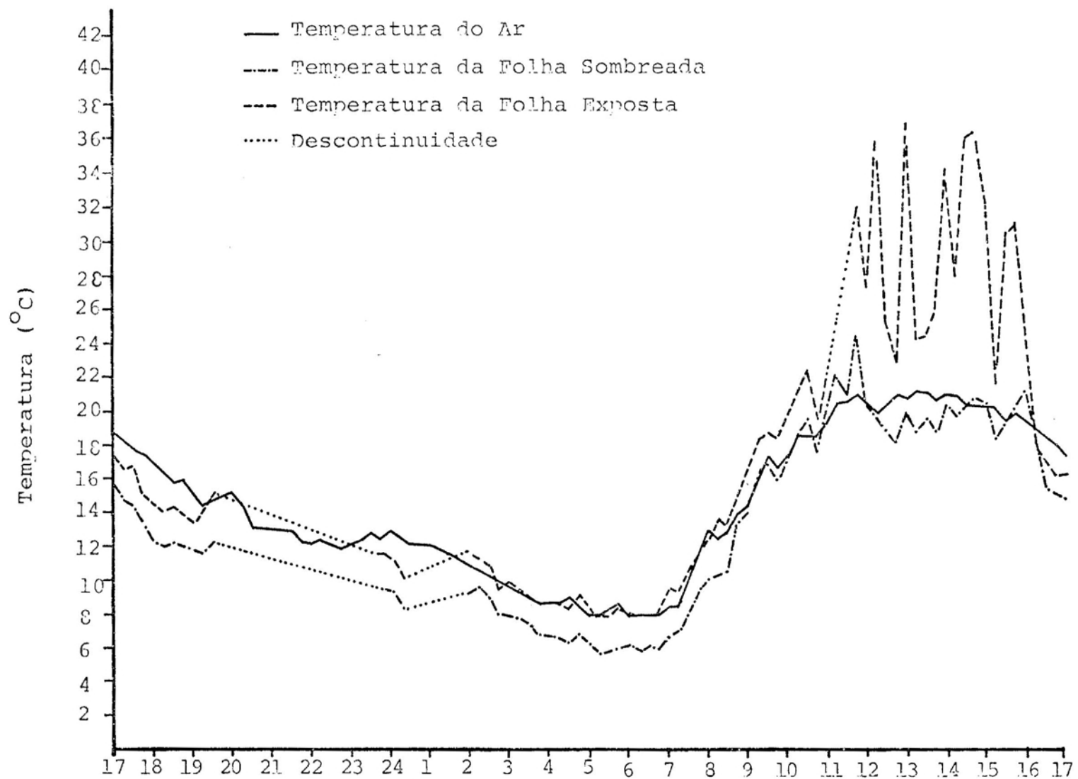
FIGURA 3 - Marcha Diária da Temperatura da Folha e da Temperatura do Ar, para a Cultura de Café, Obtida nos Dias 24 e 25 de Julho de 1985.
