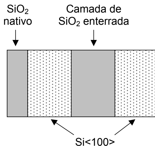
Fig. 4.1: Estrutura de uma amostra de SIMOX.
