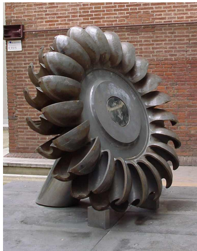
FIGURA 2.6– Rotor de uma turbina do tipo Pelton, mostrando a estrutura das pás. FONTE – http://upload.wikimedia.org/
