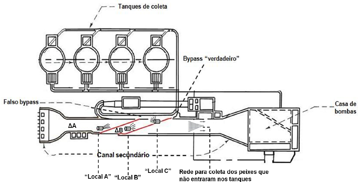
FIGURA 3.14 – Planta baixa do canal secundário do Tracy Fish Collection Facility mostrando os locais de instalação do equipamento de luz estroboscópica para os testes com Delta smelt ("Local A") e Splittail ("Local B" e "Local C") e os locais de soltura \Delta A e \Delta B para Delta smelt e \Delta A para Splittail. Adaptado de Bowen et al. (2004).
