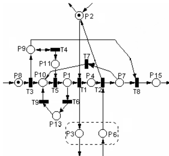
Figura 4.10: Gerenciador de mensagens para mensagem periódica.
