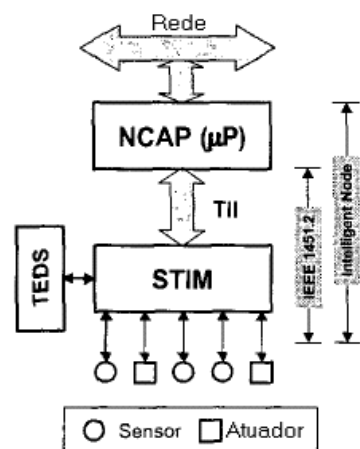
Figura 2.8: Padrão IEEE 1451.
