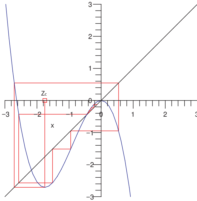
Figura 2.5: Órbita de z_c , para c = 2.6345 , após 10 iteradas.
