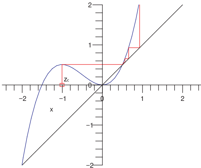
Figura 2.3: Órbita de z_c , para c = 1.51 , após 10 iterações.
