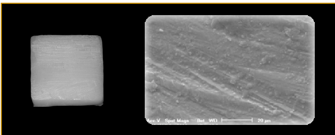
Figura 18: Fotografia e microscopia da superfície externa da zircônia após desgaste com ponta diamantada (magnificação 2000X).
