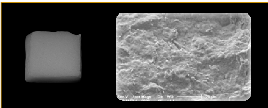
Figura 17: Fotografia e microscopia da superfície interna da zircônia (magnificação 2000X).
