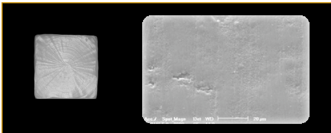
Figura 16: Fotografia e microscopia da superfície externa da zircônia (magnificação 2000X).
