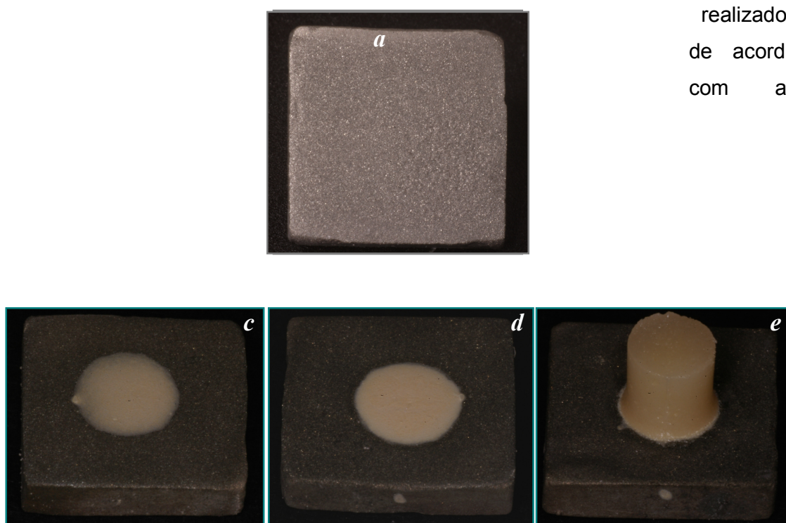
Figura 4: Infra-estrutura metálica (lixa 220) (a); após jateamento com óxido de alumínio (b); sinterização do opaco primeira camada (c); sinterização da segunda camada do opaco (d); e sinterização da massa de dentina (e).
