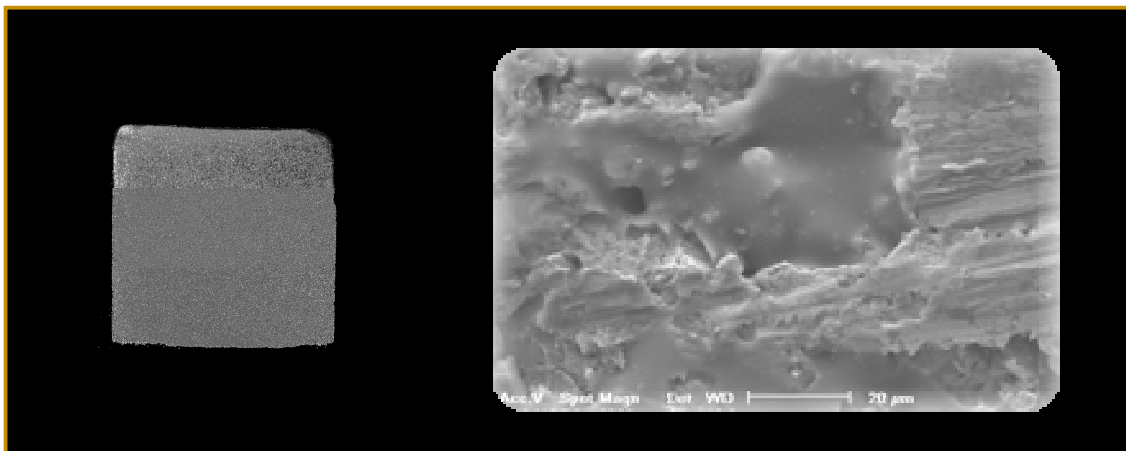
Figura 19: Fotografia e microscopia da superfície externa da liga metálica após jateamento com óxido de alumínio (magnificação 2000X).
