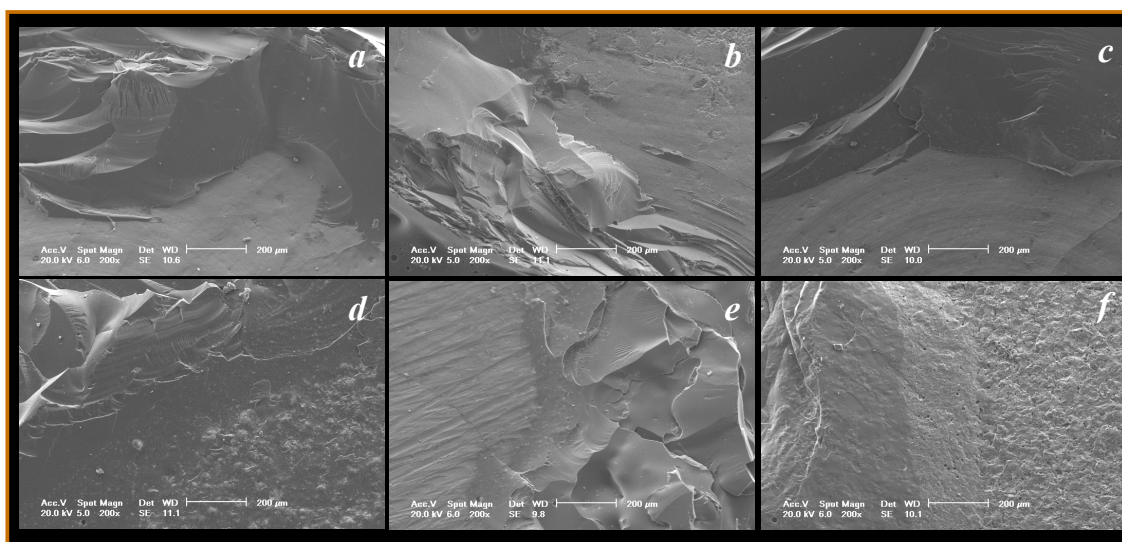
Figura 22.: Imagens microscópicas (magnificação 200X) referentes a transição entre infraestrutura e cerâmica de cobertura pós fratura. Grupo1 (a), 2 (b), 3 (c), 4 (d), 5 (e) e controle (f).
