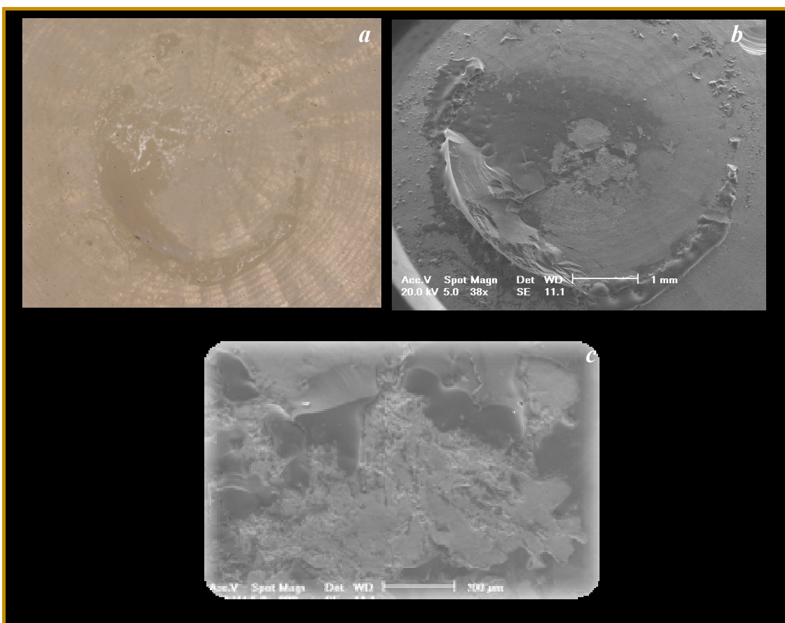
Figura 20: Imagem referente a uma amostra do grupo 2 (zircônia com cor). Observa-se praticamente a mesma qualidade de imagem da fotografia, pós cisalhamento (a), quando comparada com a microscopia numa magnitude de 38x (b). Analisando em um maior aumento (200x), observa-se uma interação da cerâmica de cobertura com a superfície da zircônia.
