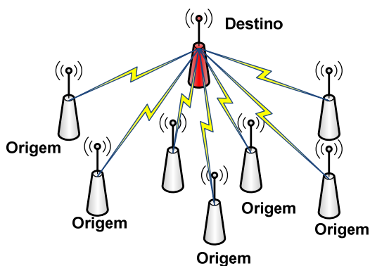
Figura 2.9 – Fusão de dados paralela.
