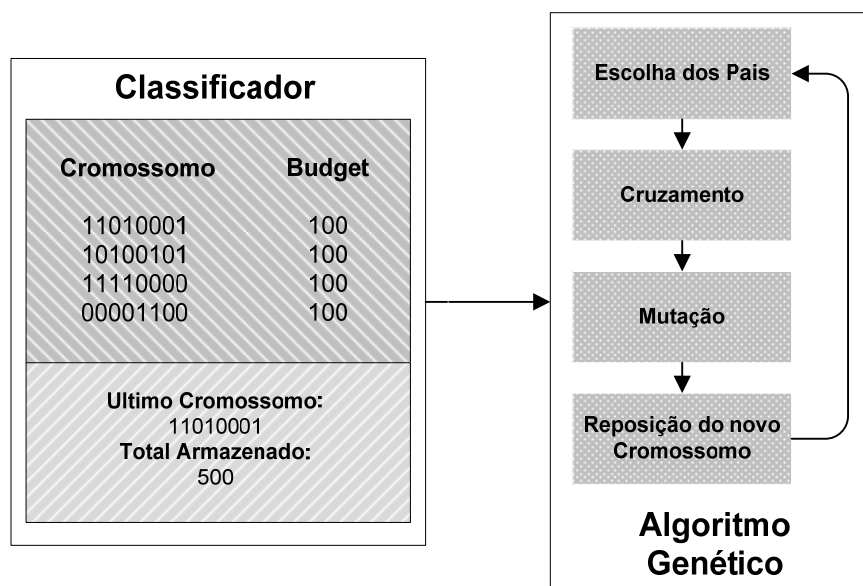
Figura 4.10 – Estrutura do classificador no algoritmo genético.
