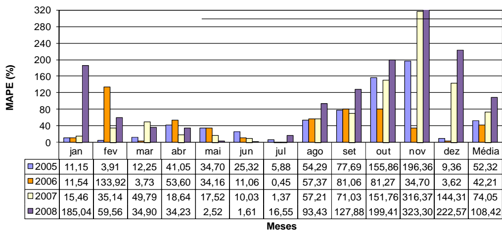
Figura 6.4 Erro da previsão do ano de 2005, 2006, 2007 e 2008 com a Configuração 3.
