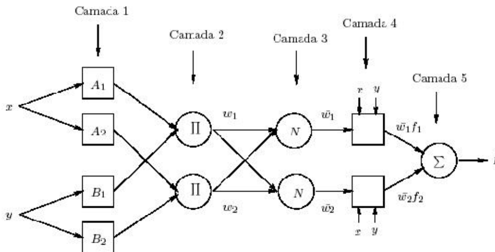
Figura 3.2 Arquitetura Neuro-Fuzzy: ANFIS.
