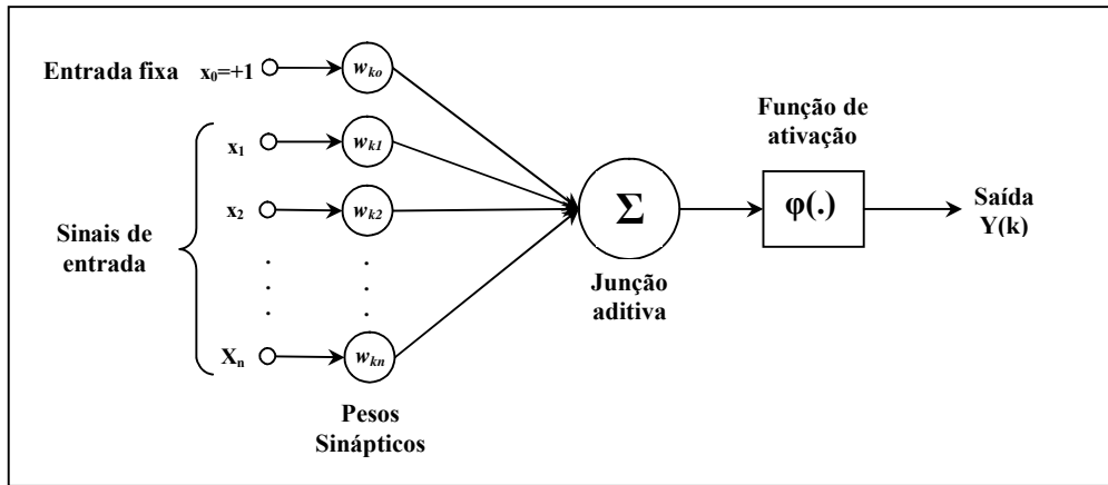
Figura 2.1 Modelo de um Neurônio Artificial.
