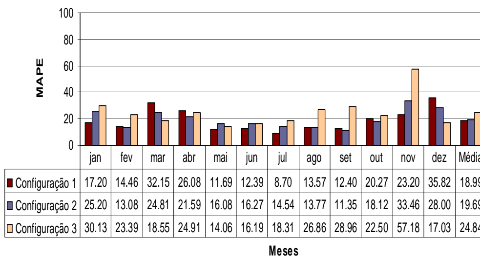
Figura 6.1 MAPE das três configurações.
