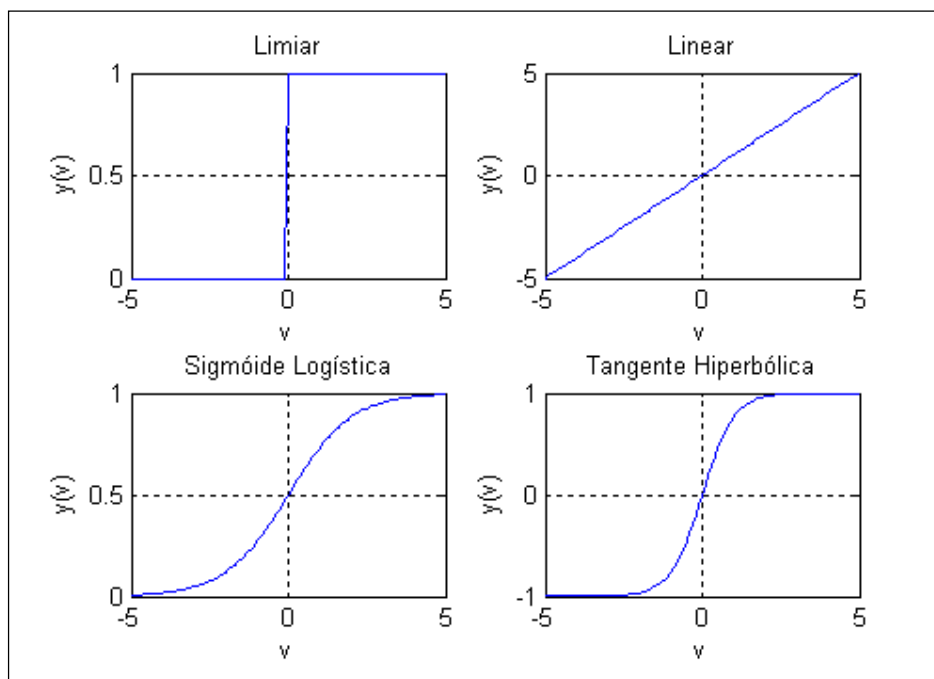
Figura 2.2 Funções de Ativações.
