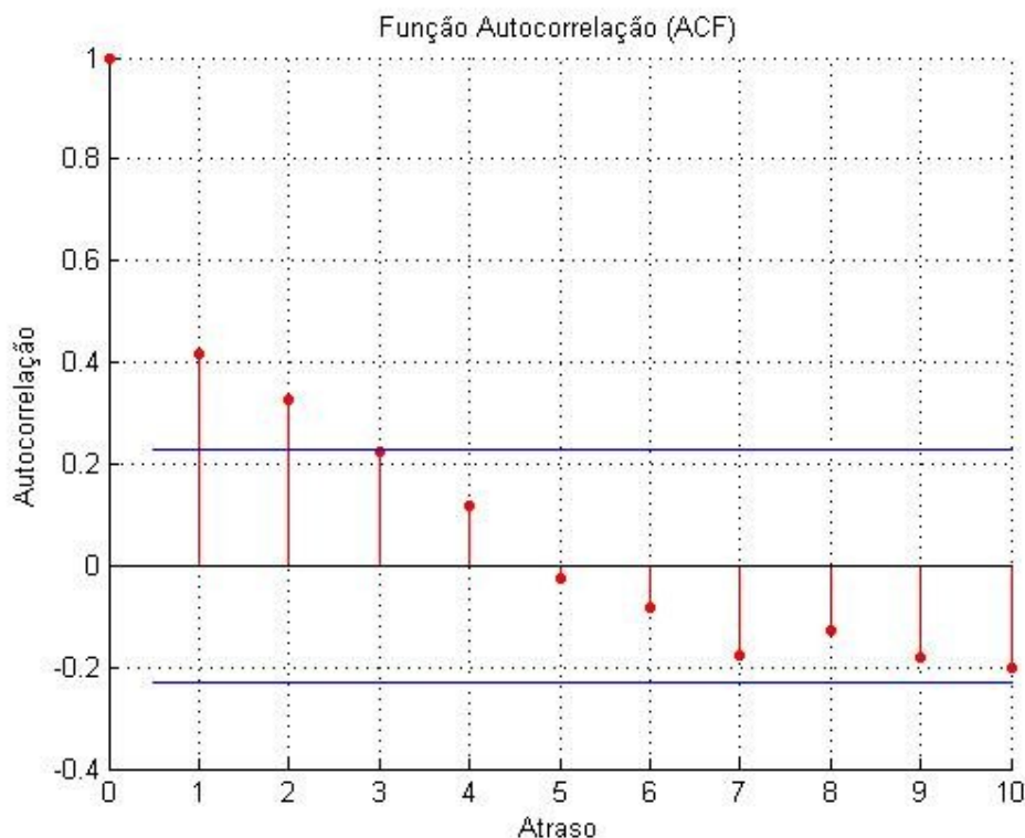
Figura 5. 2 Função Autocorrelação Anual.
