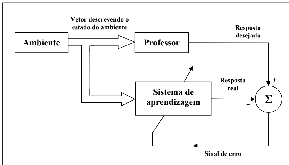
Figura 2.3 Diagramas de Blocos da Aprendizagem com Professor.
