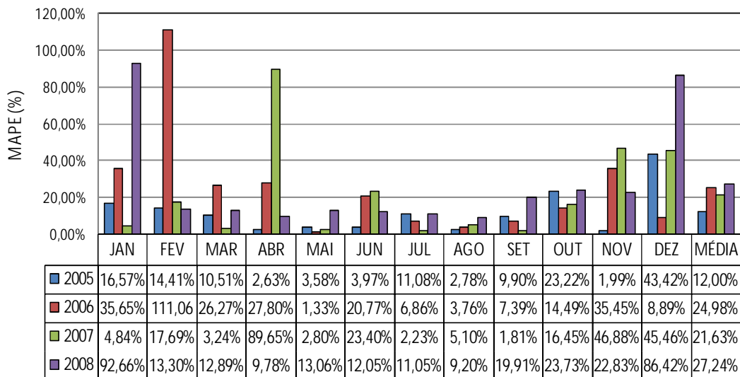
Figura 6.9 MAPE da Previsão na Configuração Um Mês à Frente com o ANFIS.
