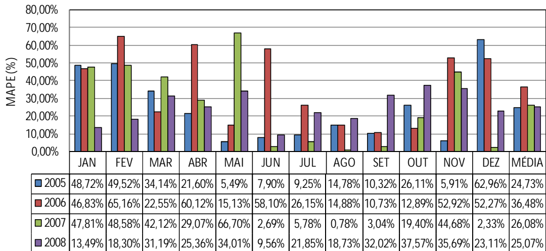
Figura 6.8 MAPE da Previsão na Configuração Dois Meses à Frente com RNA.
