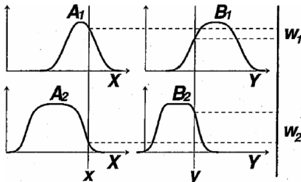
Figura 3.3 Exemplo do Sistema Takagi-Sugeno de Primeira Ordem.
