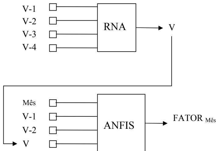
Figura 5. 6 Modelo de previsão Híbrido RNA-ANFIS.
