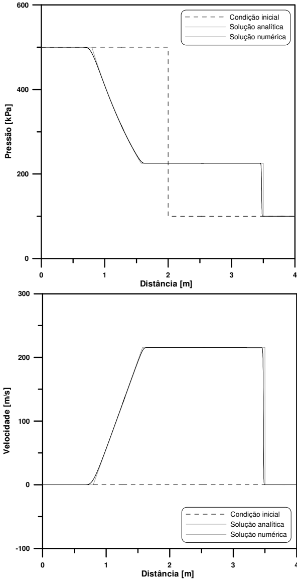
Figura 3.7 – Campos de pressão e velocidade em t = 3ms . Comparação da solução analítica exata com os resultados numéricos obtidos pela formulação conservativa de primeira ordem.
