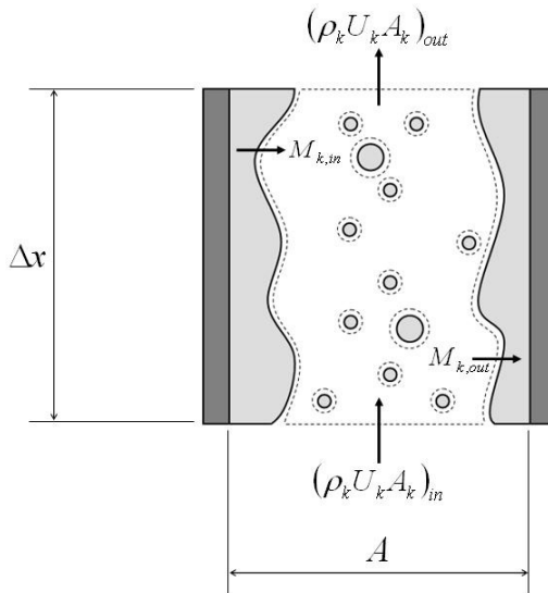
Figura B.1 – Geometria do duto, arranjo de fases e balanço de massa no volume de controle.
