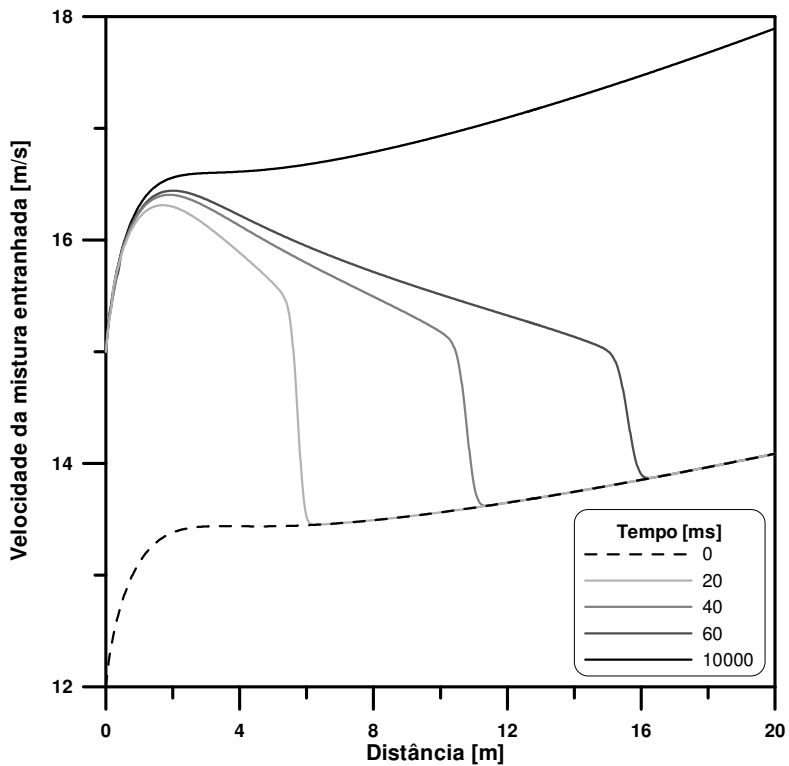
Figura 6.4 – Campos de velocidade da mistura entranhada para diversos instantes de tempo simulados. Regime transitente introduzido pela variação da velocidade da mistura entranhada e do filme de líquido na entrada do duto.
