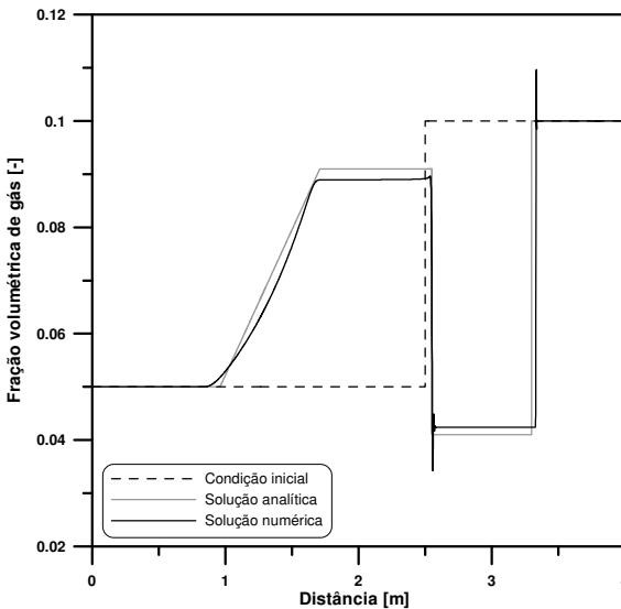
Figura 4.3 – Campos de fração volumétrica de gás em t = 15ms . Comparação da solução analítica com os resultados obtidos pelo modelo homogêneo de não-equilíbrio para C_T = 1 \times 10^9 W/m^3 K .
