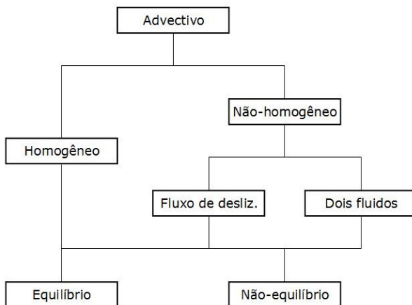
Figura 2.3 – Classificação dos modelos mecanicistas advectivos.
