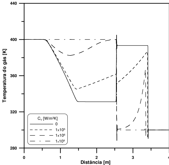
Figura 4.8 – Campos de temperatura do gás em t = 15ms . Comparação dos resultados obtidos pelo modelo homogêneo de não-equilíbrio para diferentes coeficientes de troca térmica.
