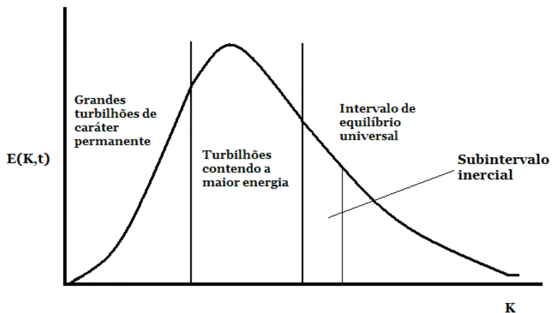
Figura 2.1 – Forma do espectro de energia para uma turbulência bem desenvolvida. Adaptada de Möller e Silvestrine, 2004.
